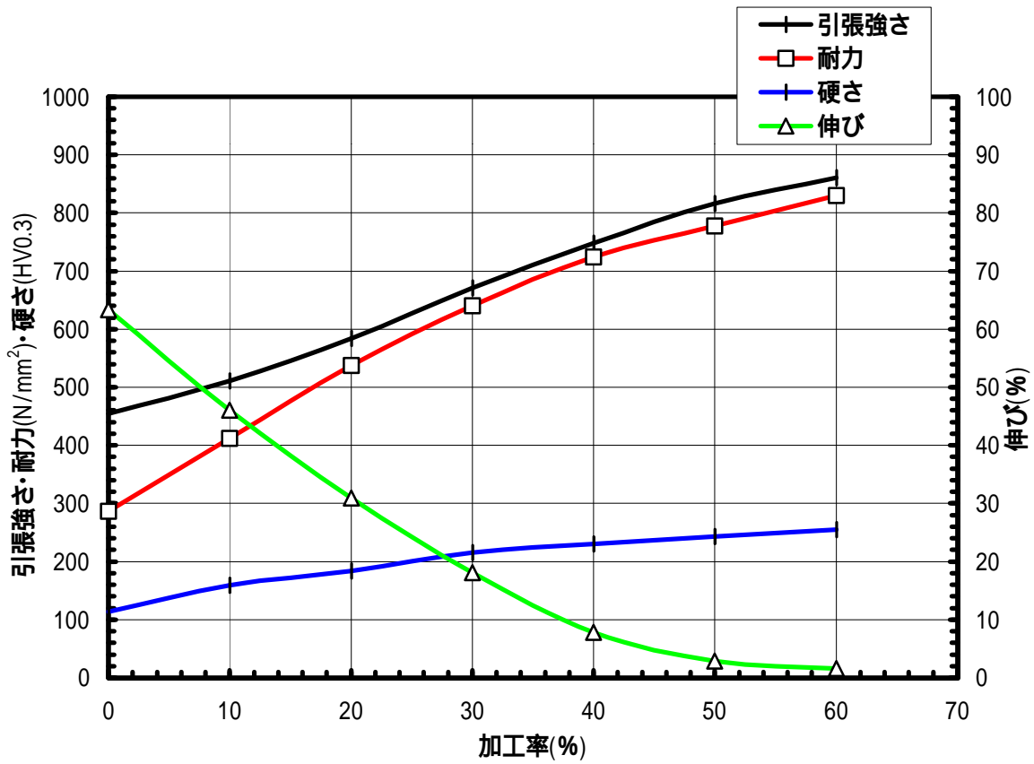
図 8.7 C5210の加工硬化特性(L.D.)
