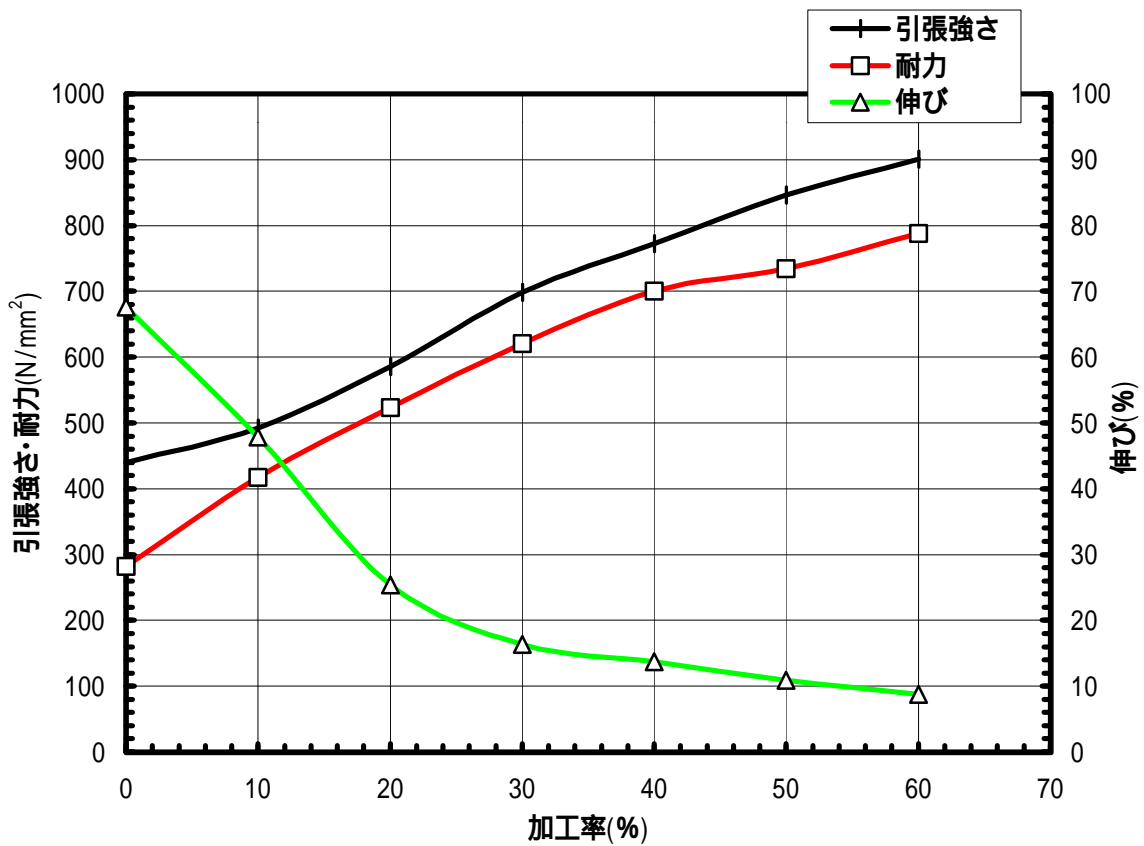
図 8.8 C5210の加工硬化特性(T.D.)
