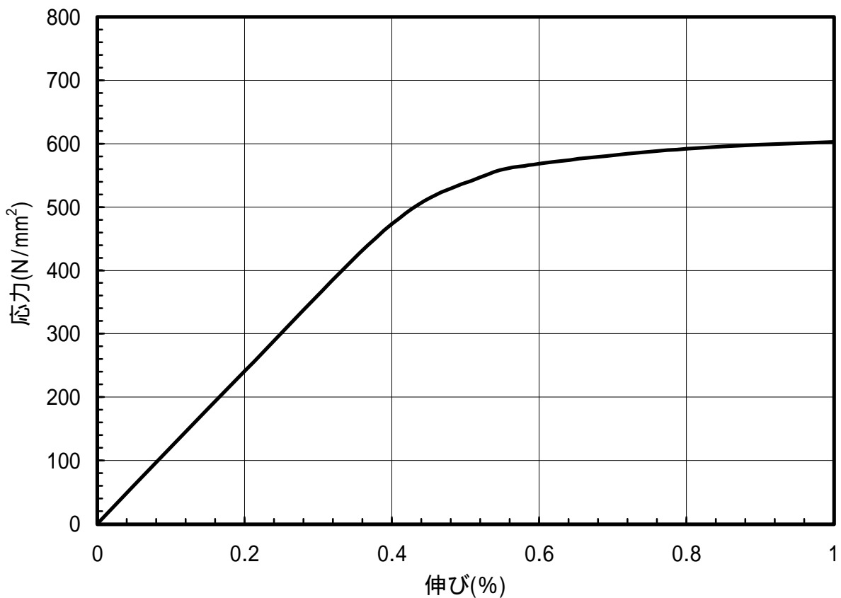
図 1.155 C7701-EH材のS-S曲線(45°)
