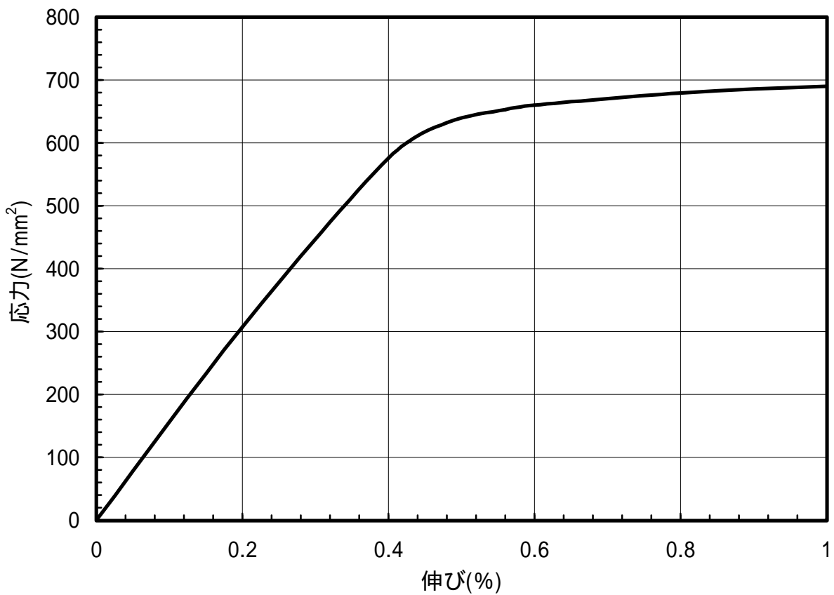
図 1.157 C7701-EH材のS-S曲線(T.D.)
