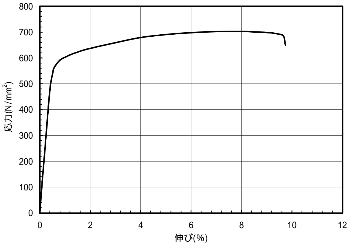
図 1.154 C7701-EH材のS-S曲線(45°)
