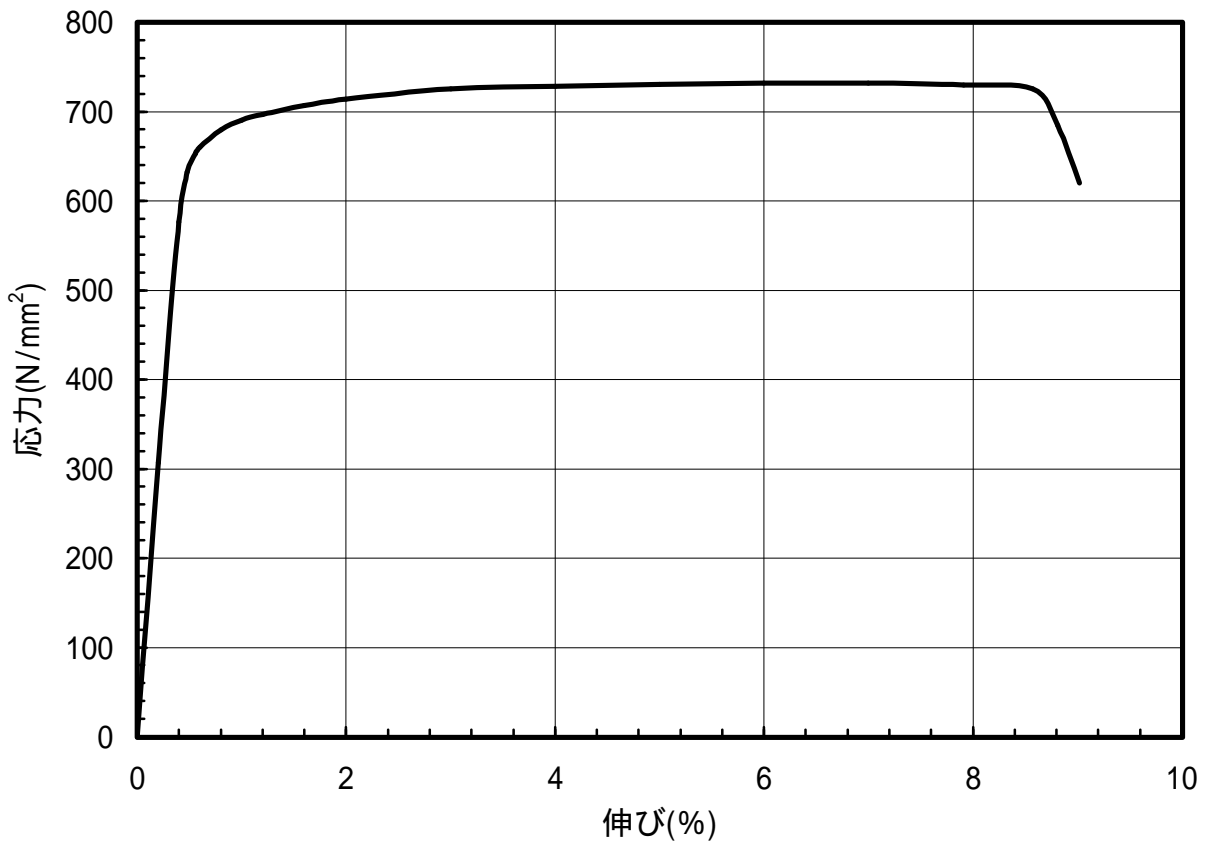
図 1.156 C7701-EH材のS-S曲線(T.D.)
