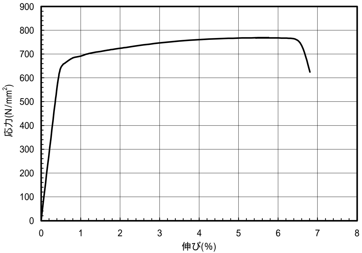
図 1.152 C7701-EH材のS-S曲線(L.D.)
