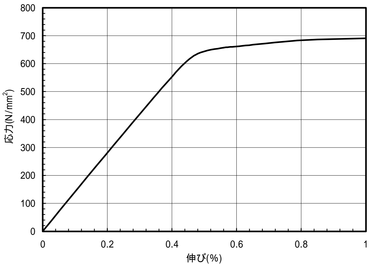
図 1.153 C7701-EH材のS-S曲線(L.D.)
