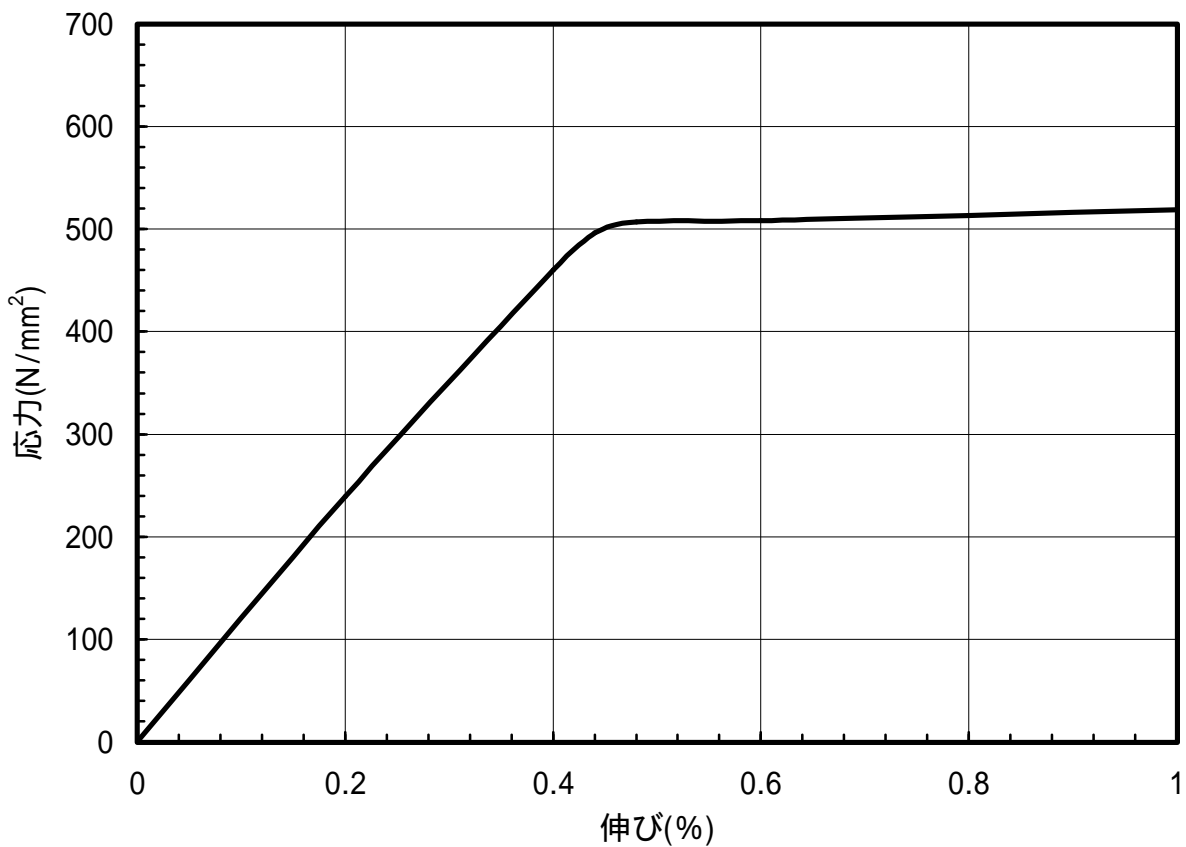
図 1.149 C7701-H材のS-S曲線(45 °)
