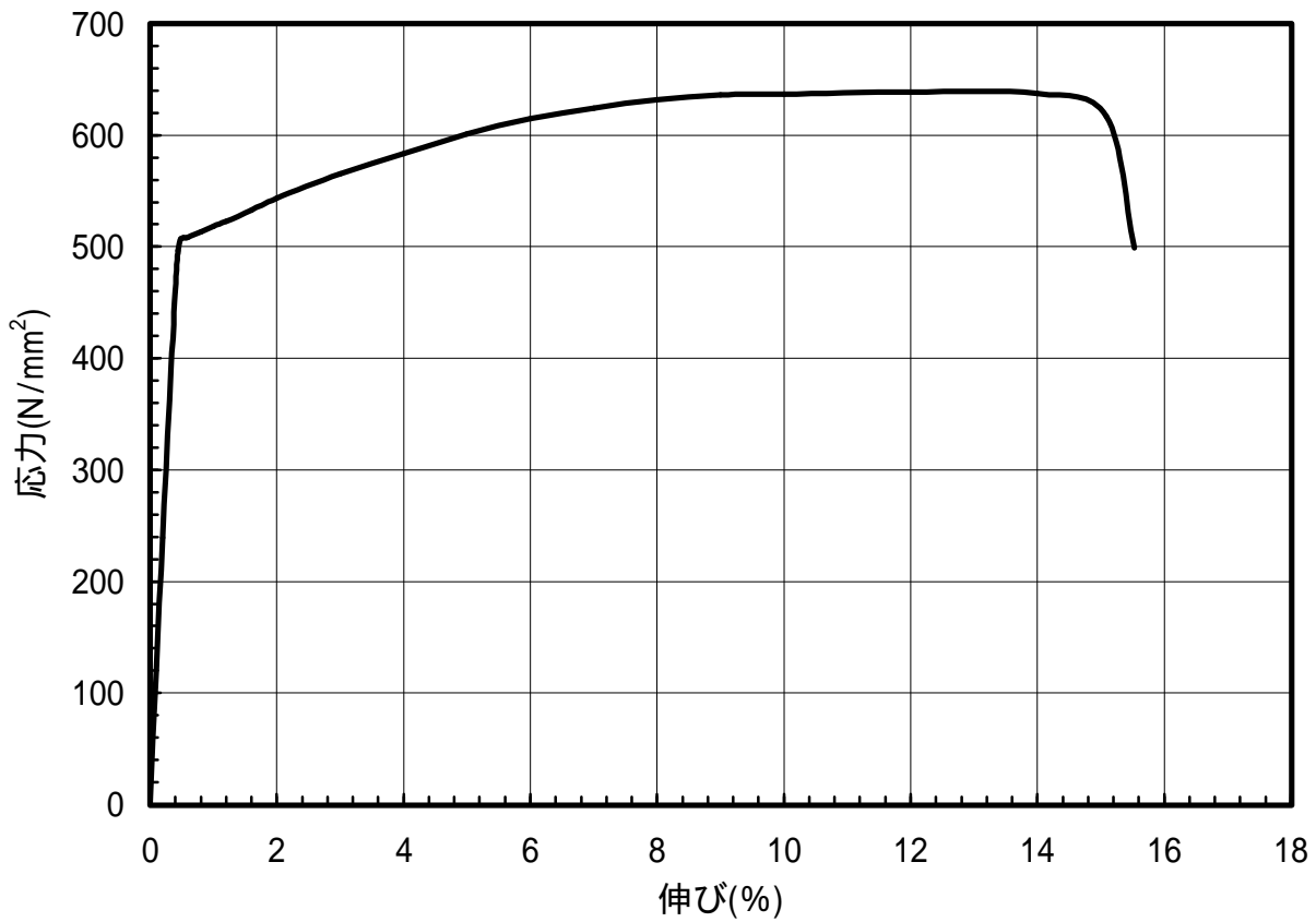
図 1.148 C7701-H材のS-S曲線(45 °)
