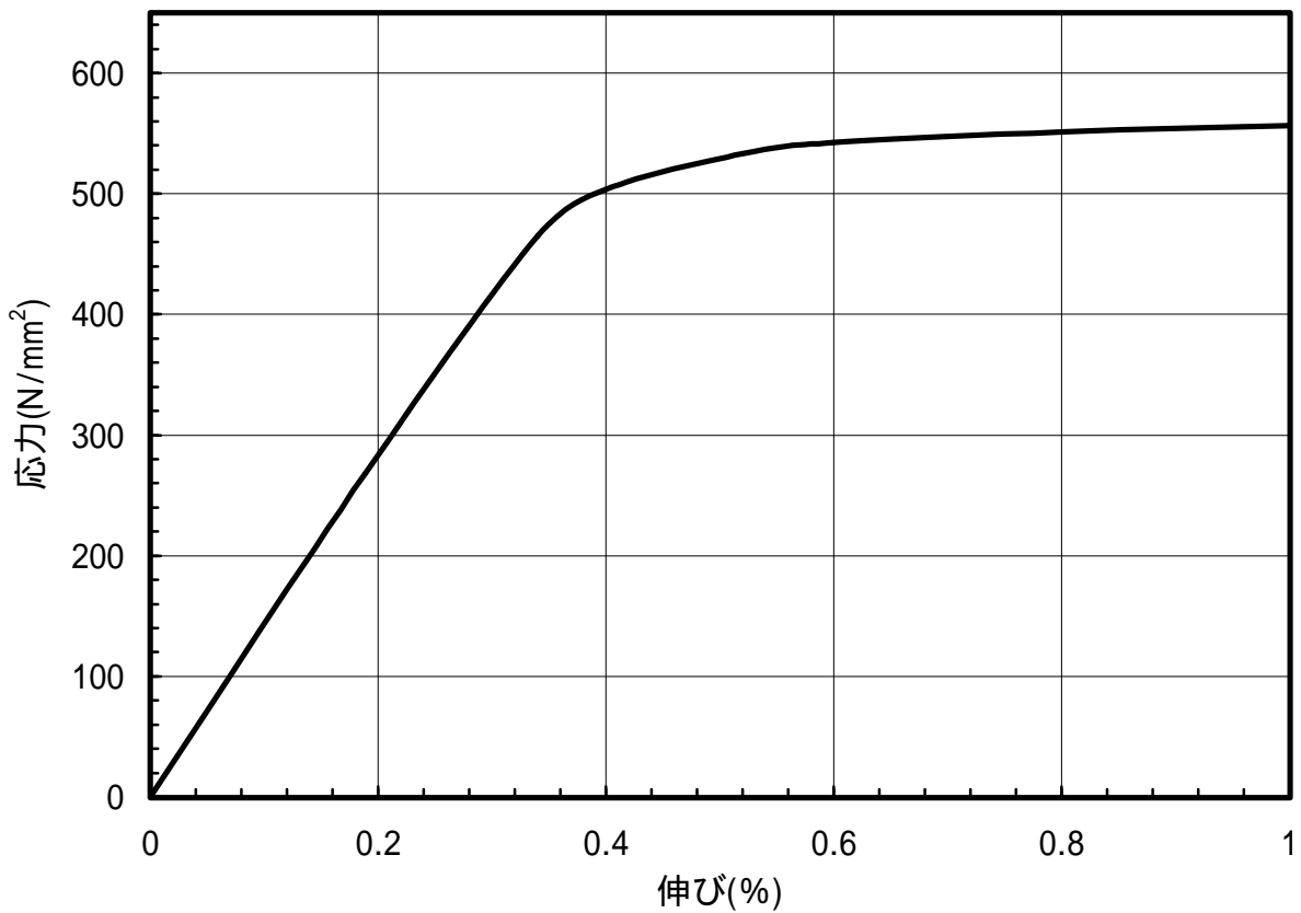
図 1.147 C7701-H材のS-S曲線(L.D.)
