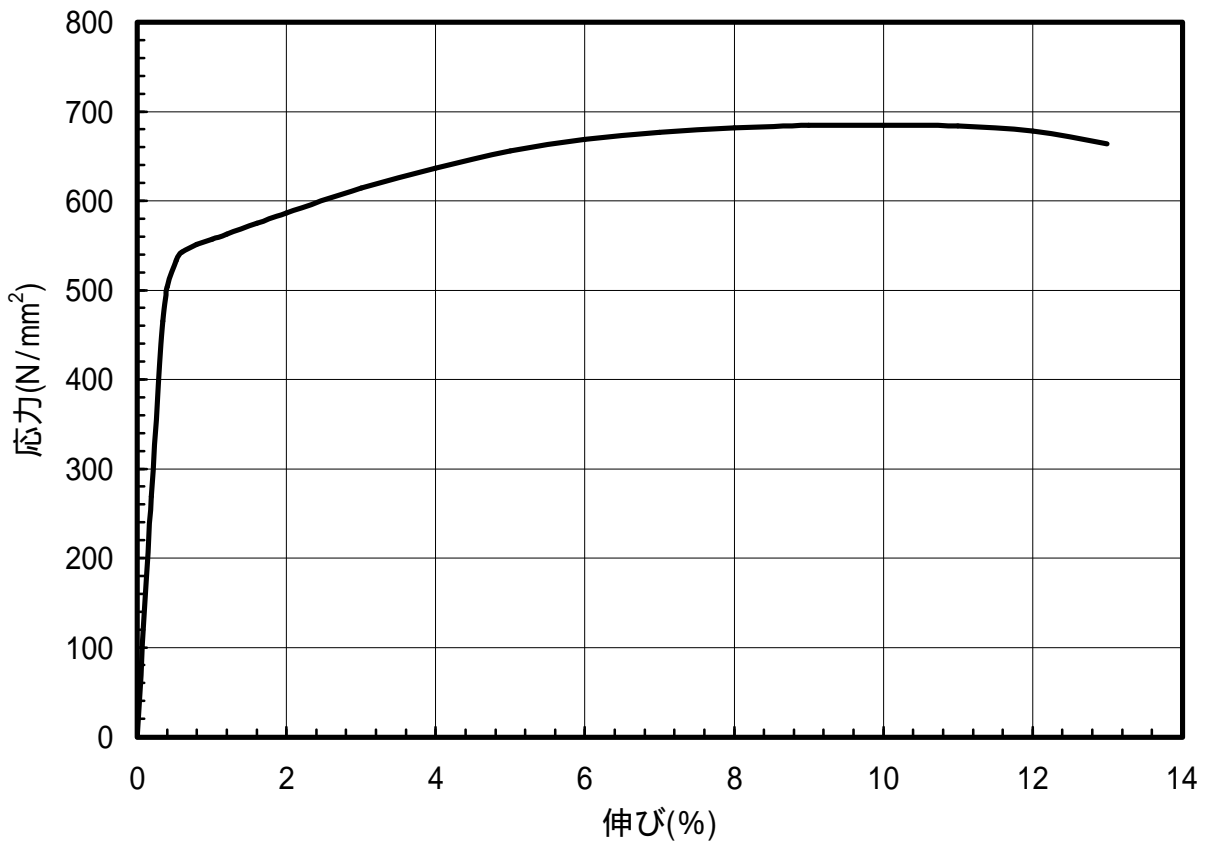
図 1.146 C7701-H材のS-S曲線(L.D.)
