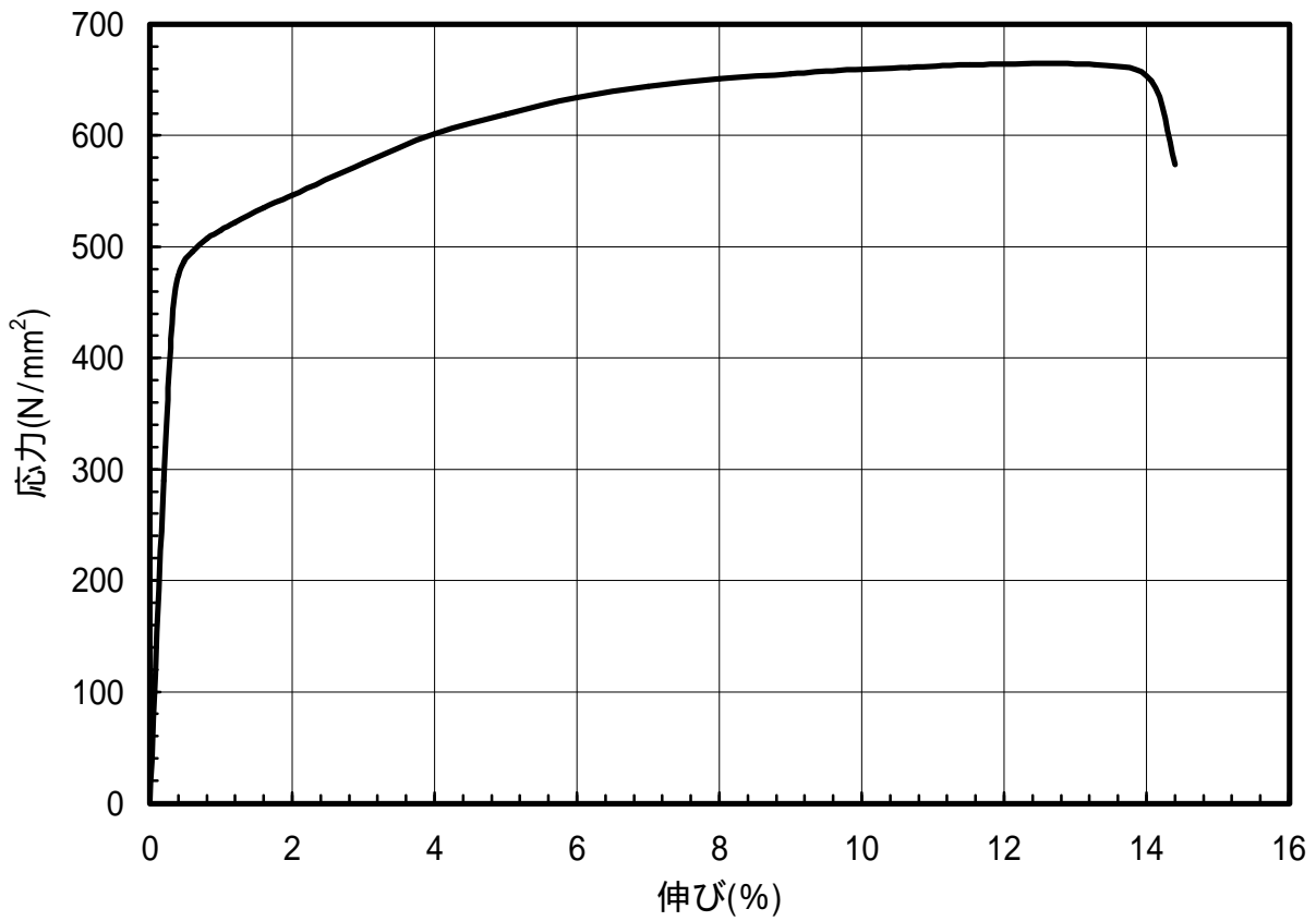
図 1.50 C7701-H材のS-S曲線(T.D.)
