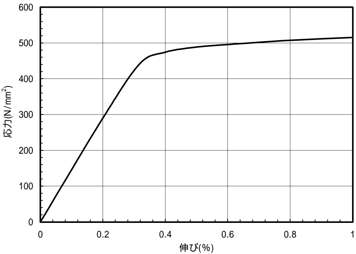
図 1.151 C7701-H材のS-S曲線(T.D.)
