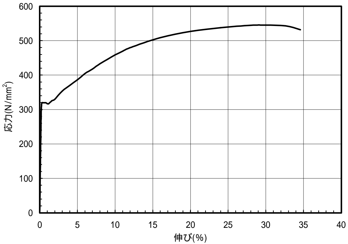
図 1.144 C7701-1/2H材のS-S曲線(T.D.)
