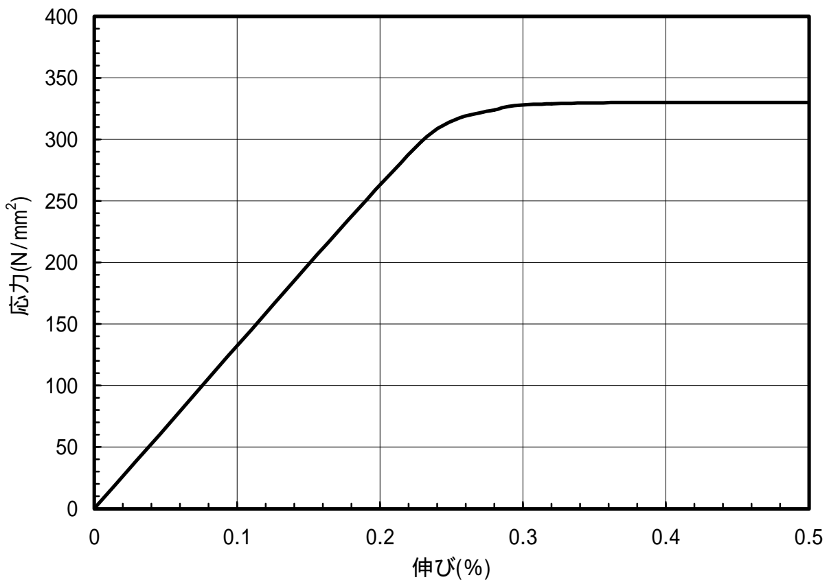
図 1.141 C7701-1/2H材のS-S曲線(L.D.)
