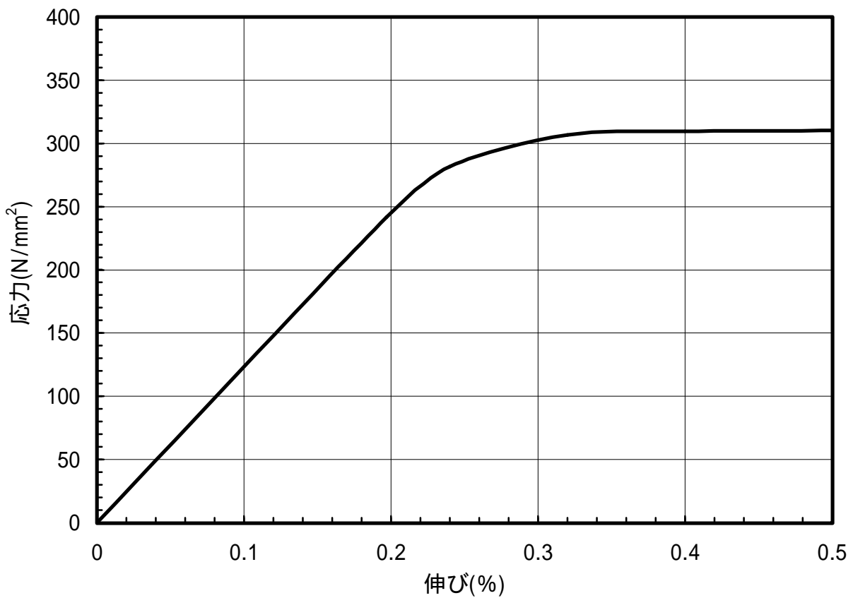
図 1.143 C7701-1/2H材のS-S曲線(45°)
