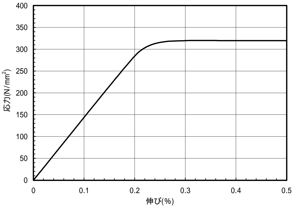
図 1.145 C7701-1/2H材のS-S曲線(T.D.)
