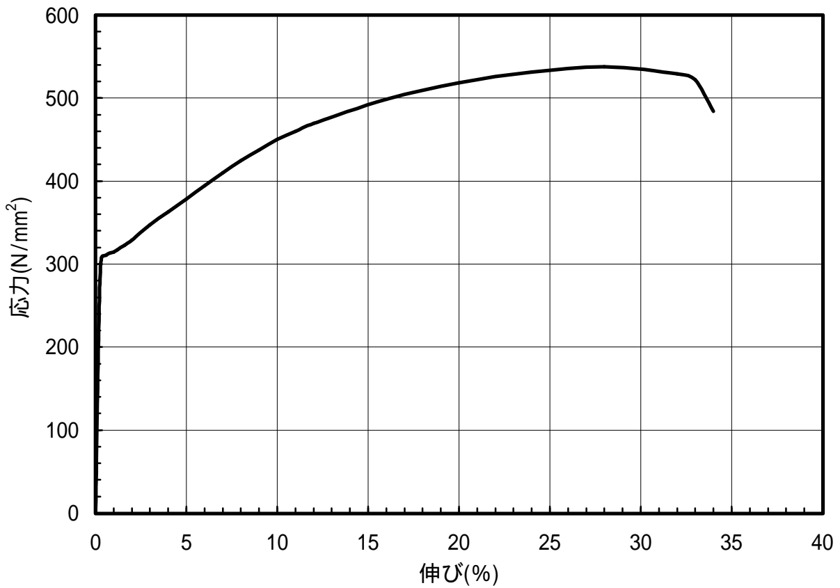
図 1.142 C7701-1/2H材のS-S曲線(45°)
