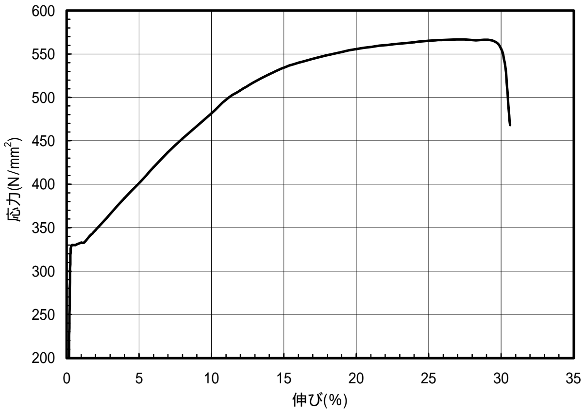
図 1.140 C7701-1/2H材のS-S曲線(L.D.)
