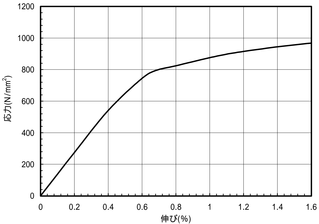
図 1.137 C1990-EHM材のS-S曲線(45 °)
