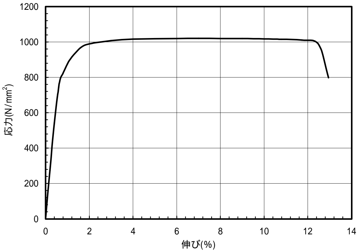
図 1.136 C1990-EHM材のS-S曲線(45 °)
