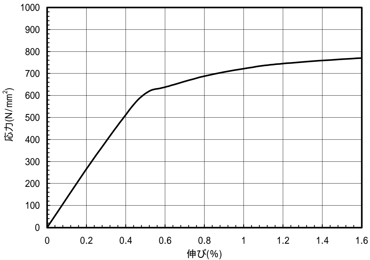
図 1.131 C1990-1/4HM材のS-S曲線(45 °)
