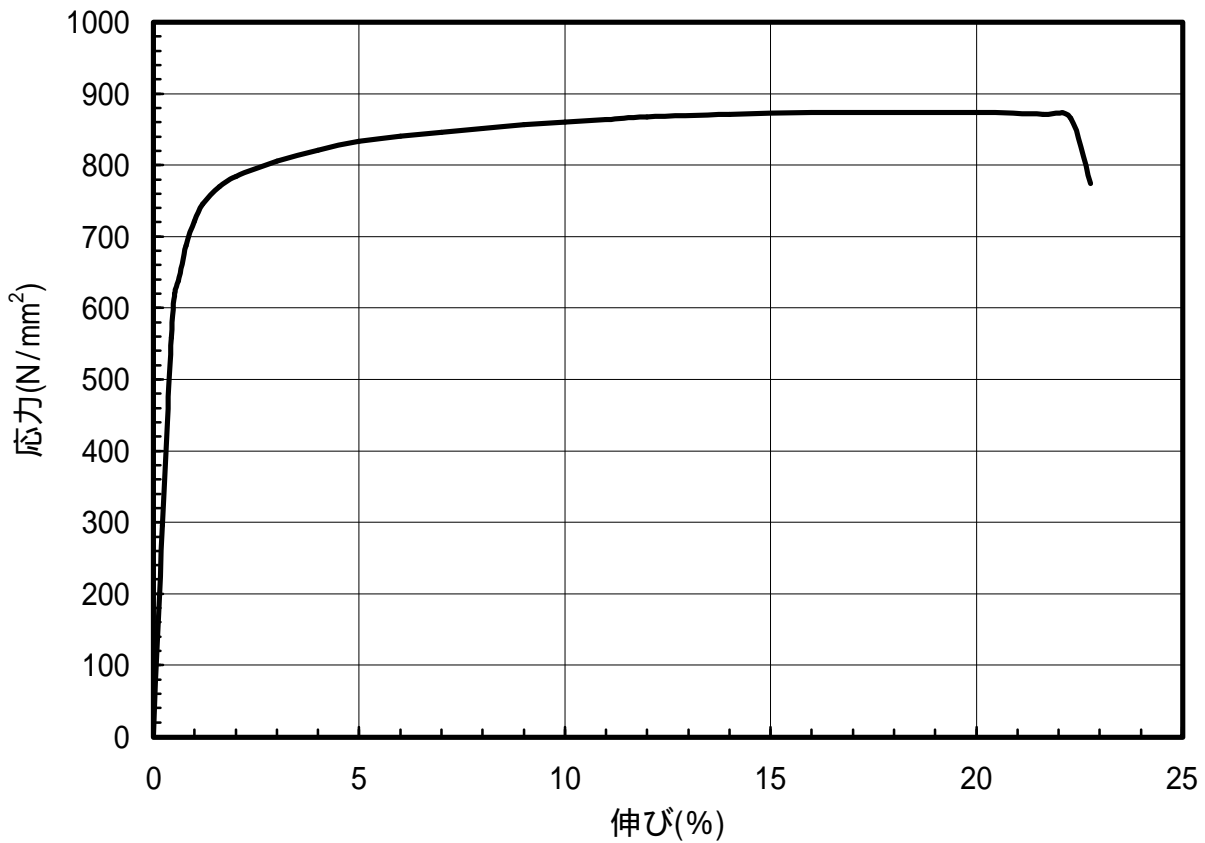
図 1.130 C1990-1/4HM材のS-S曲線(45 °)
