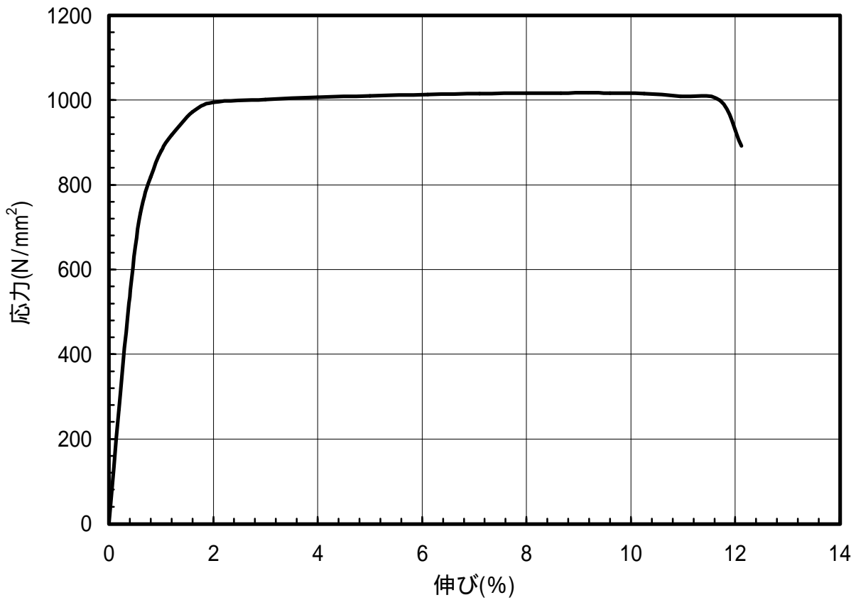
図 1.126 C1720-HM材のS-S曲線(T.D.)
