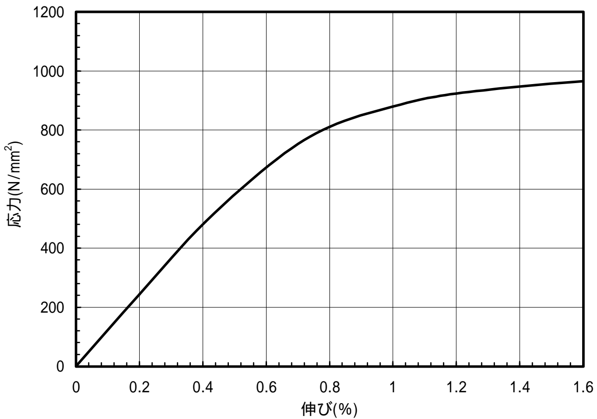
図 1.123 C1720-HM材のS-S曲線(L.D.)
