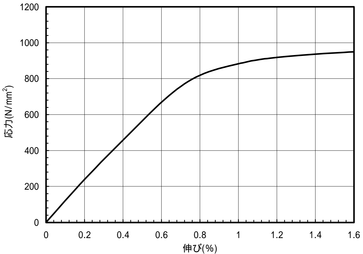
図 1.125 C1720-HM材のS-S曲線(45°)
