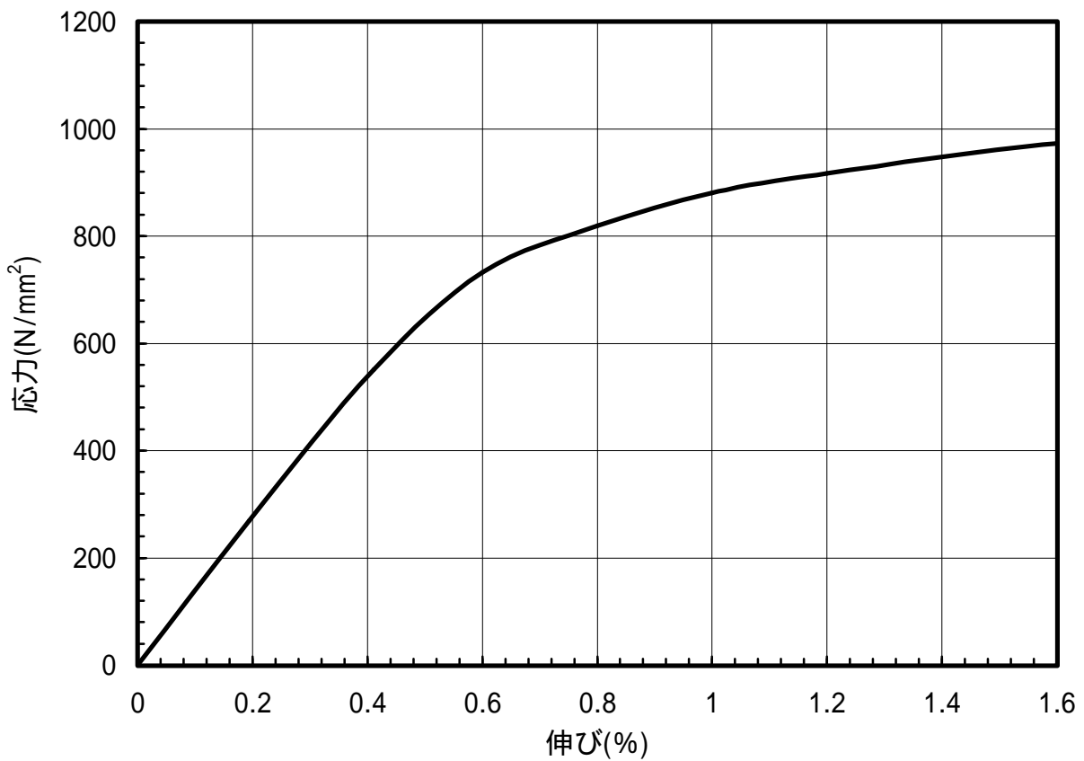
図 1.127 C1720-HM材のS-S曲線(T.D.)
