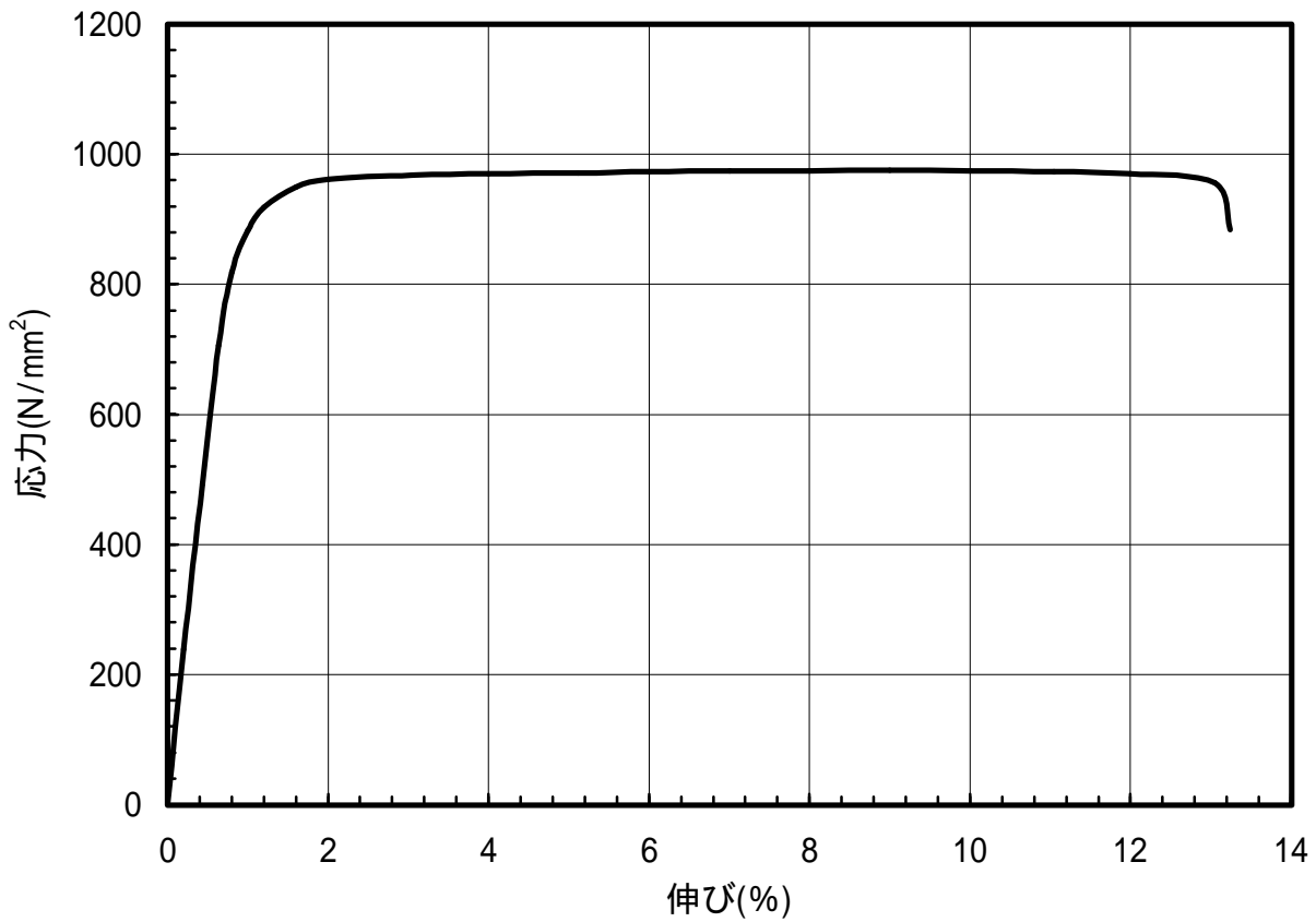
図 1.124 C1720-HM材のS-S曲線(45°)
