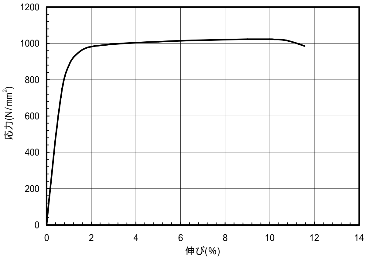
図 1.122 C1720-HM材のS-S曲線(L.D.)
