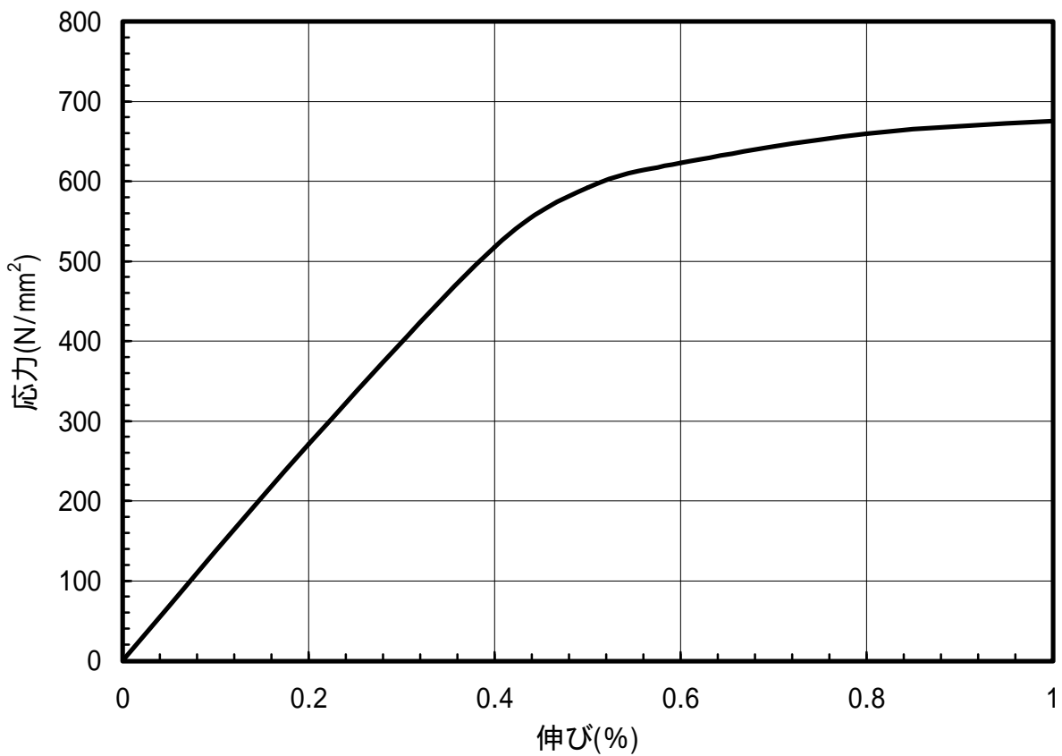
図 1.117 C1720-1/4HM材のS-S曲線(L.D.)
