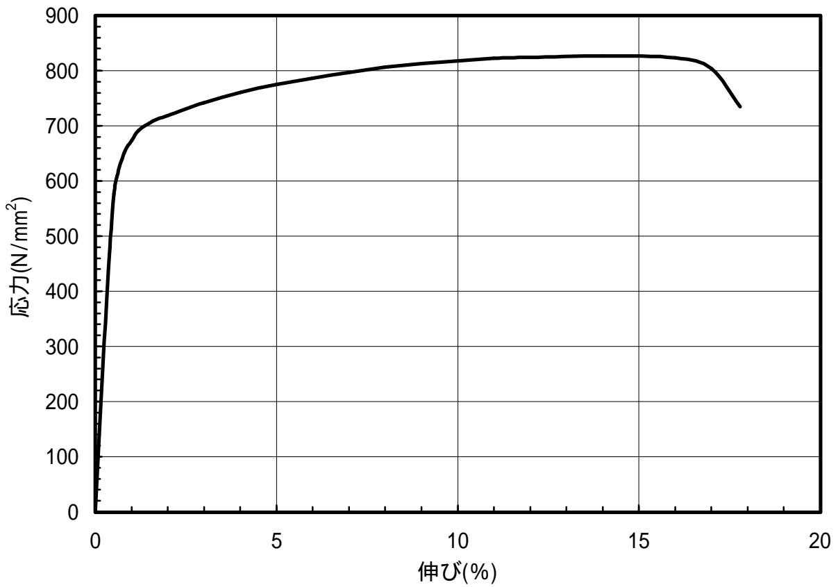
図 1.118 C1720-1/4HM材のS-S曲線(45 °)
