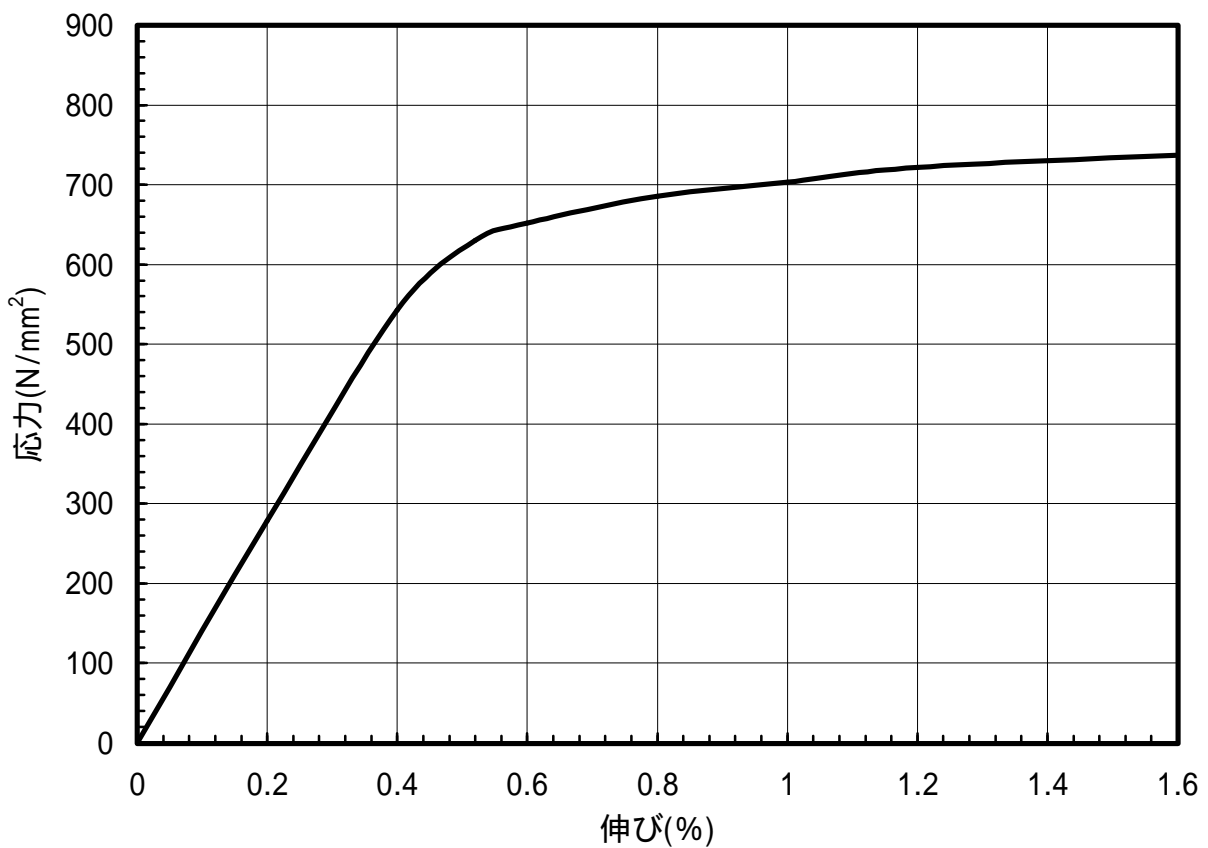
図 1.121 C1720-1/4HM材のS-S曲線(T.D.)
