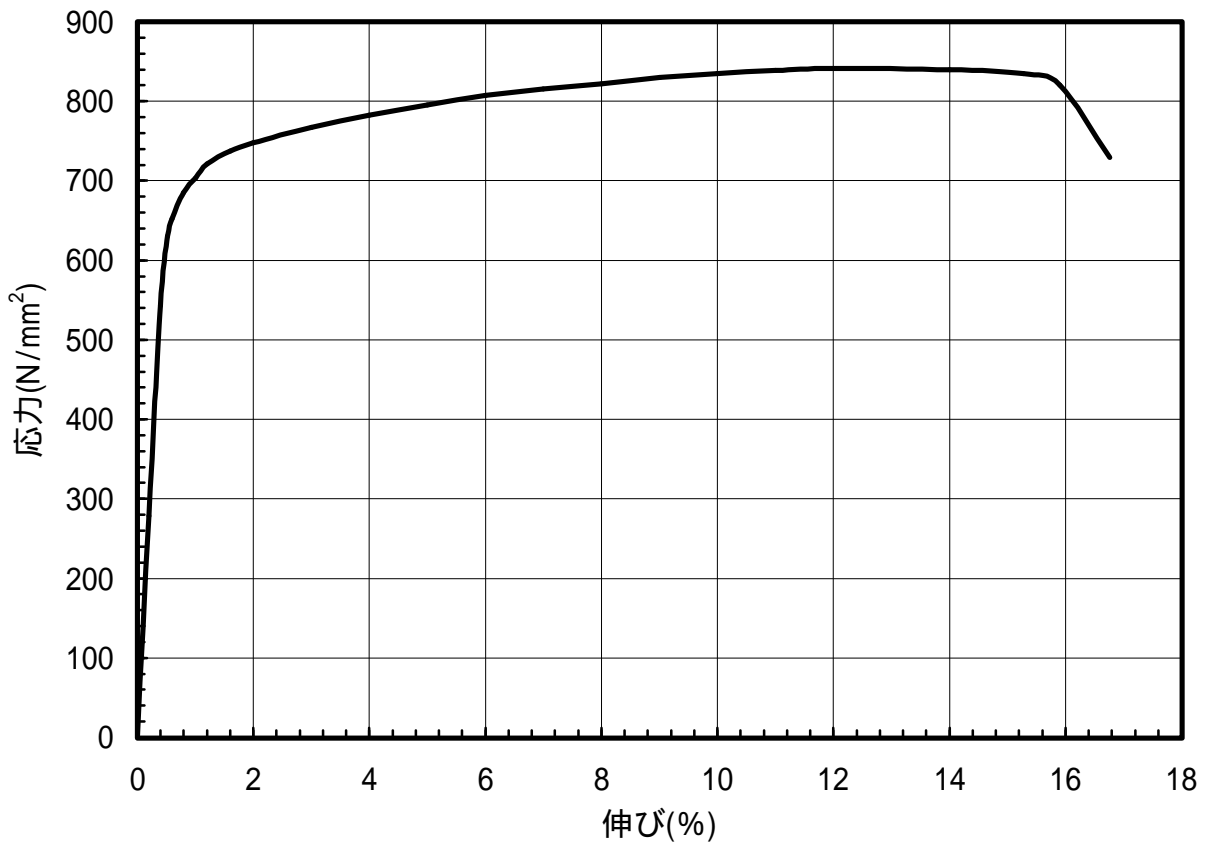
図 1.120 C1720-1/4HM材のS-S曲線(T.D.)
