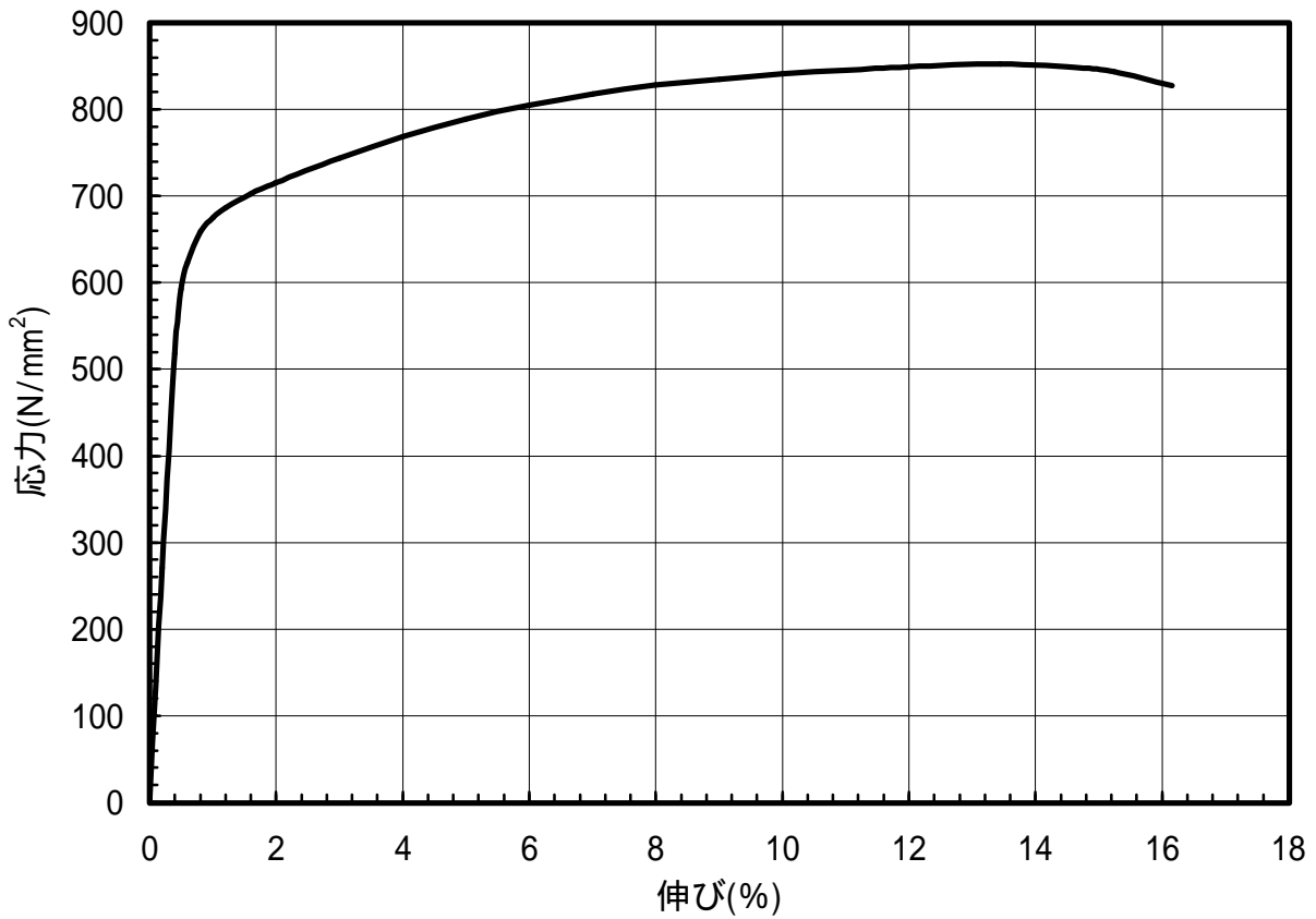
図 1.116 C1720-1/4HM材のS-S曲線(L.D.)
