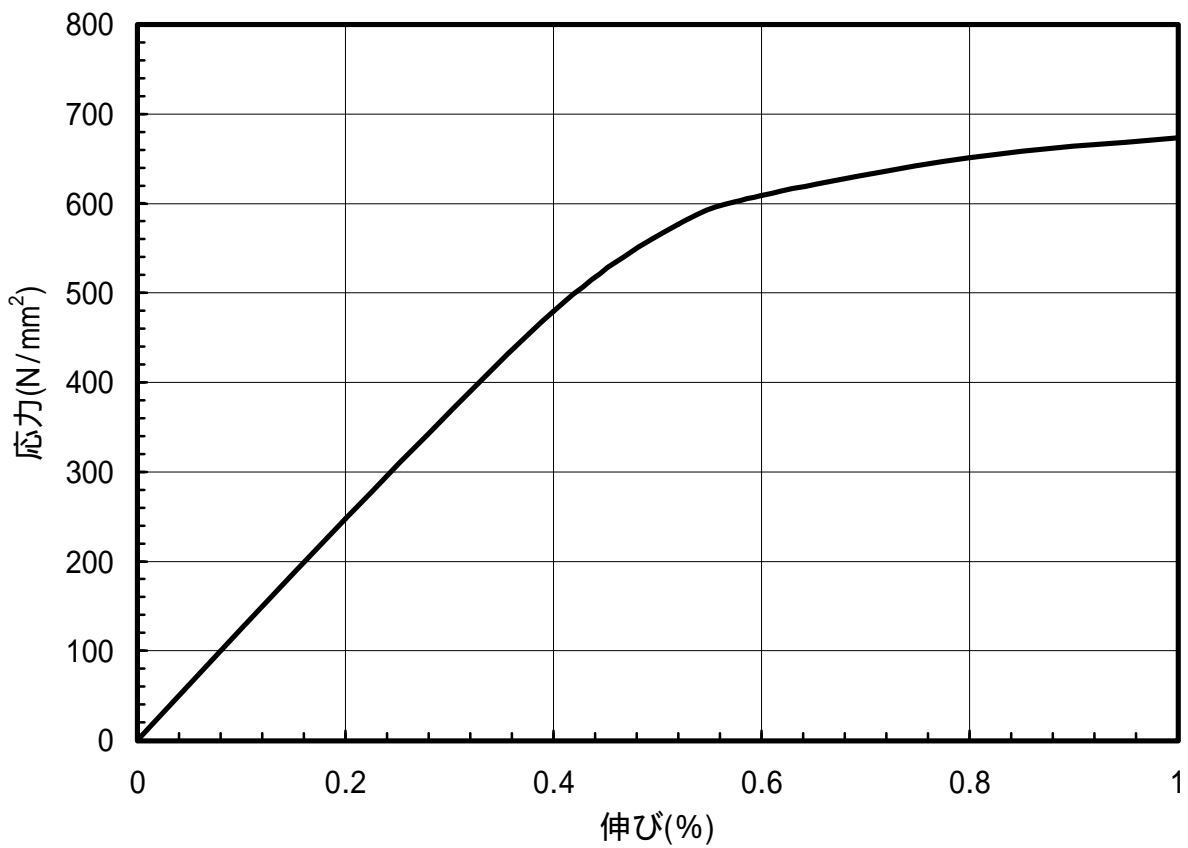
図 1.119 C1720-1/4HM材のS-S曲線(45 °)
