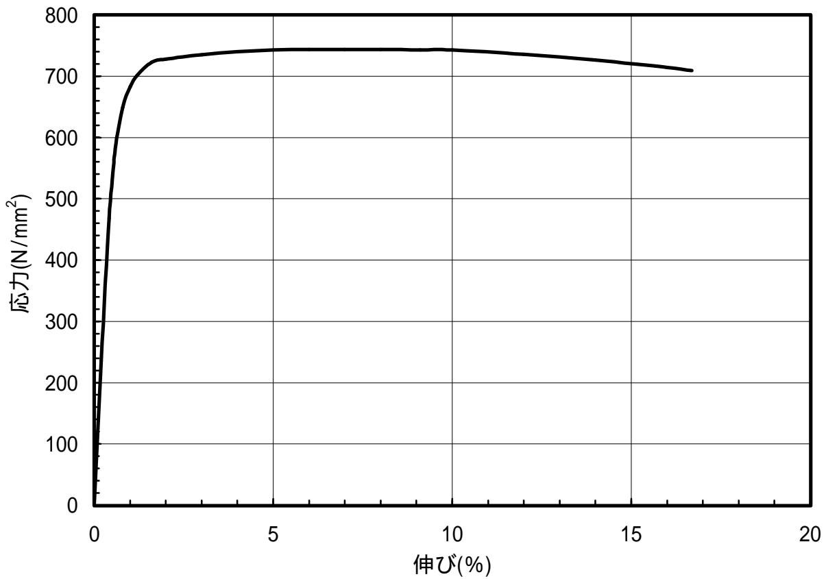
図 1.114 C5210-EH材のS-S曲線(T.D.)
