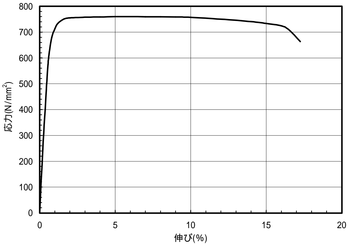
図 1.112 C5210-EH材のS-S曲線(45°)
