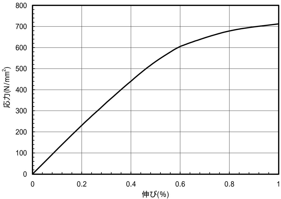
図 1.113 C5210-EH材のS-S曲線(45°)
