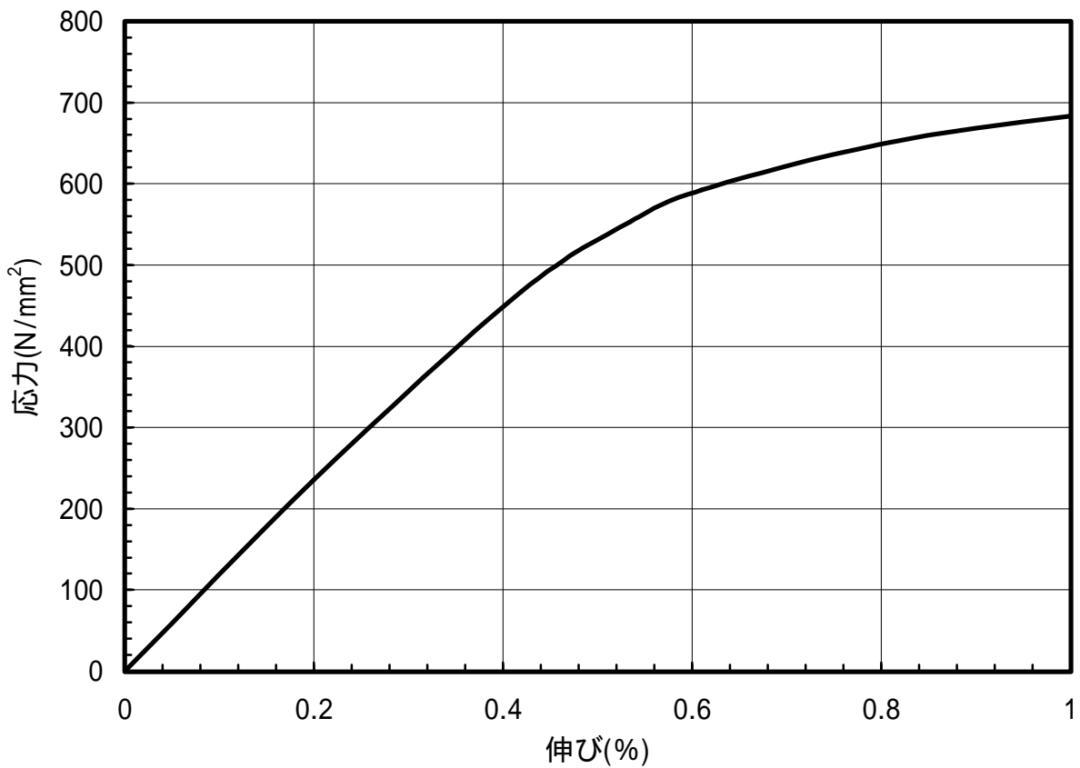
図 1.115 C5210-EH材のS-S曲線(T.D.)
