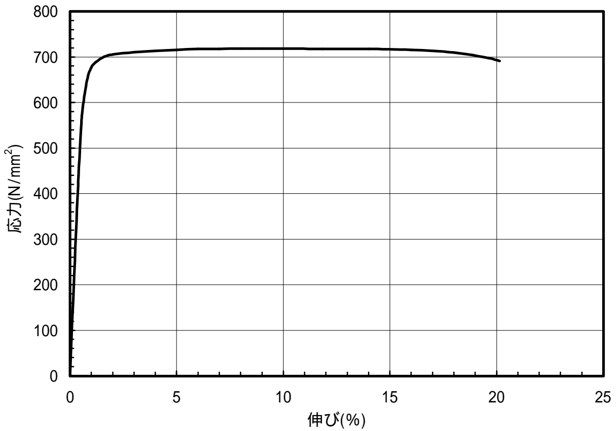
図 1.110 C5210-EH材のS-S曲線(L.D.)
