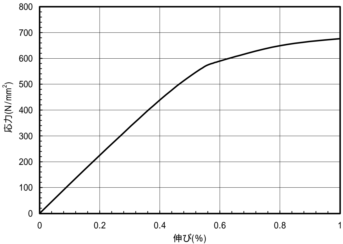
図 1.111 C5210-EH材のS-S曲線(L.D.)
