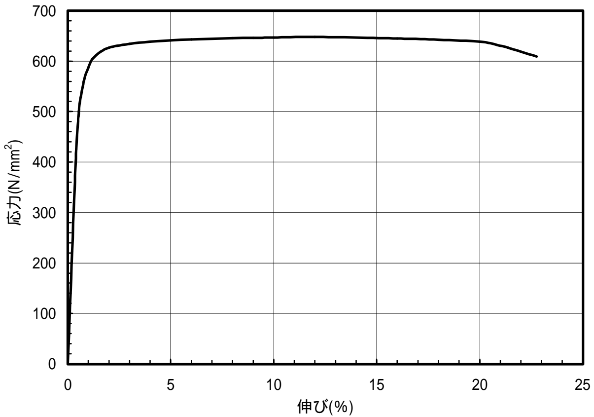
図 1.106 C5210-H材のS-S曲線(45 °)
