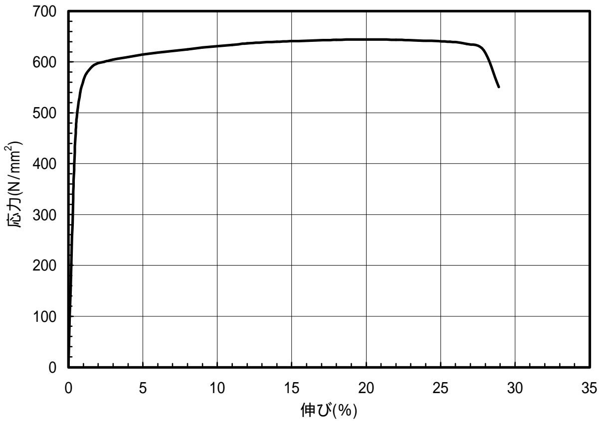
図 1.104 C5210-H材のS-S曲線(L.D.)
