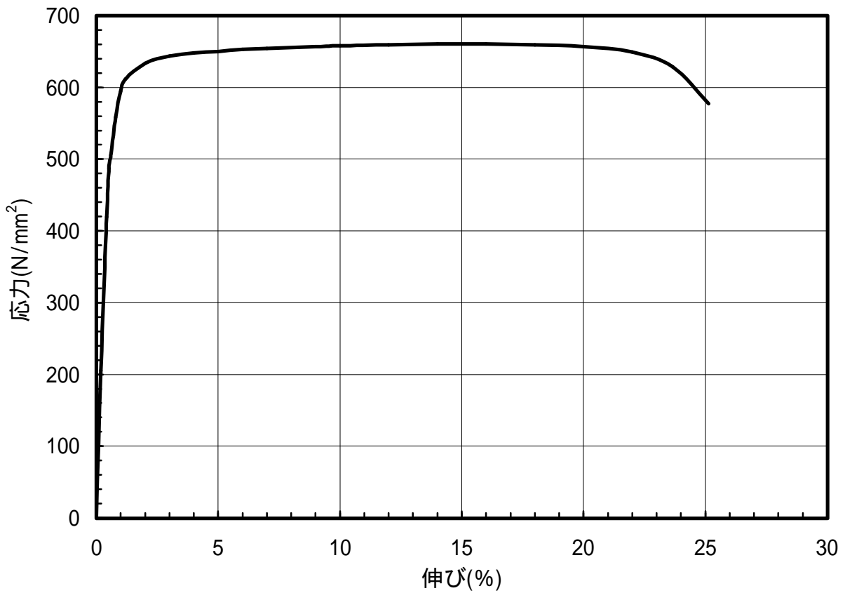
図 1.108 C5210-H材のS-S曲線(T.D.)
