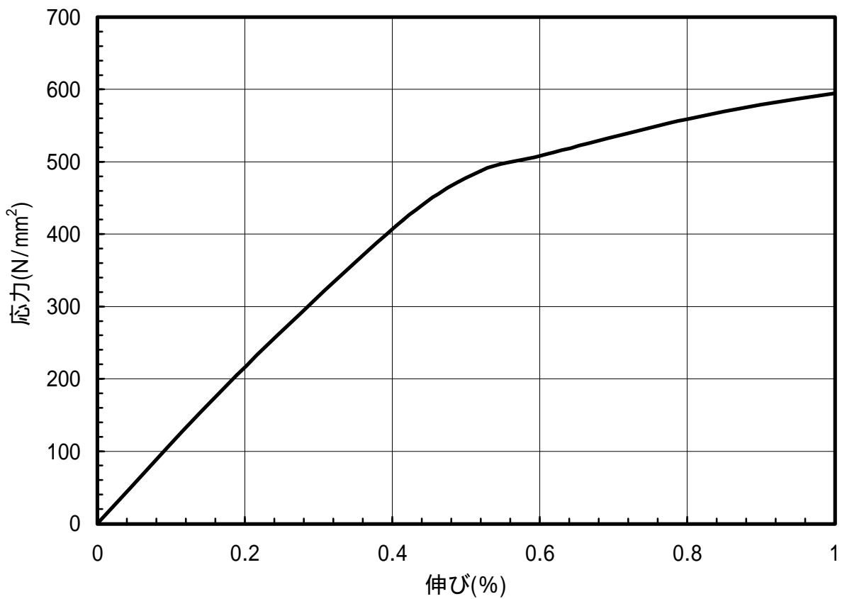
図 1.109 C5210-H材のS-S曲線(T.D.)
