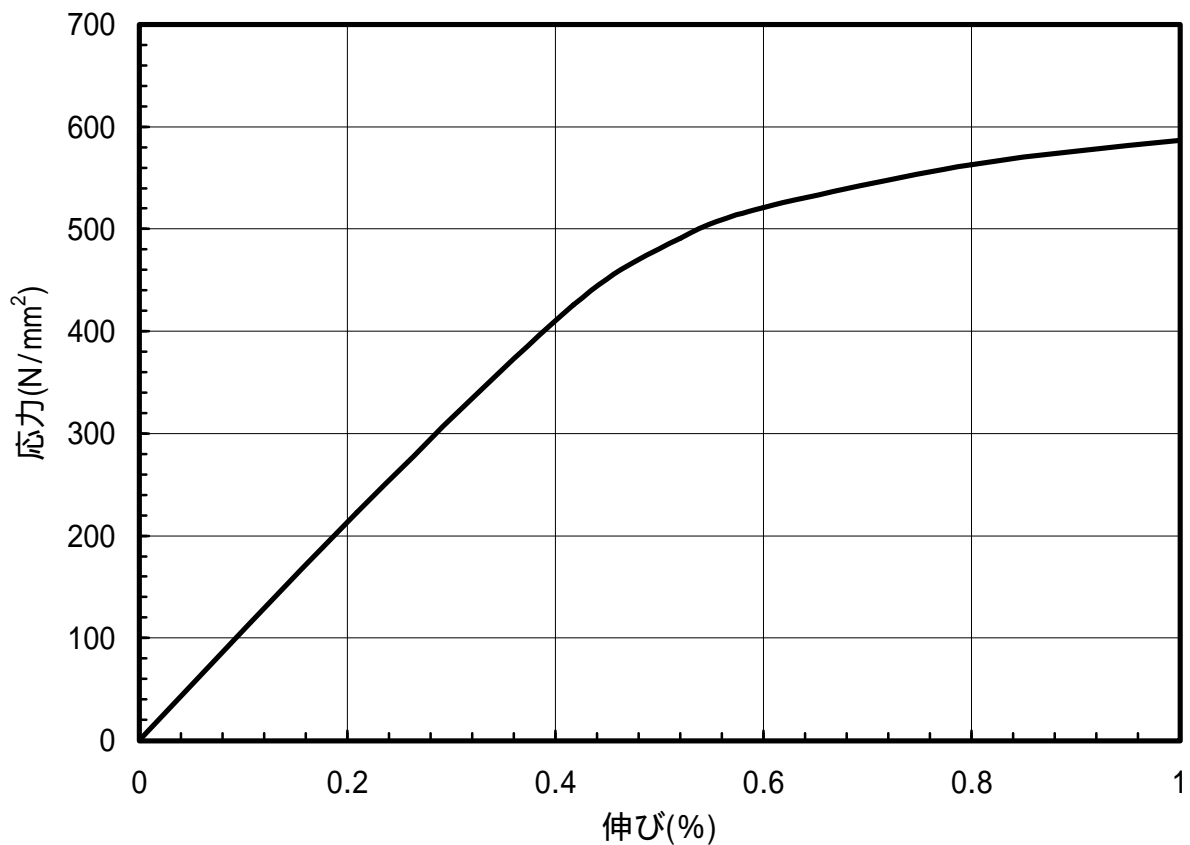
図 1.107 C5210-H材のS-S曲線(T.D.)
