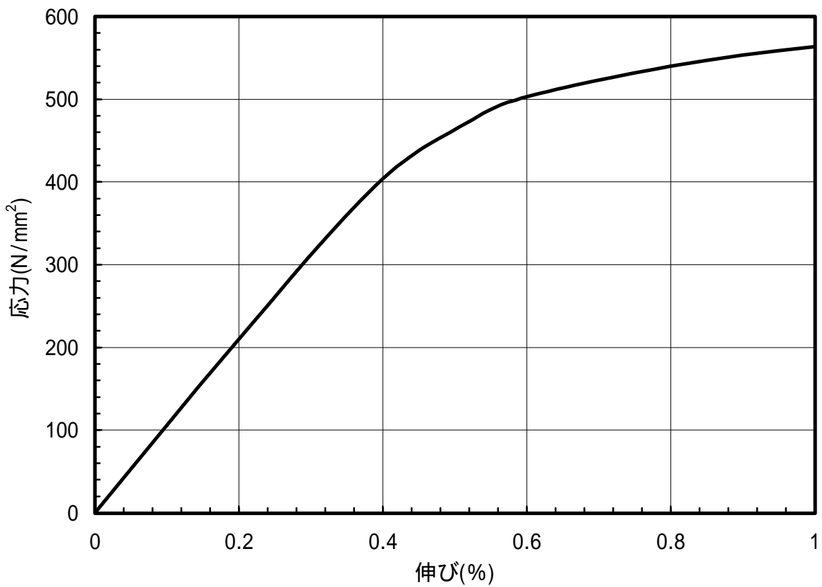
図 1.105 C5210-H材のS-S曲線(L.D.)
