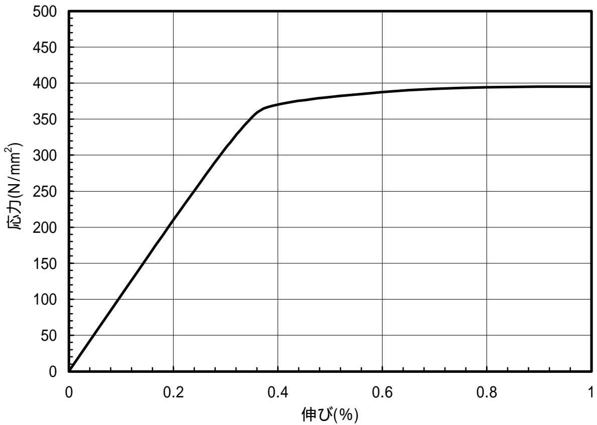
図 1.101 C5210-1/2H材のS-S曲線(45 °)
