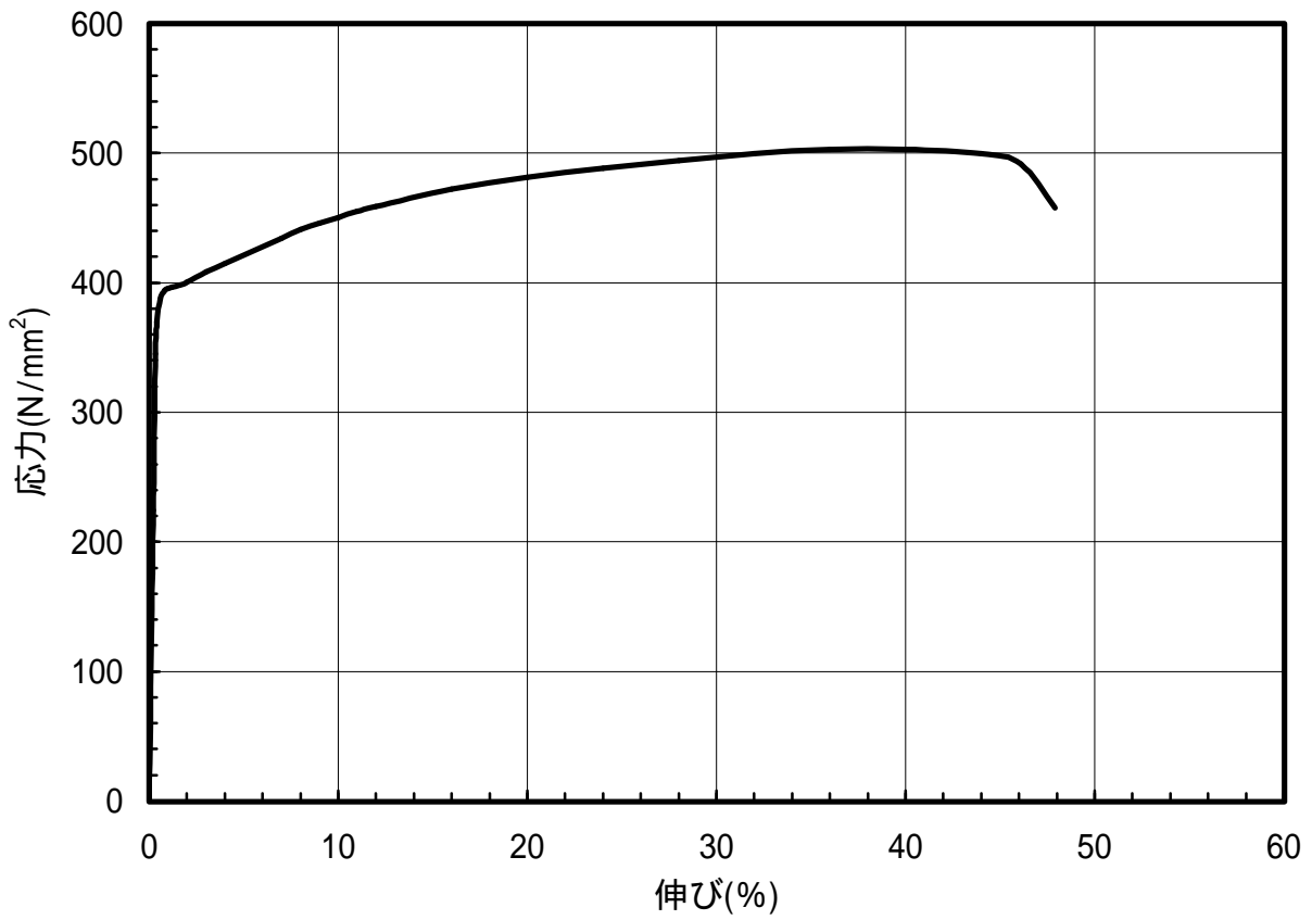
図 1.100 C5210-1/2H材のS-S曲線(45 °)
