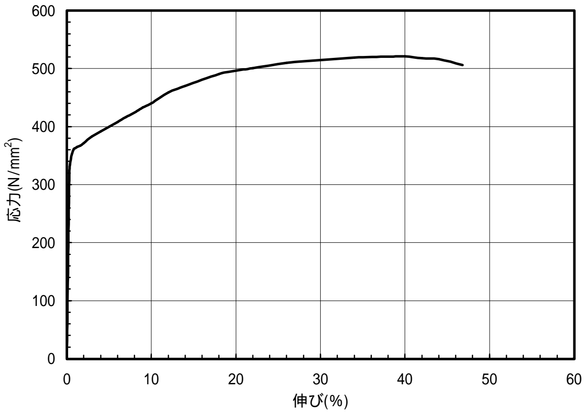
図 1.98 C5210-1/2H材のS-S曲線(L.D.)
