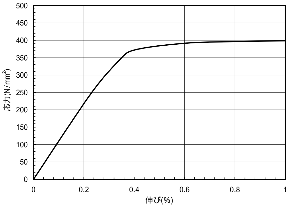
図 1.103 C5210-1/2H材のS-S曲線(T.D.)
