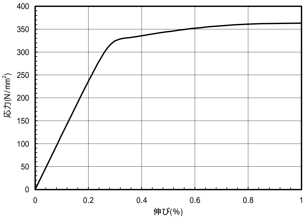
図 1.99 C5210-1/2H材のS-S曲線(L.D.)
