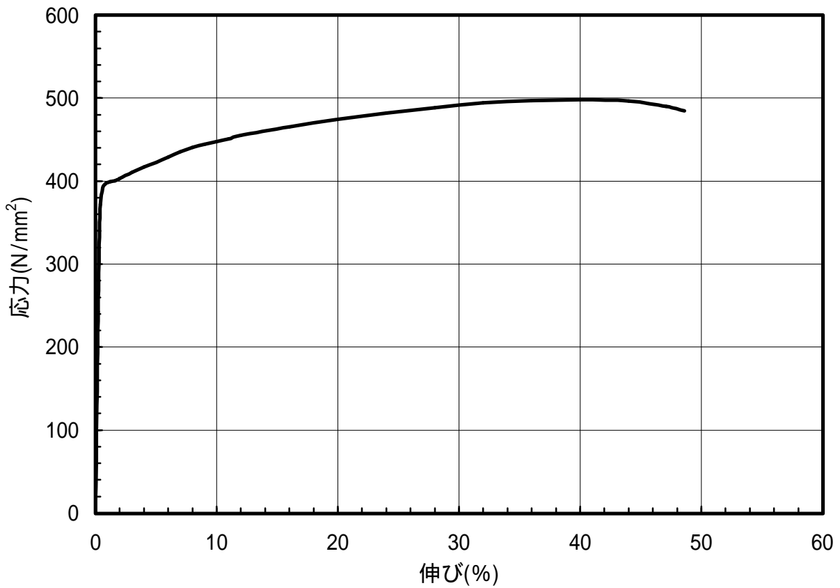
図 1.102 C5210-1/2H材のS-S曲線(T.D.)
