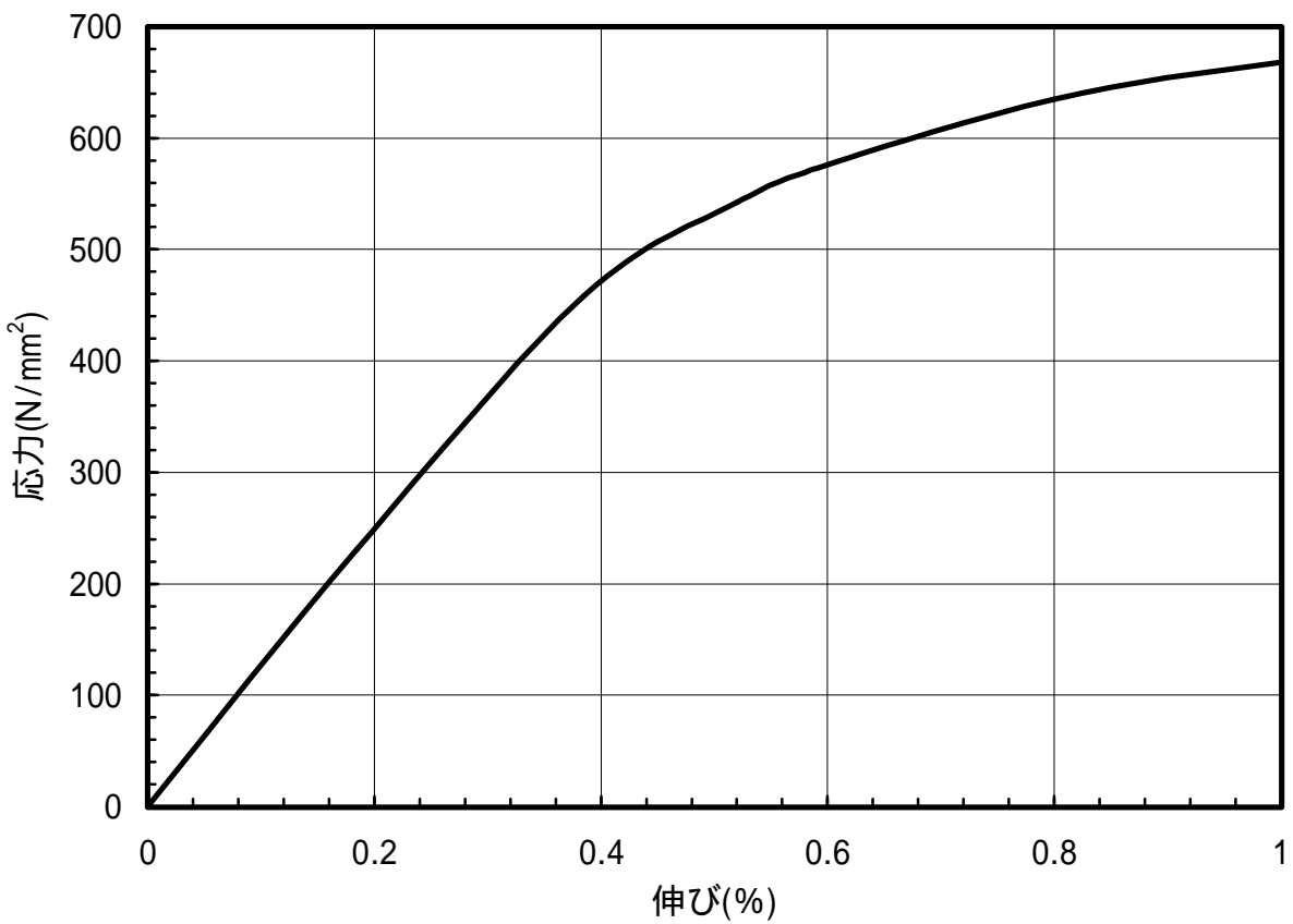
図 1.97 C5191-EH材のS-S曲線(T.D.)
