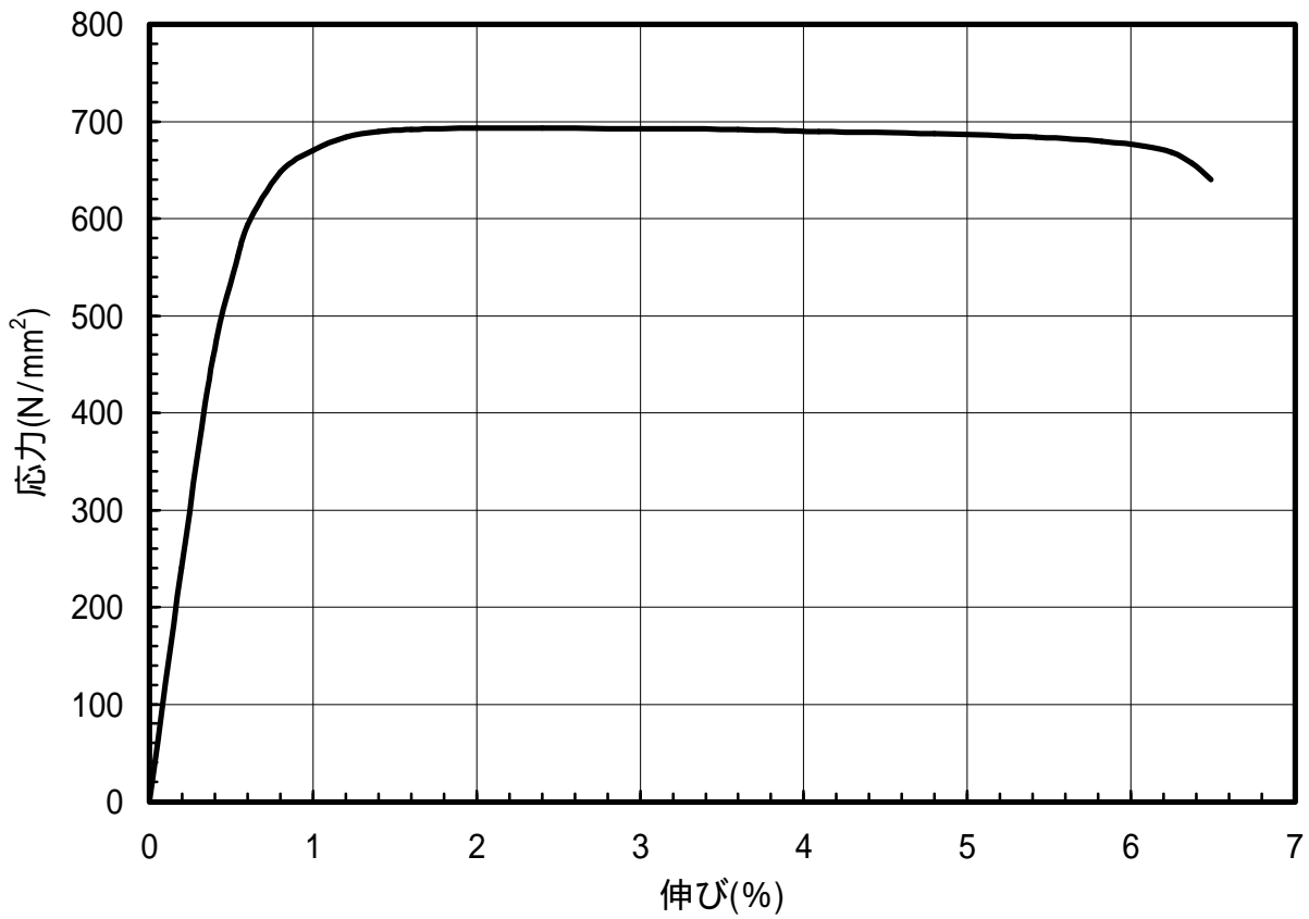
図 1.92 C5191-EH材のS-S曲線(L.D.)
