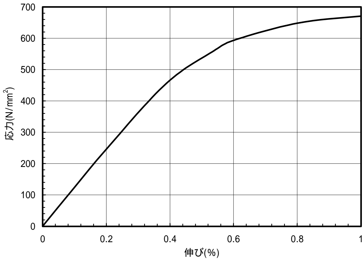
図 1.93 C5191-EH材のS-S曲線(L.D.)
