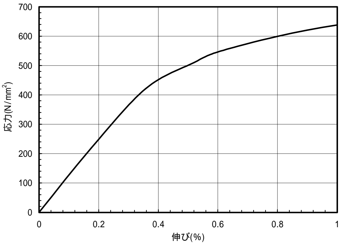
図 1.95 C5191-EH材のS-S曲線(45°)
