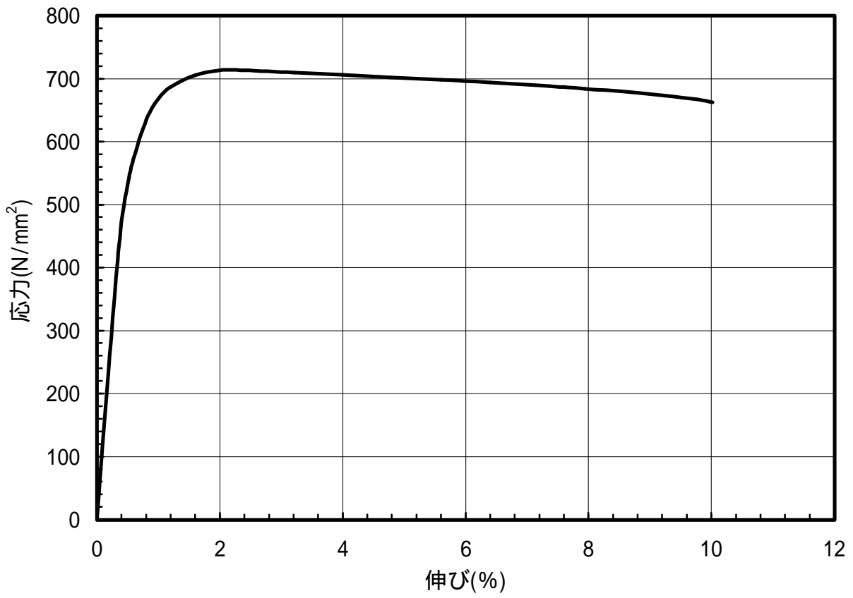
図 1.96 C5191-EH材のS-S曲線(T.D.)
