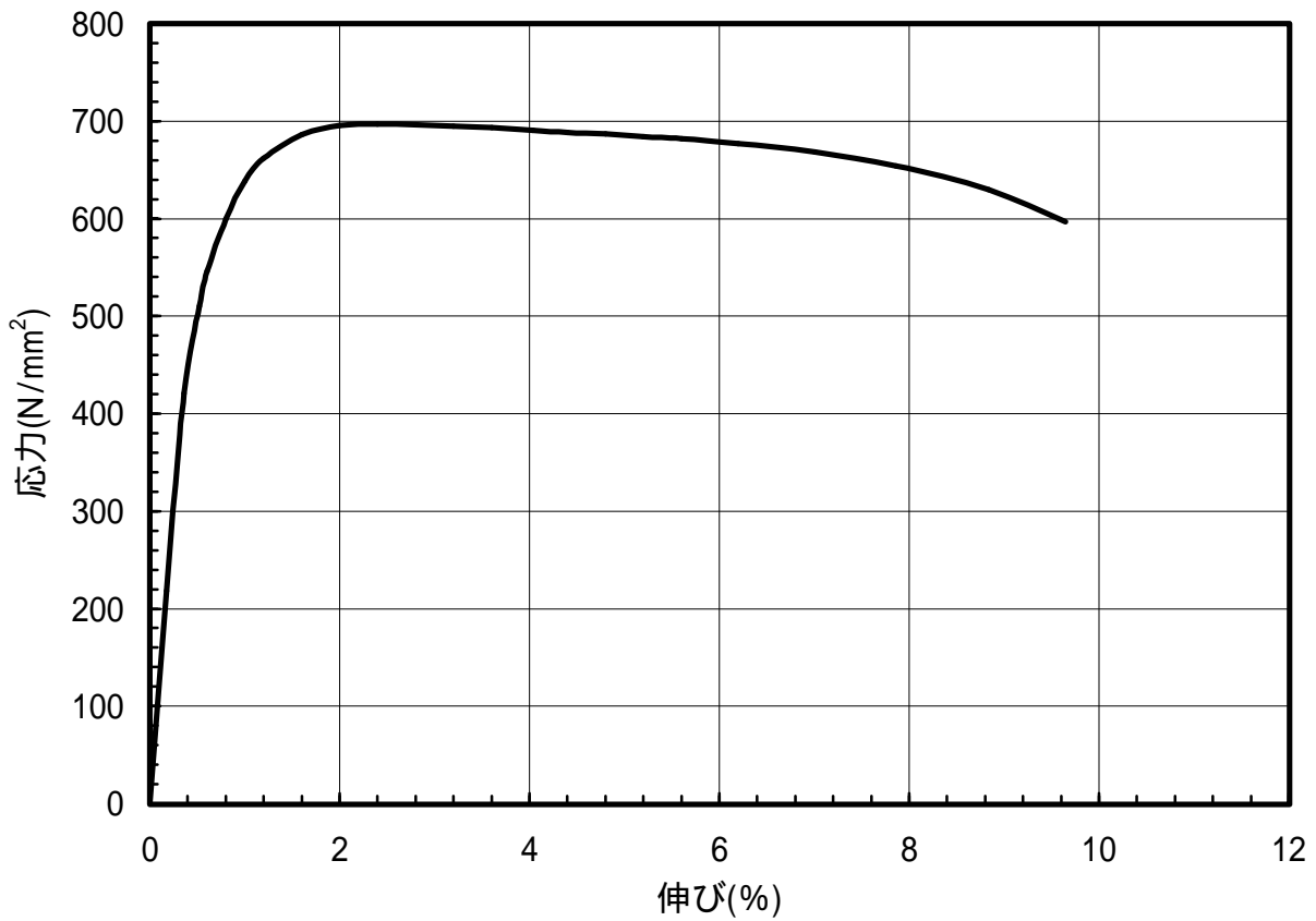
図 1.94 C5191-EH材のS-S曲線(45°)
