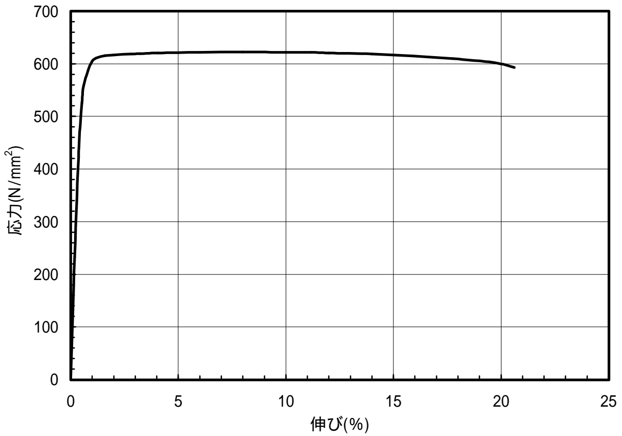
図 1.86 C5191-H材のS-S曲線(L.D.)
