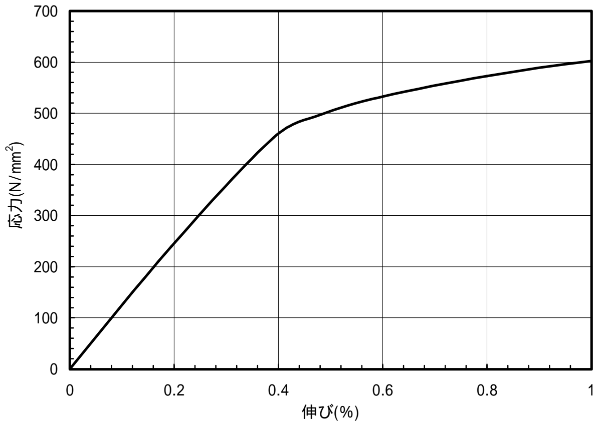
図 1.89 C5191-H材のS-S曲線(45°)
