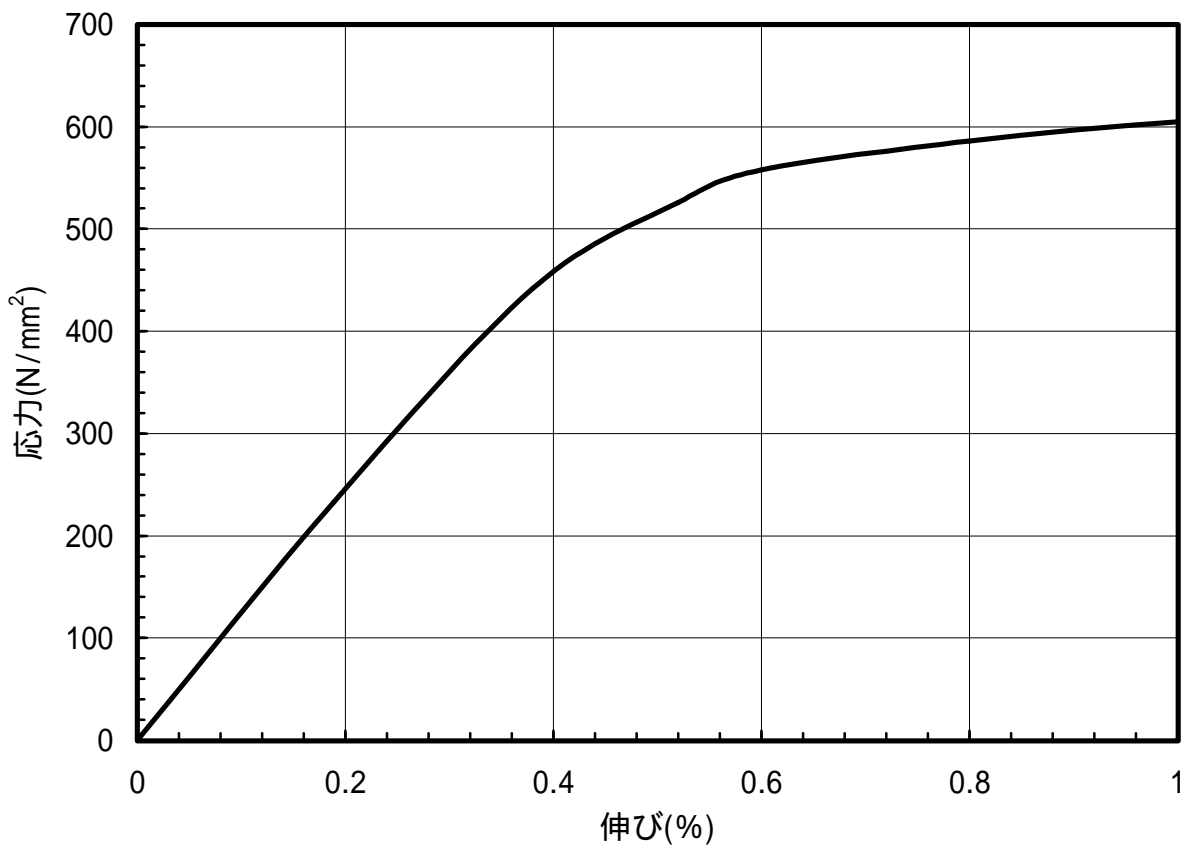
図 1.87 C5191-H材のS-S曲線(L.D.)
