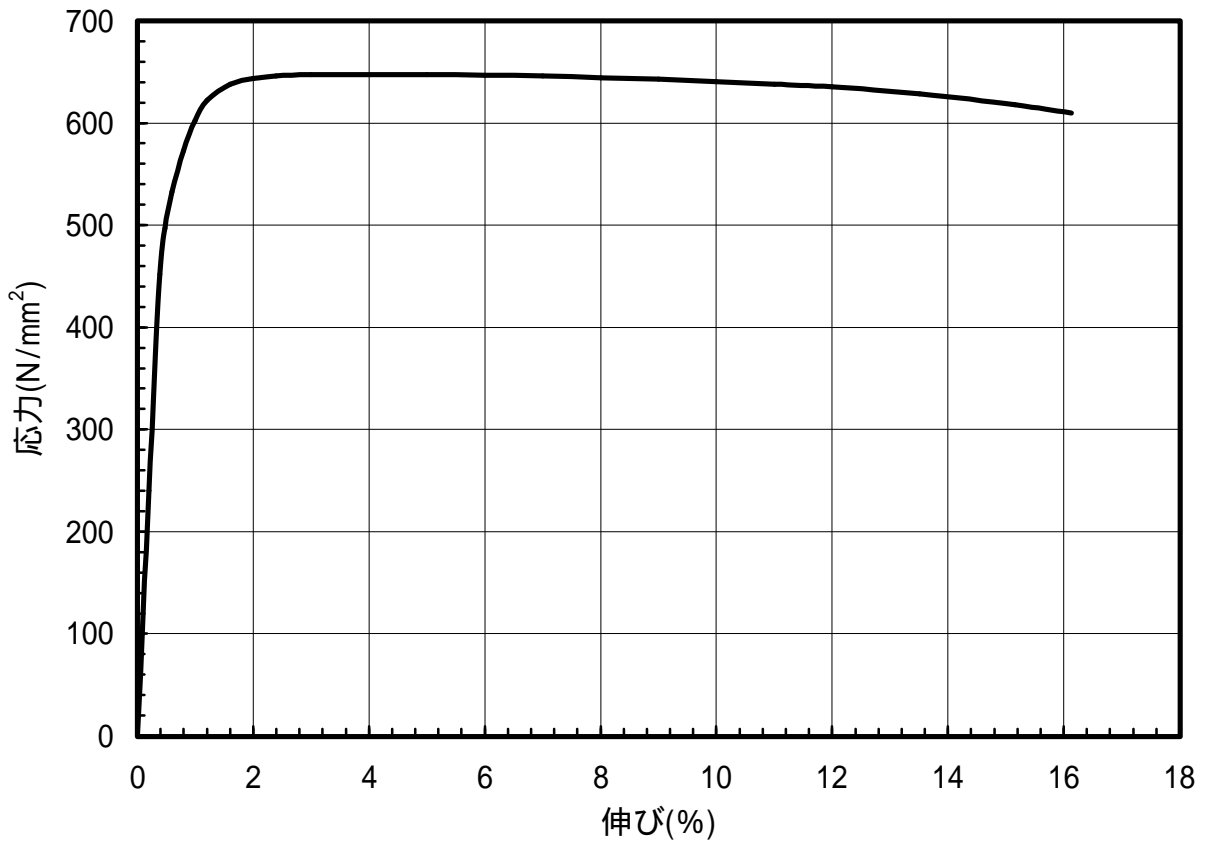
図 1.88 C5191-H材のS-S曲線(45°)
