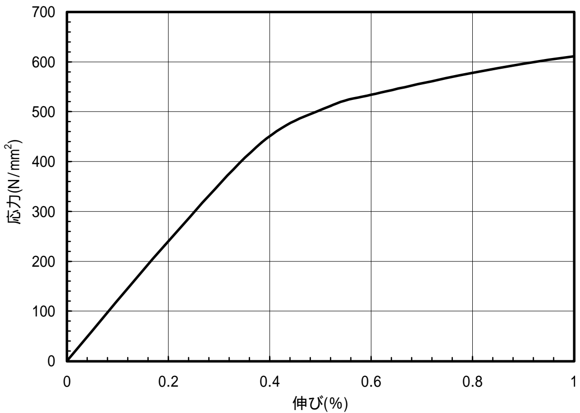
図 1.91 C5191-H材のS-S曲線(T.D.)
