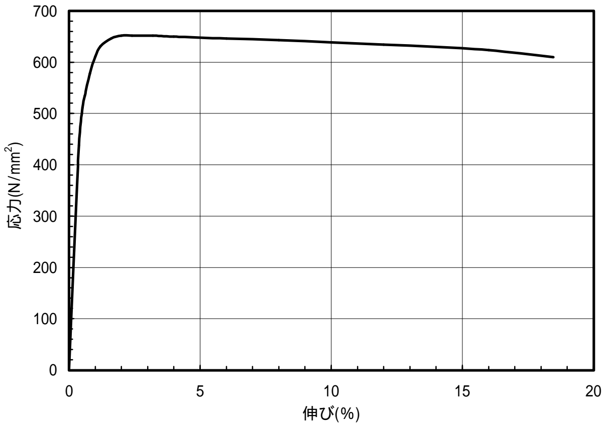
図 1.90 C5191-H材のS-S曲線(T.D.)
