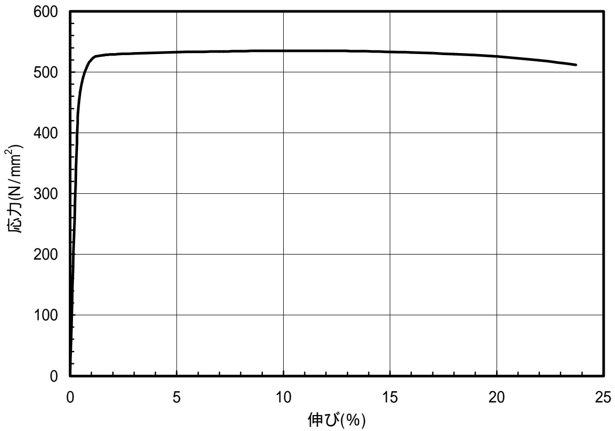
図 1.82 C5191-1/2H材のS-S曲線(45 °)
