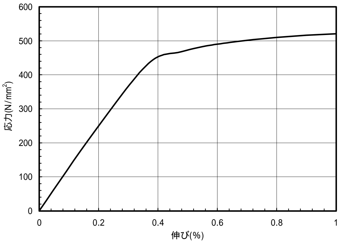
図 1.83 C5191-1/2H材のS-S曲線(45 °)
