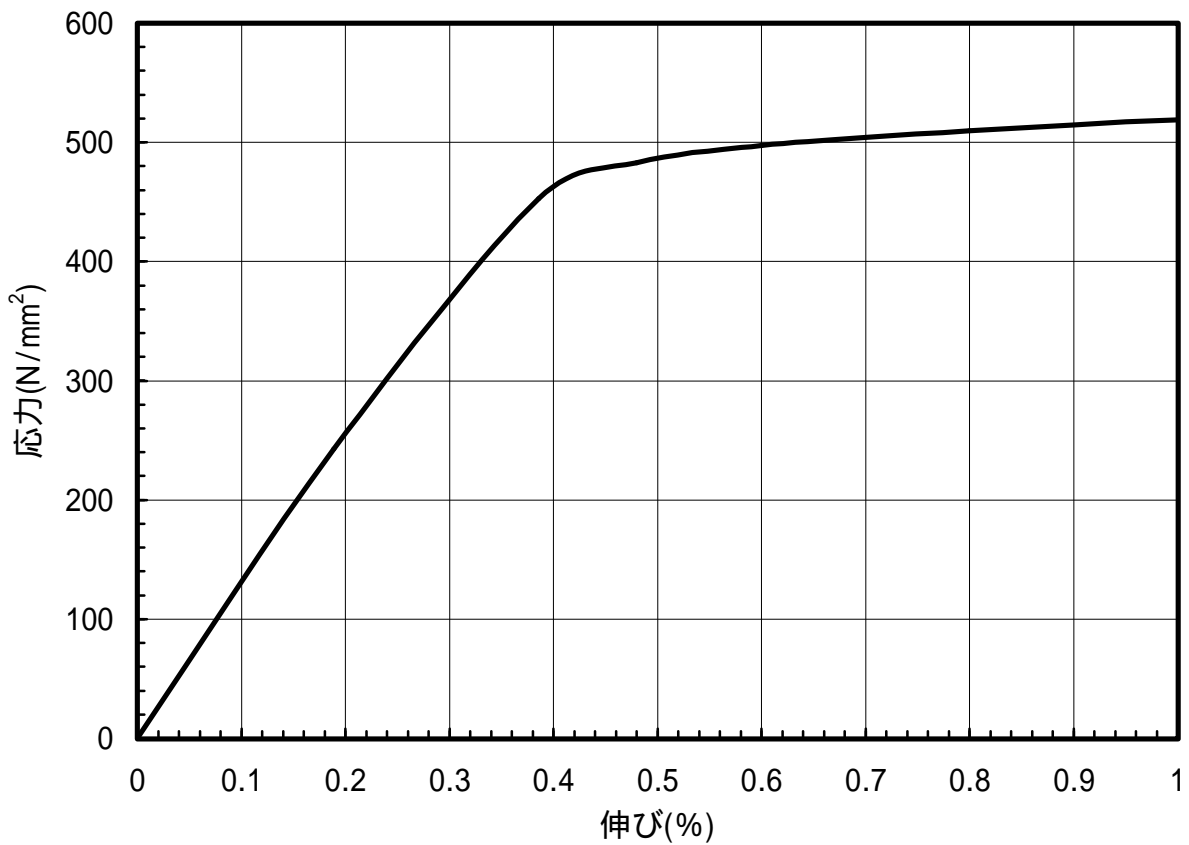
図 1.81 C5191-1/2H材のS-S曲線(L.D.)
