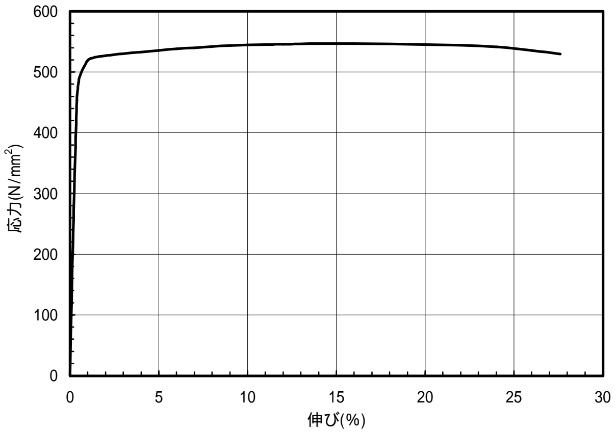
図 1.80 C5191-1/2H材のS-S曲線(L.D.)
