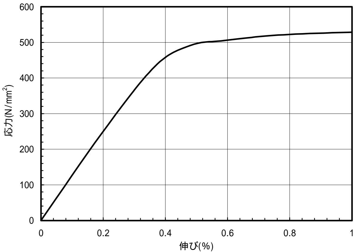
図 1.85 C5191-1/2H材のS-S曲線(T.D.)
