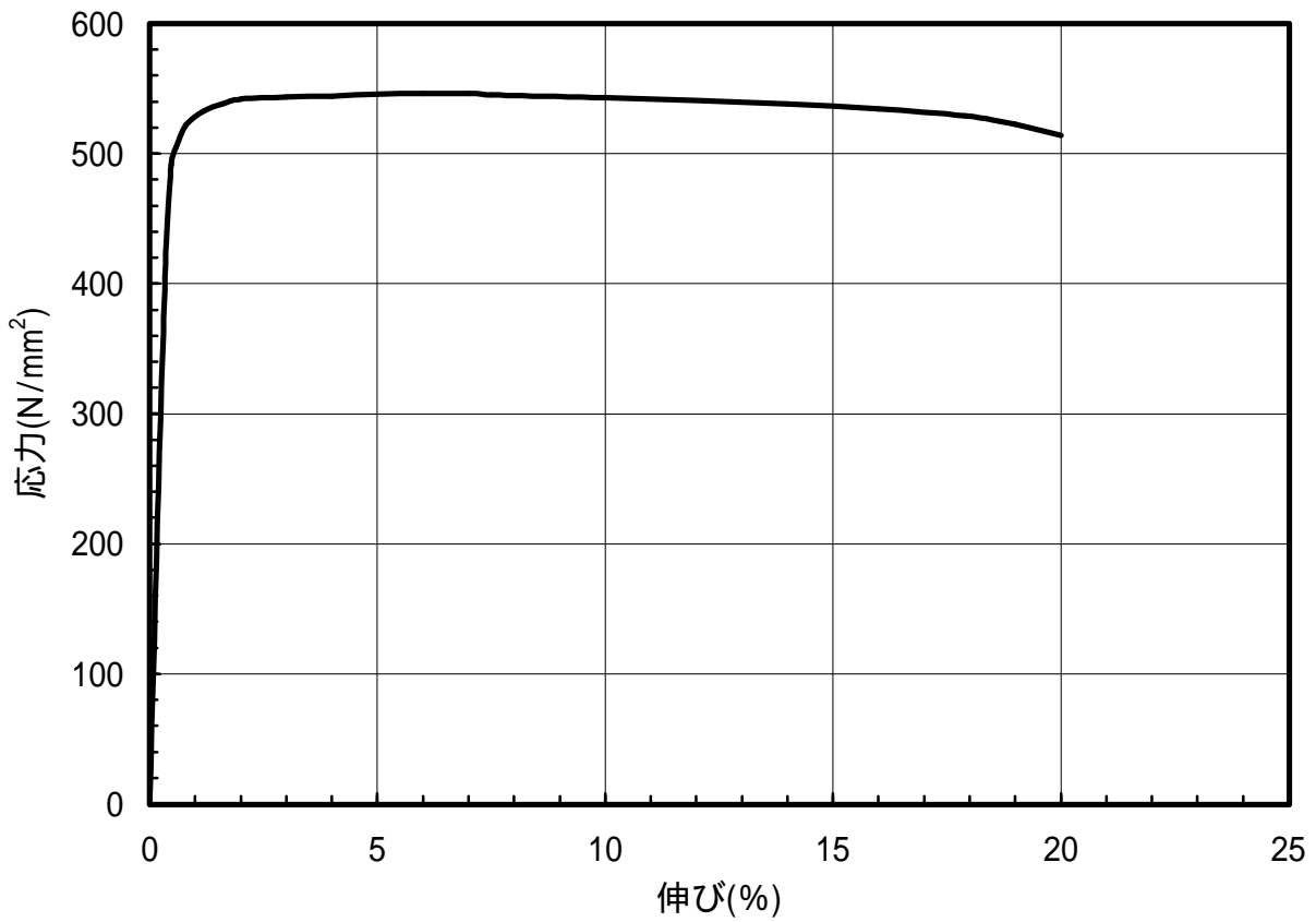
図 1.84 C5191-1/2H材のS-S曲線(T.D.)
