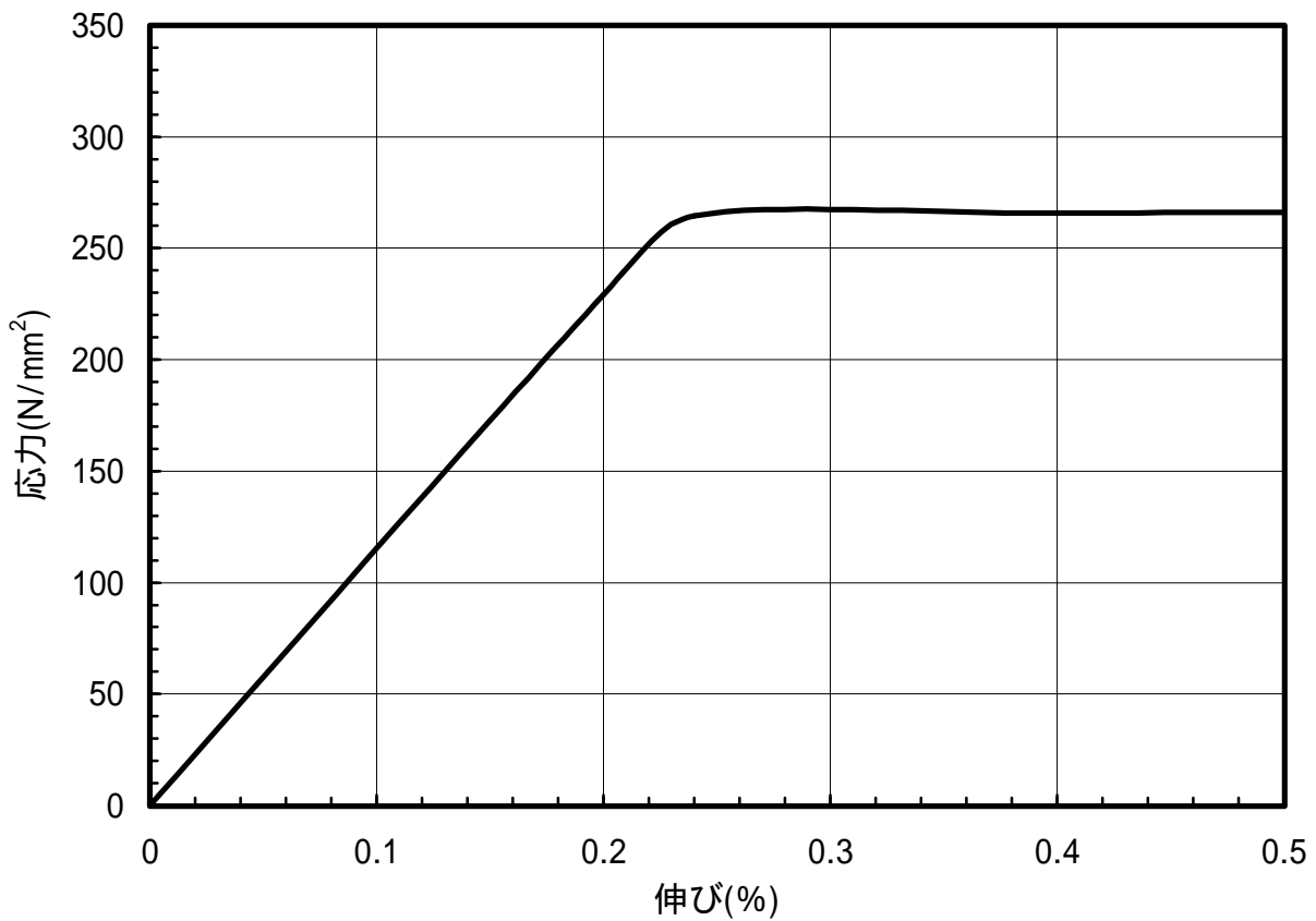
図 1.77 C5191-O材のS-S曲線(45 °)
