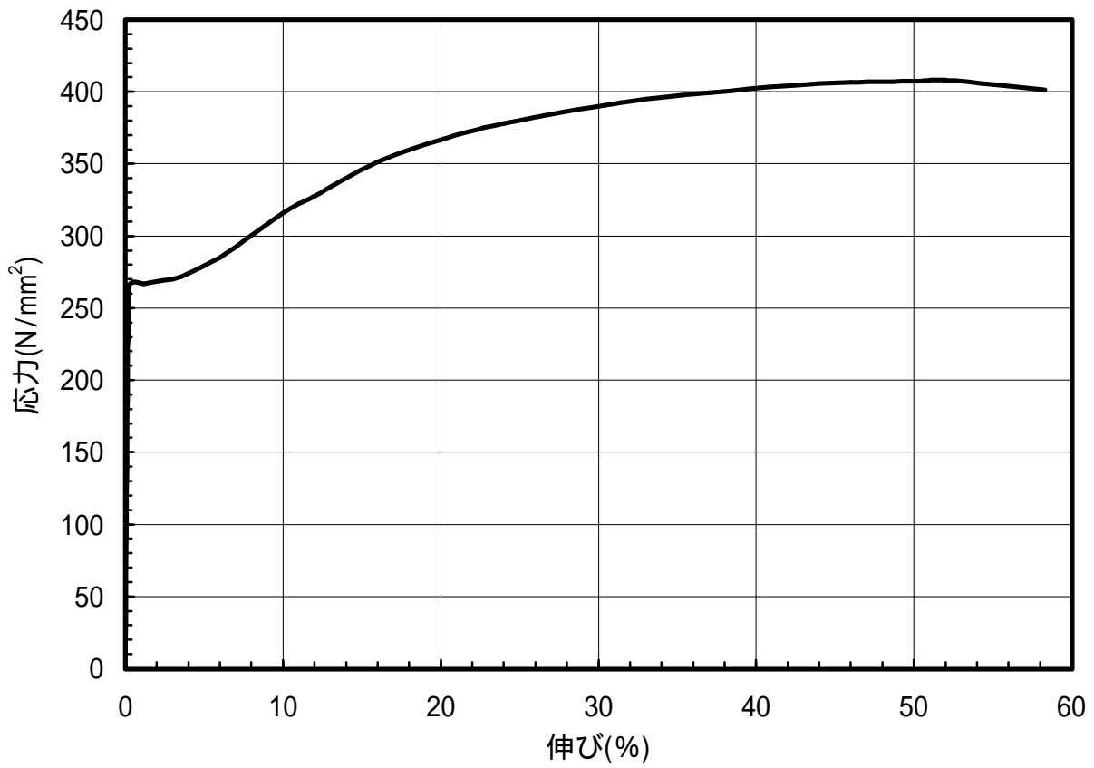
図 1.78 C5191-O材のS-S曲線(T.D.)
