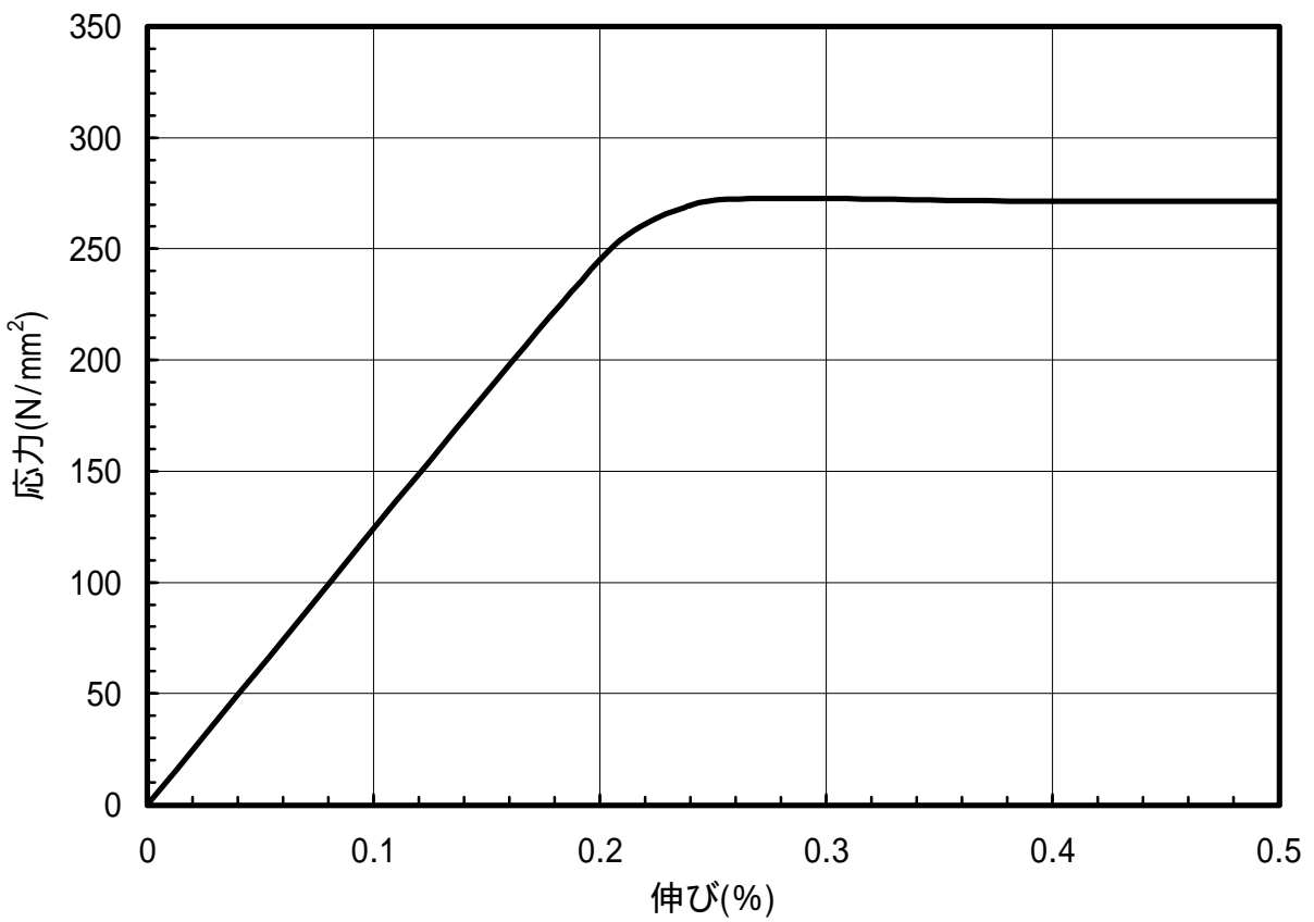
図 1.75 C5191-O材のS-S曲線(L.D.)
