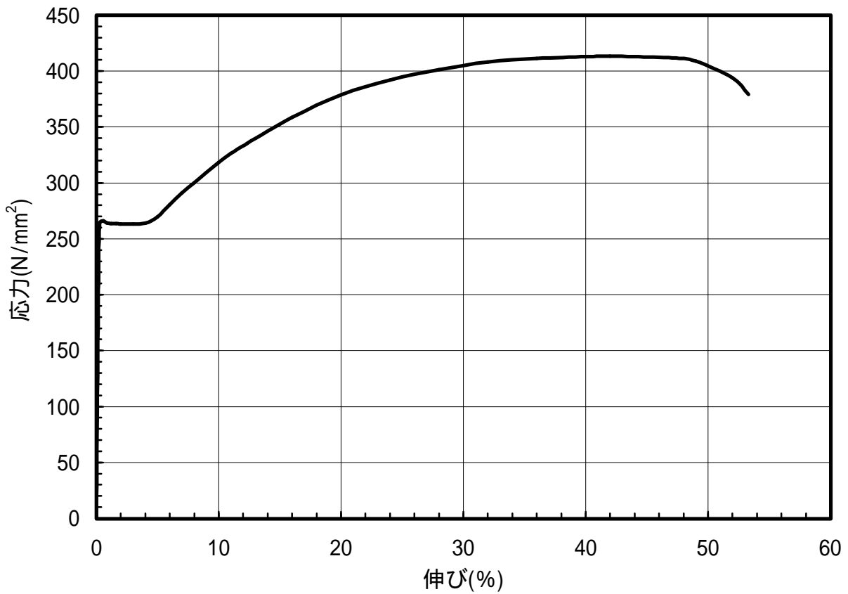
図 1.76 C5191-O材のS-S曲線(45 °)
