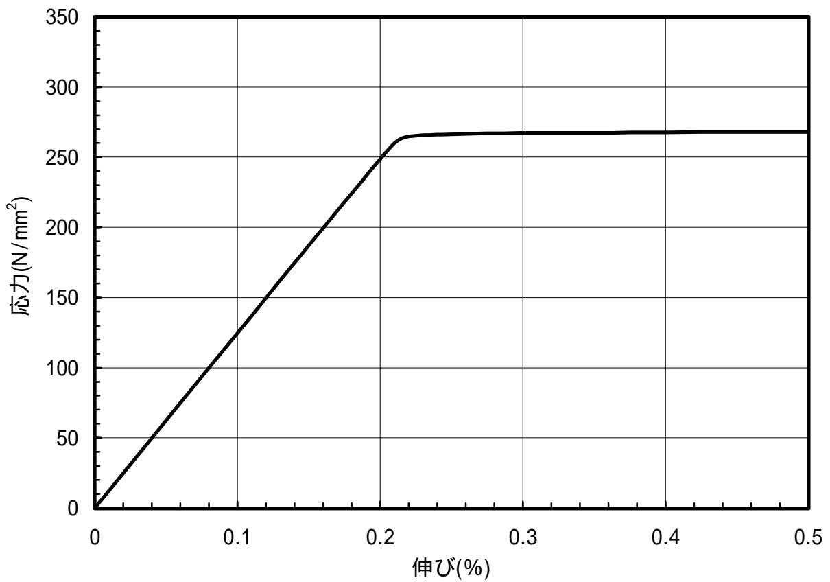
図 1.79 C5191-O材のS-S曲線(T.D.)
