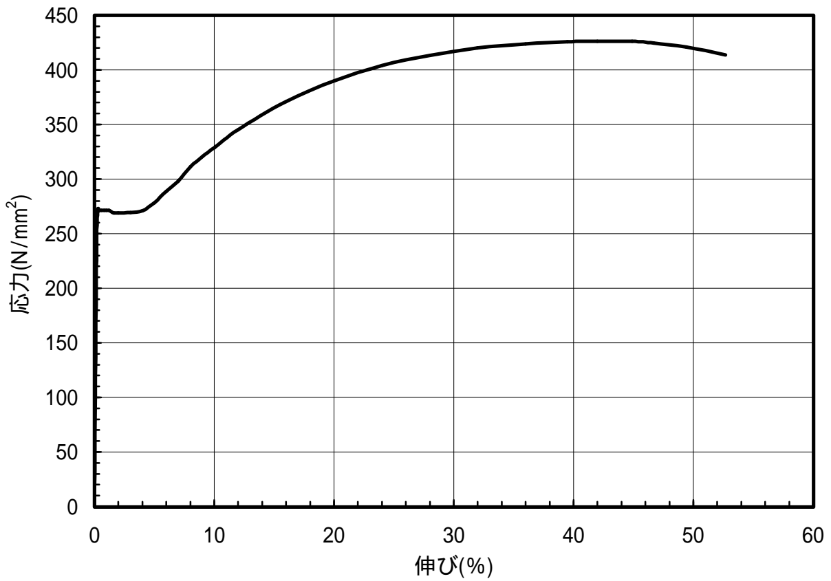
図 1.74 C5191-O材のS-S曲線(L.D.)
