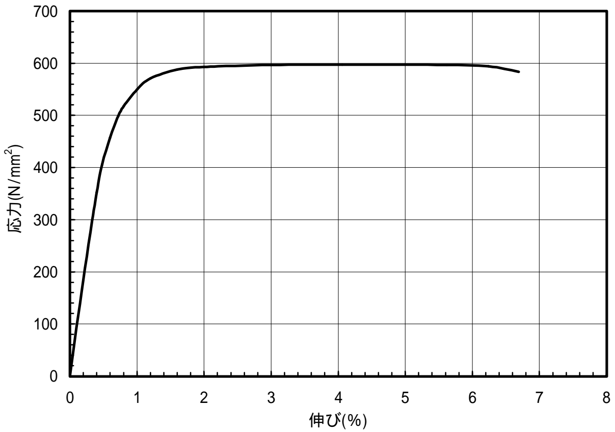
図 1.68 C2801-EH材のS-S曲線(L.D.)
