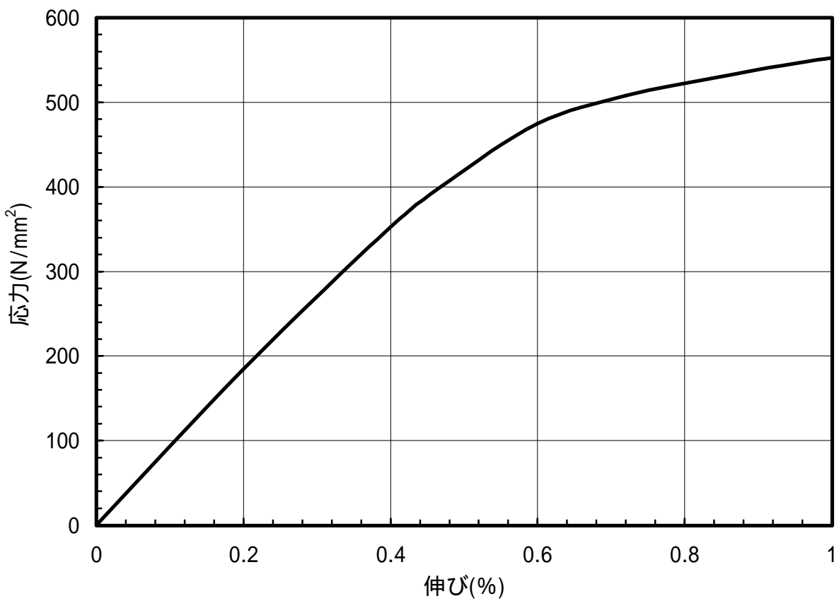
図 1.73 C2801-EH材のS-S曲線(T.D.)
