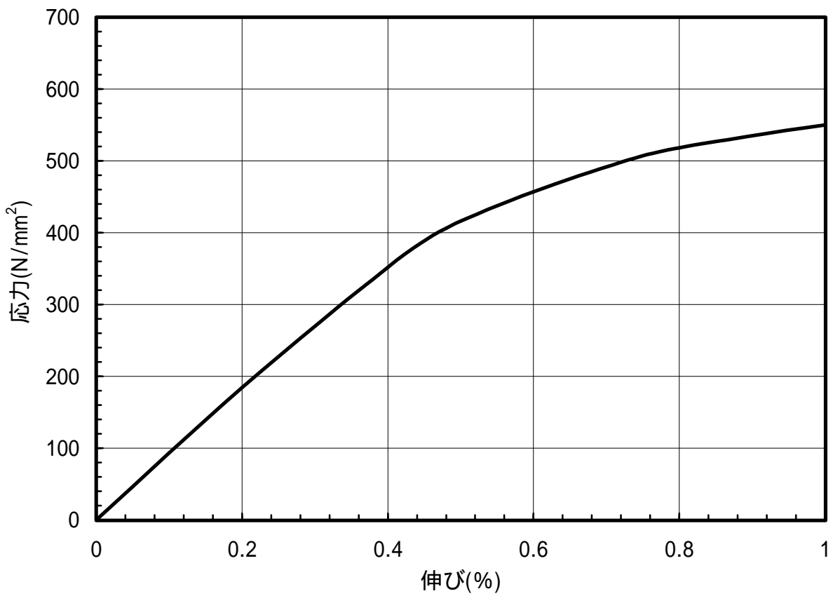
図 1.69 C2801-EH材のS-S曲線(L.D.)
