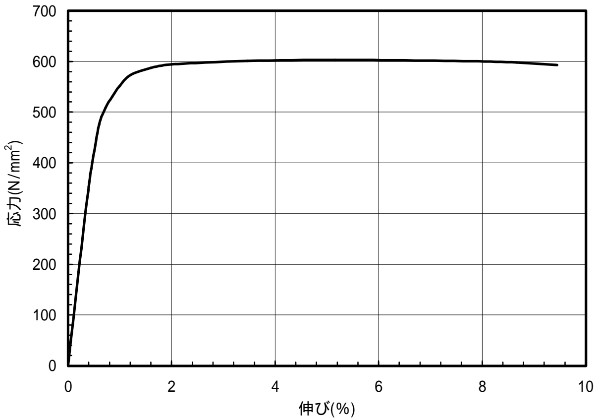
図 1.72 C2801-EH材のS-S曲線(T.D.)
