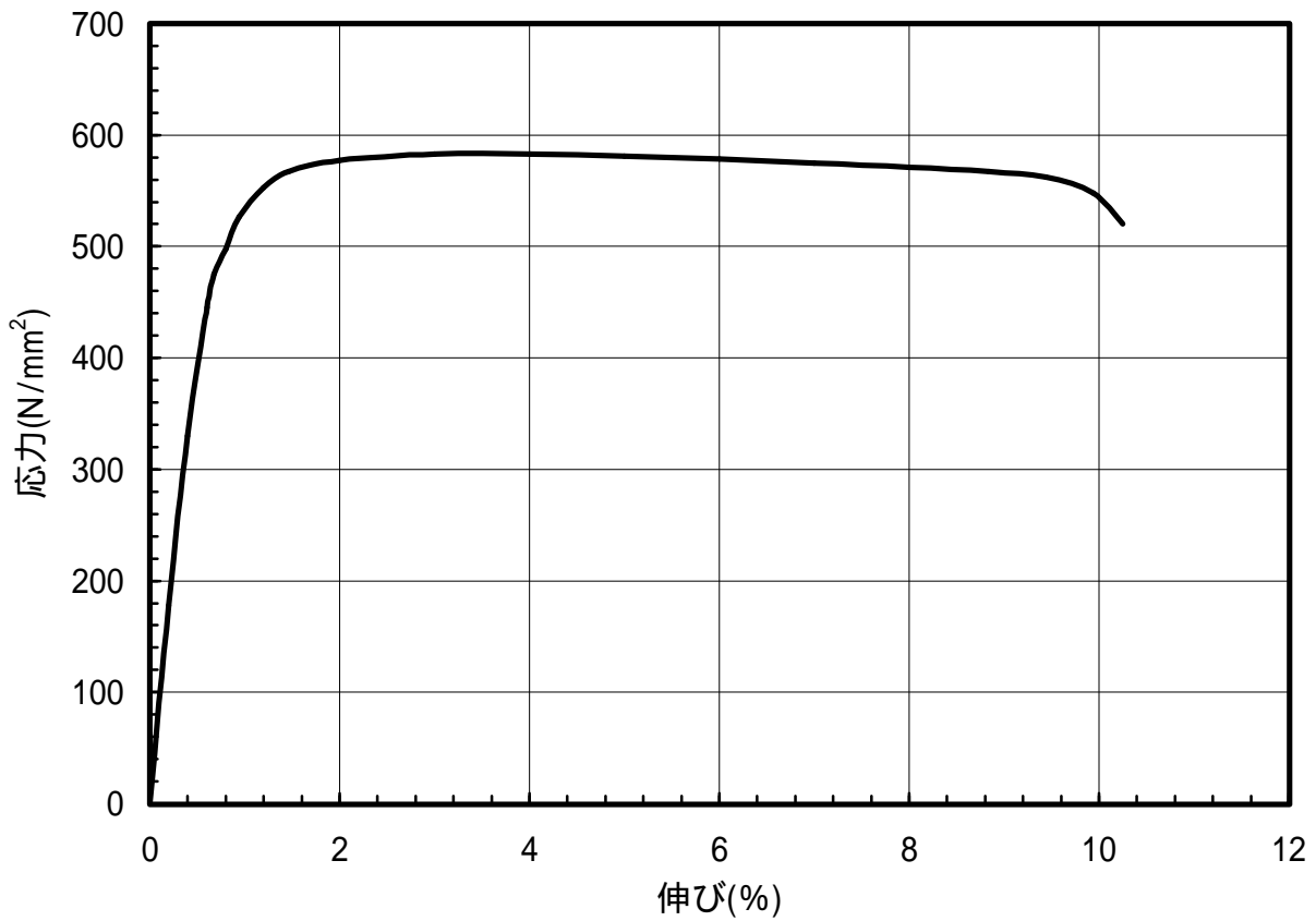
図 1.70 C2801-EH材のS-S曲線(45°)
