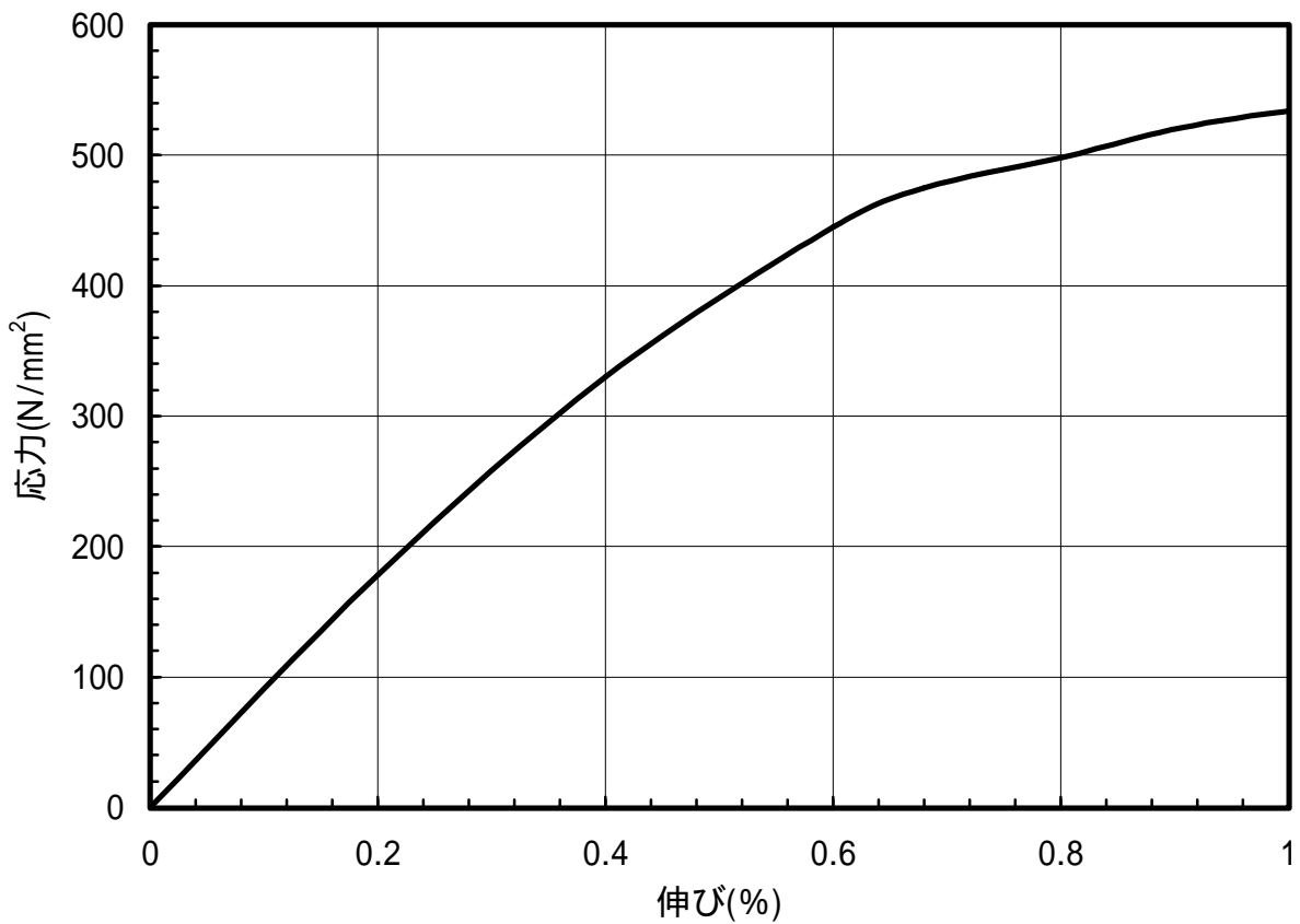
図 1.71 C2801-EH材のS-S曲線(45°)
