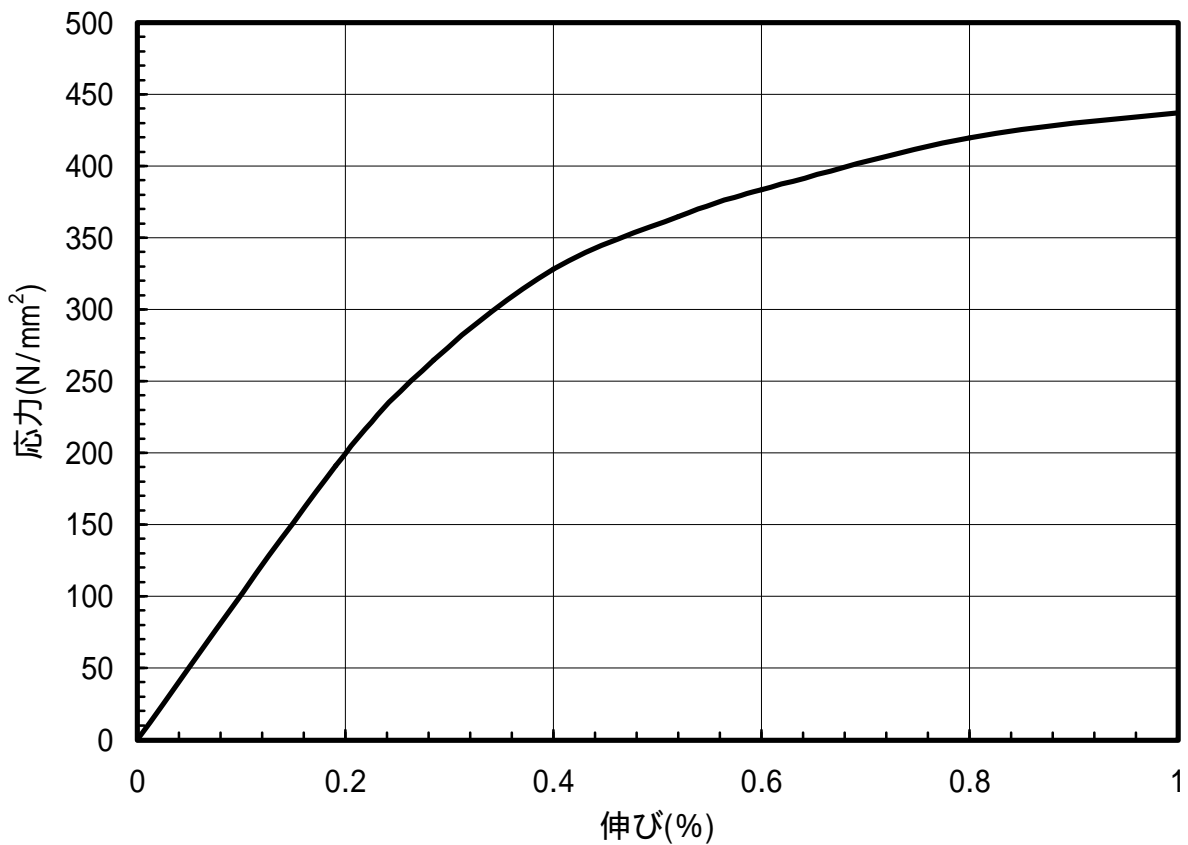
図 1.65 C2801-H材のS-S曲線(45°)
