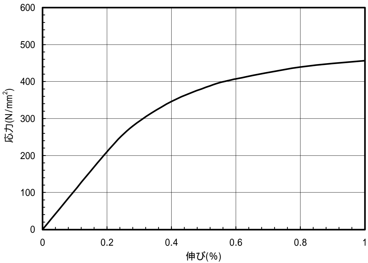
図 1.67 C2801-H材のS-S曲線(T.D.)
