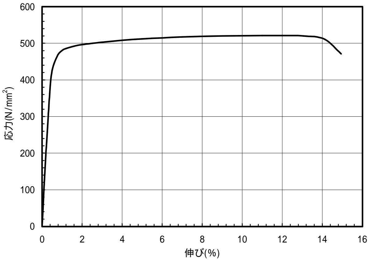
図 1.62 C2801-H材のS-S曲線(L.D.)
