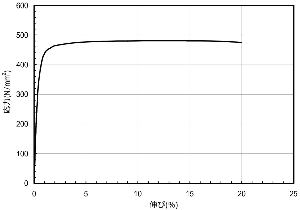
図 1.64 C2801-H材のS-S曲線(45°)
