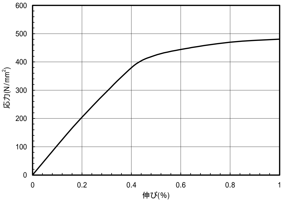
図 1.63 C2801-H材のS-S曲線(L.D.)
