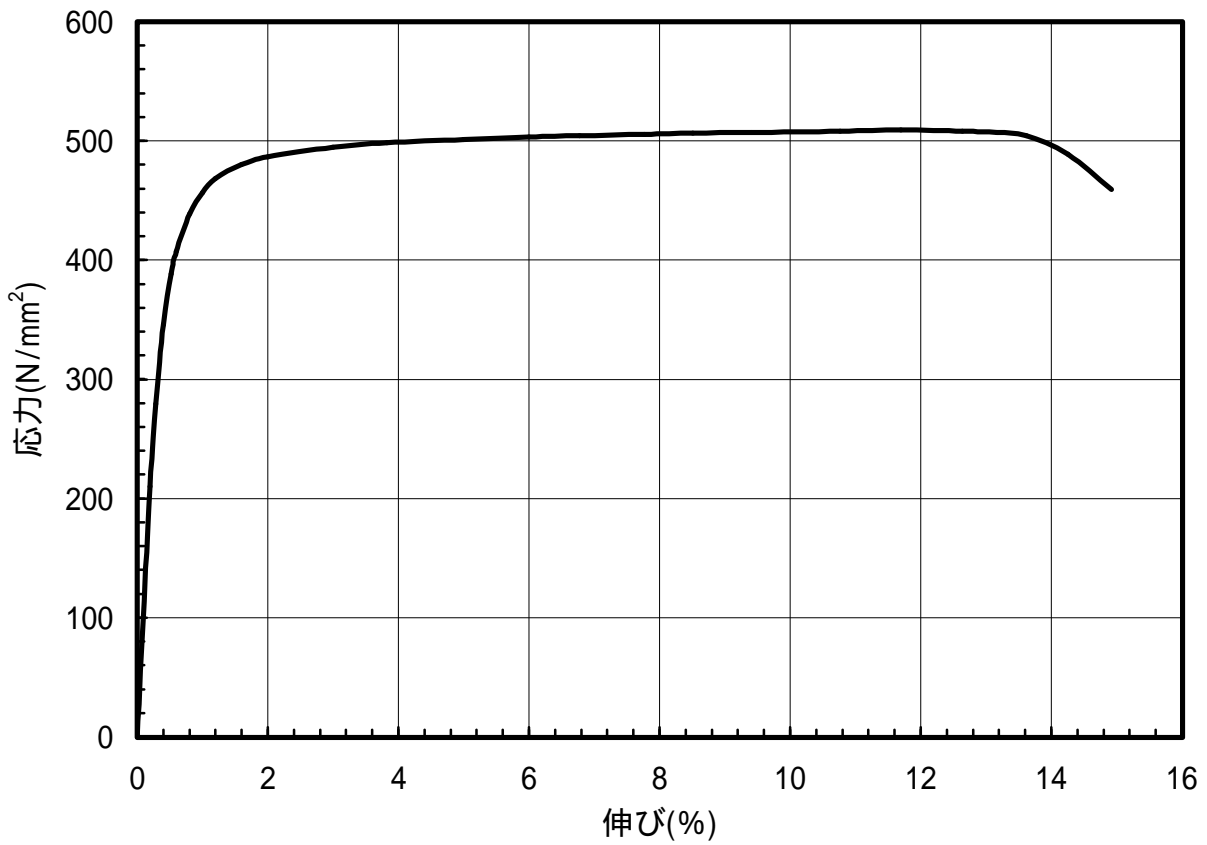
図 1.66 C2801-H材のS-S曲線(T.D.)
