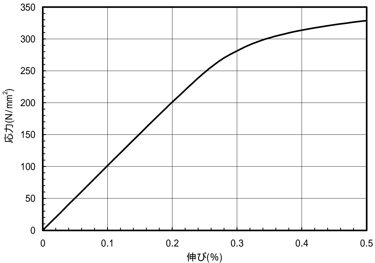
図 1.57 C2801-1/2H材のS-S曲線(L.D.)
