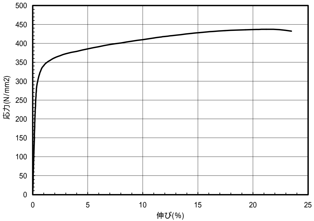
図 1.60 C2801-1/2H材のS-S曲線(T.D.)
