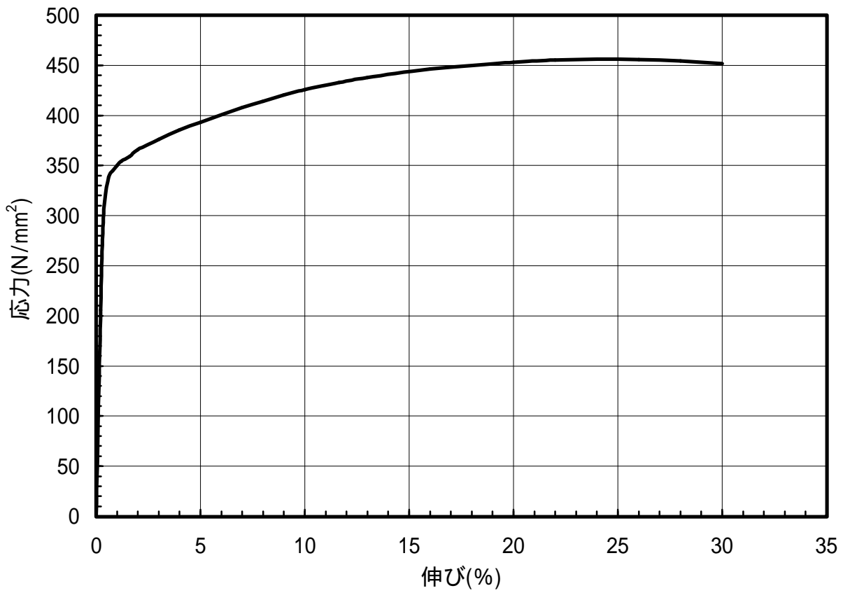
図 1.56 C2801-1/2H材のS-S曲線(L.D.)
