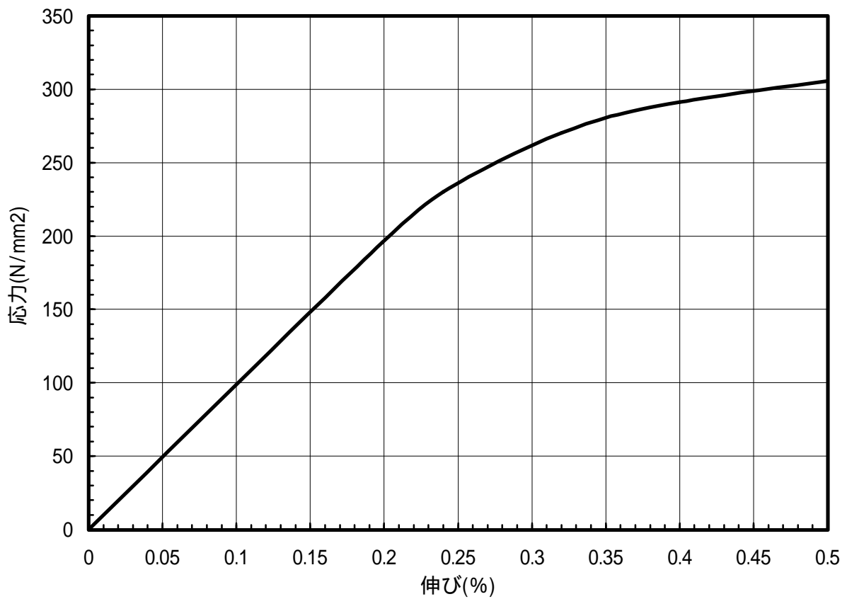
図 1.61 C2801-1/2H材のS-S曲線(T.D.)
