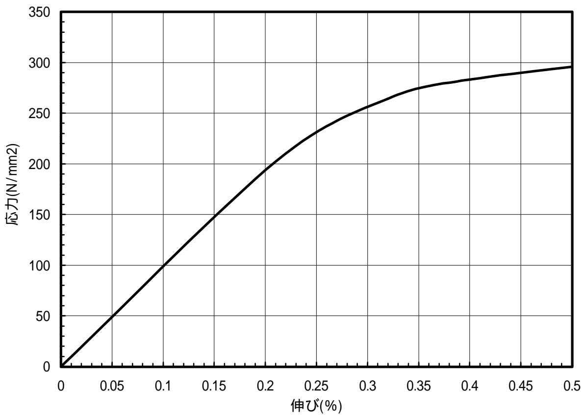
図 1.59 C2801-1/2H材のS-S曲線(45°)
