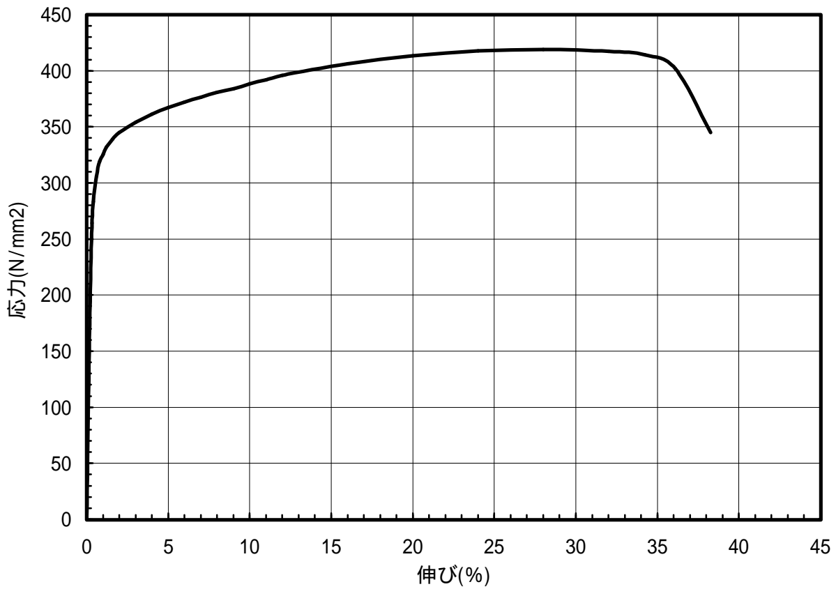
図 1.58 C2800-1/2H材のS-S曲線(45°)
