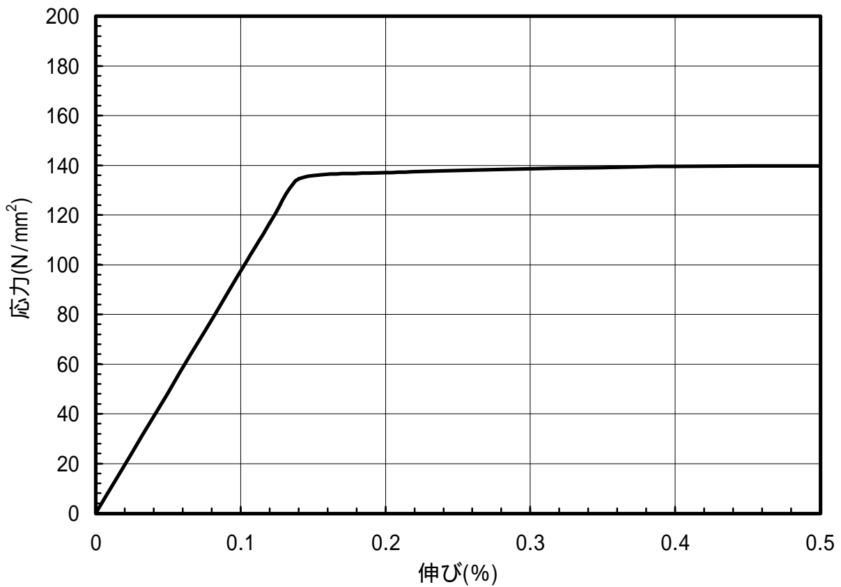
図 1.53 C2801-O材のS-S曲線(45°)
