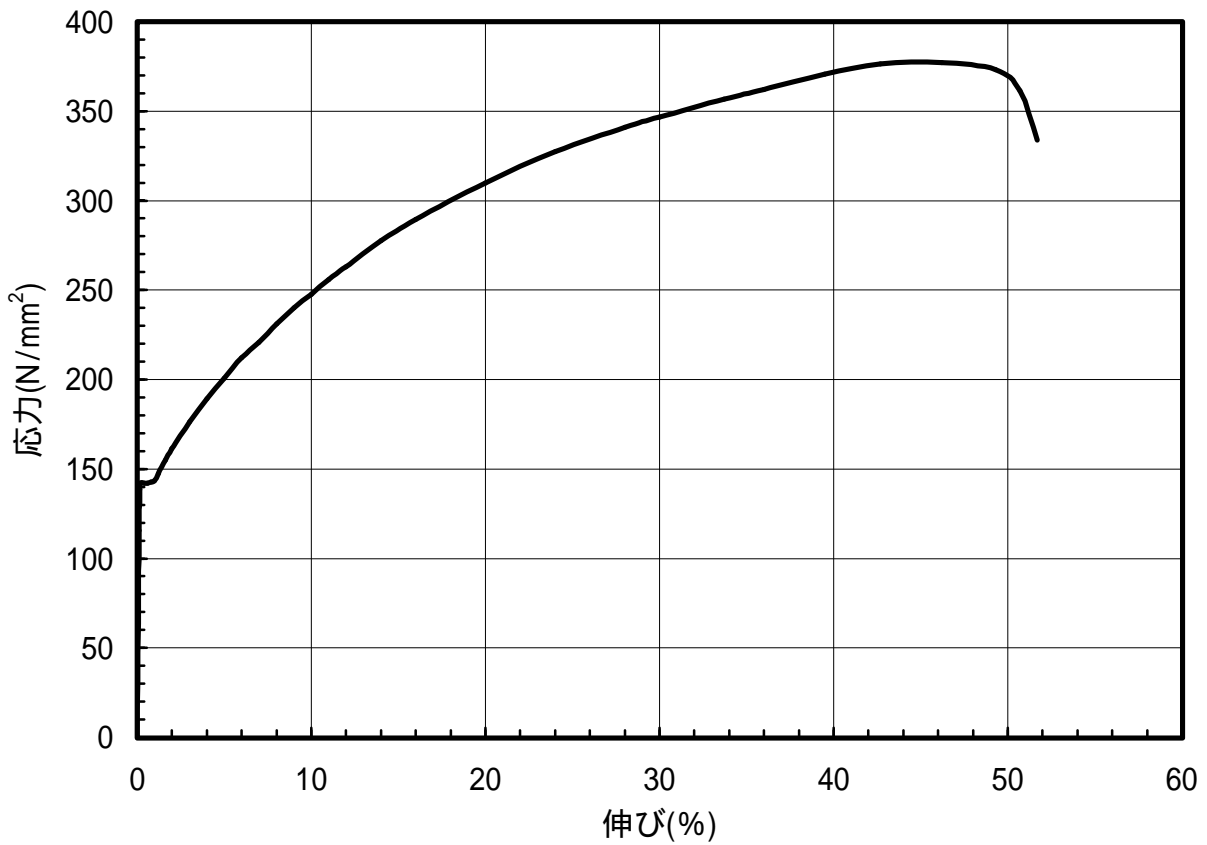
図 1.50 C2801-O材のS-S曲線(L.D.)
