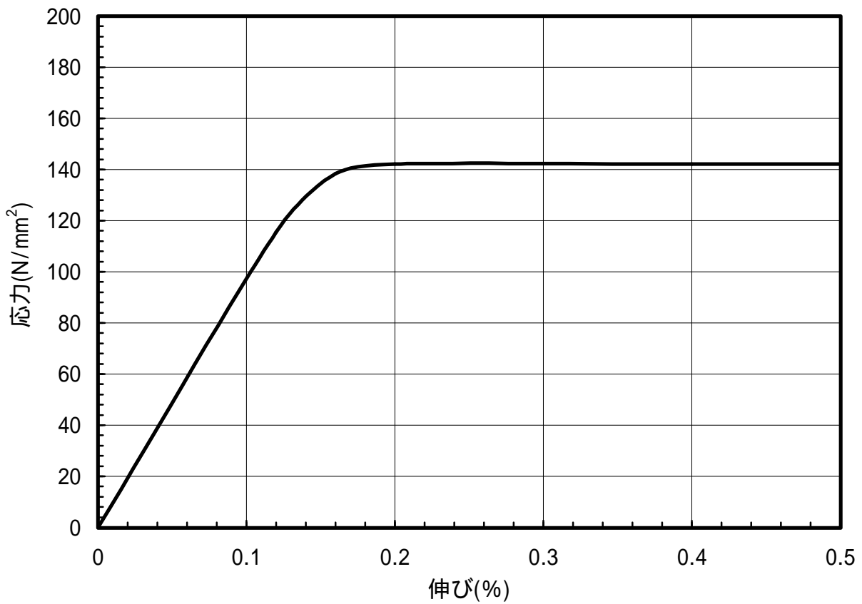
図 1.51 C2801-O材のS-S曲線(L.D.)
