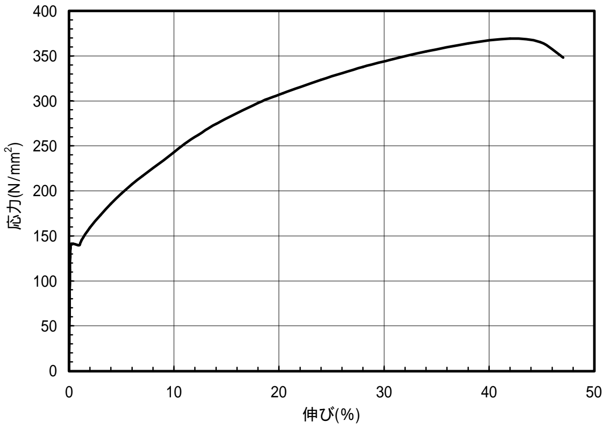
図 1.54 C2801-O材のS-S曲線(T.D.)
