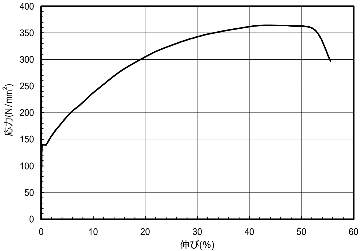
図 1.52 C2801-O材のS-S曲線(45°)
