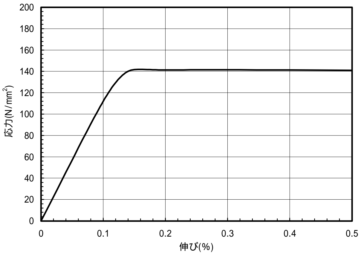
図 1.55 C2801-O材のS-S曲線(T.D.)
