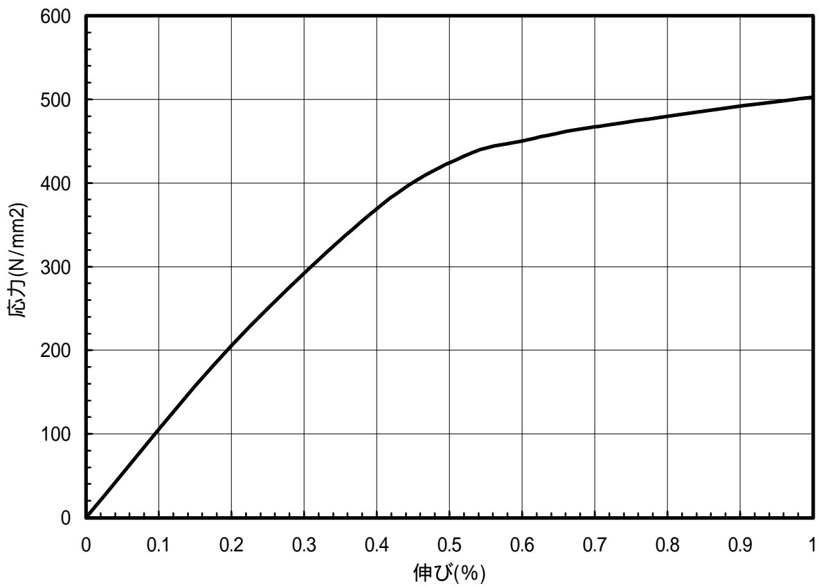
図 1.47 C2600-EH材のS-S曲線(45°)
