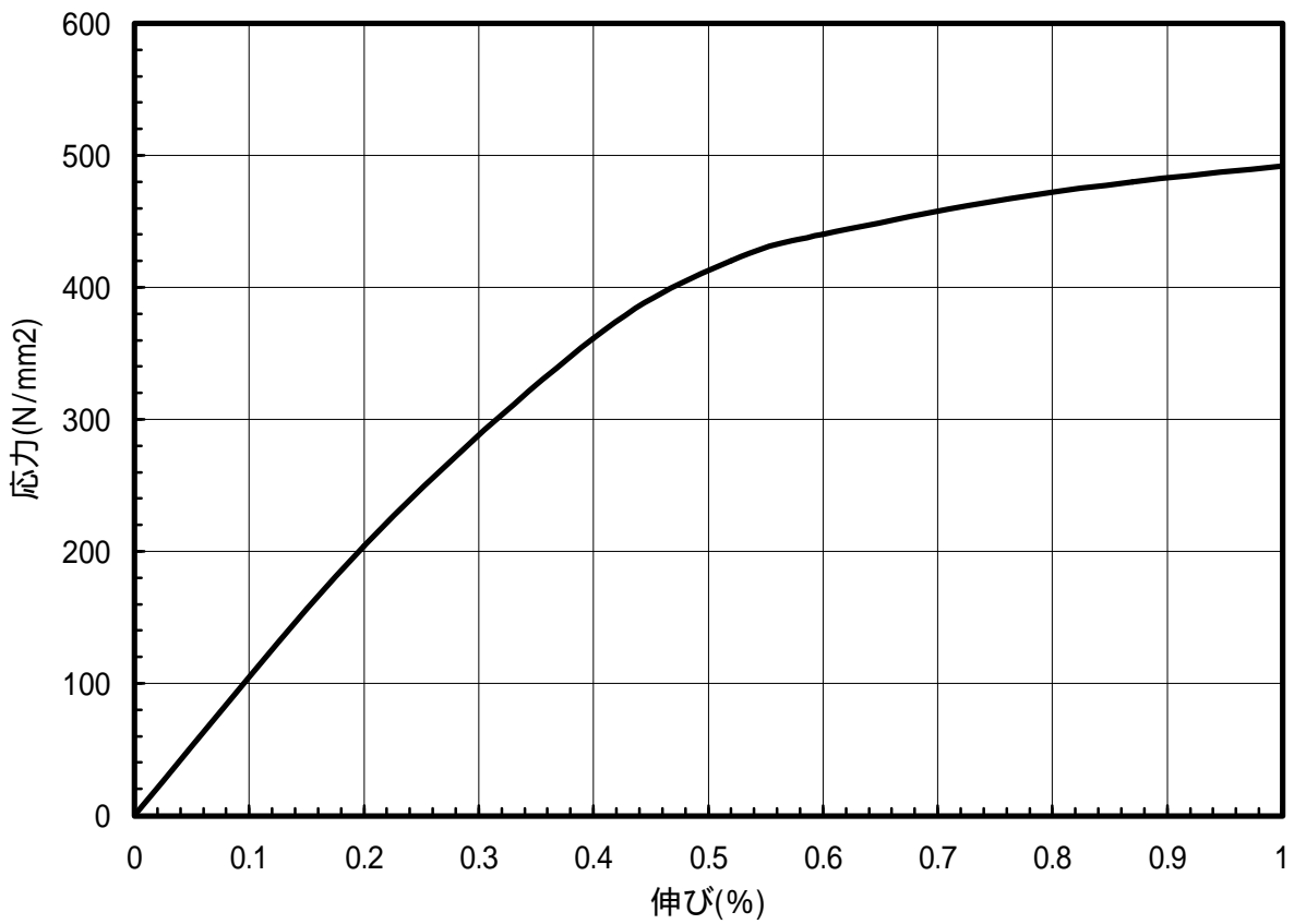
図 1.49 C2600-EH材のS-S曲線(T.D.)
