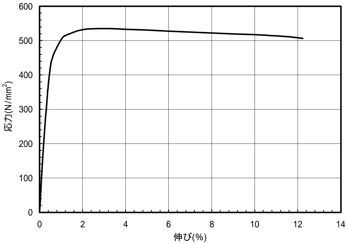
図 1.46 C2600-EH材のS-S曲線(45°)
