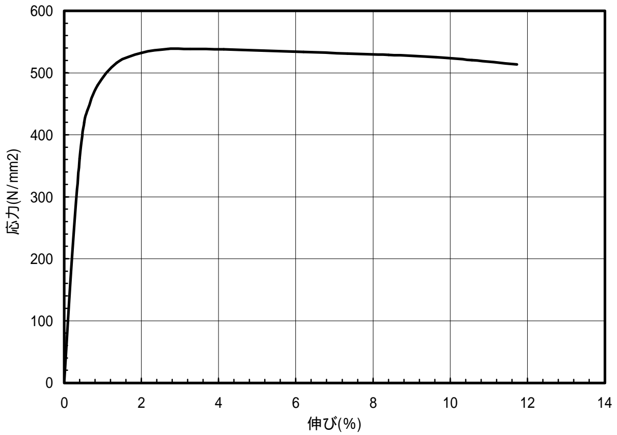
図 1.48 C2600-EH材のS-S曲線(T.D.)
