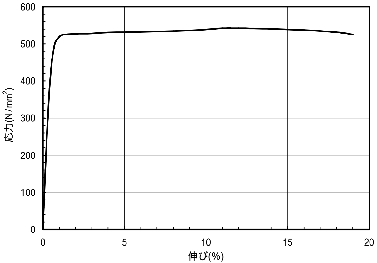
図 1.44 C2600-EH材のS-S曲線(L.D.)
