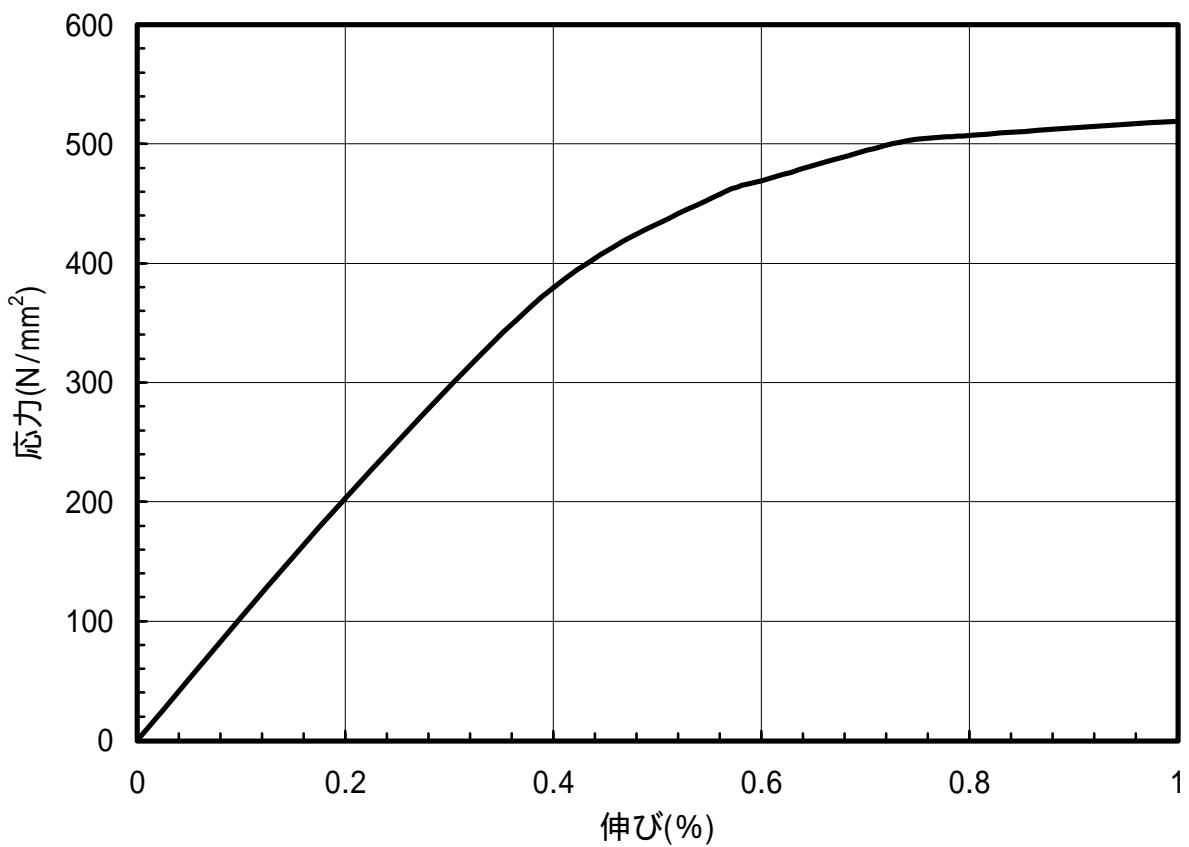
図 1.45 C2600-EH材のS-S曲線(L.D.)
