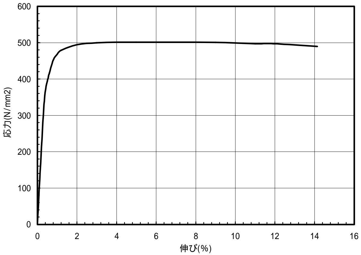
図 1.42 C2600-H材のS-S曲線(T.D.)
