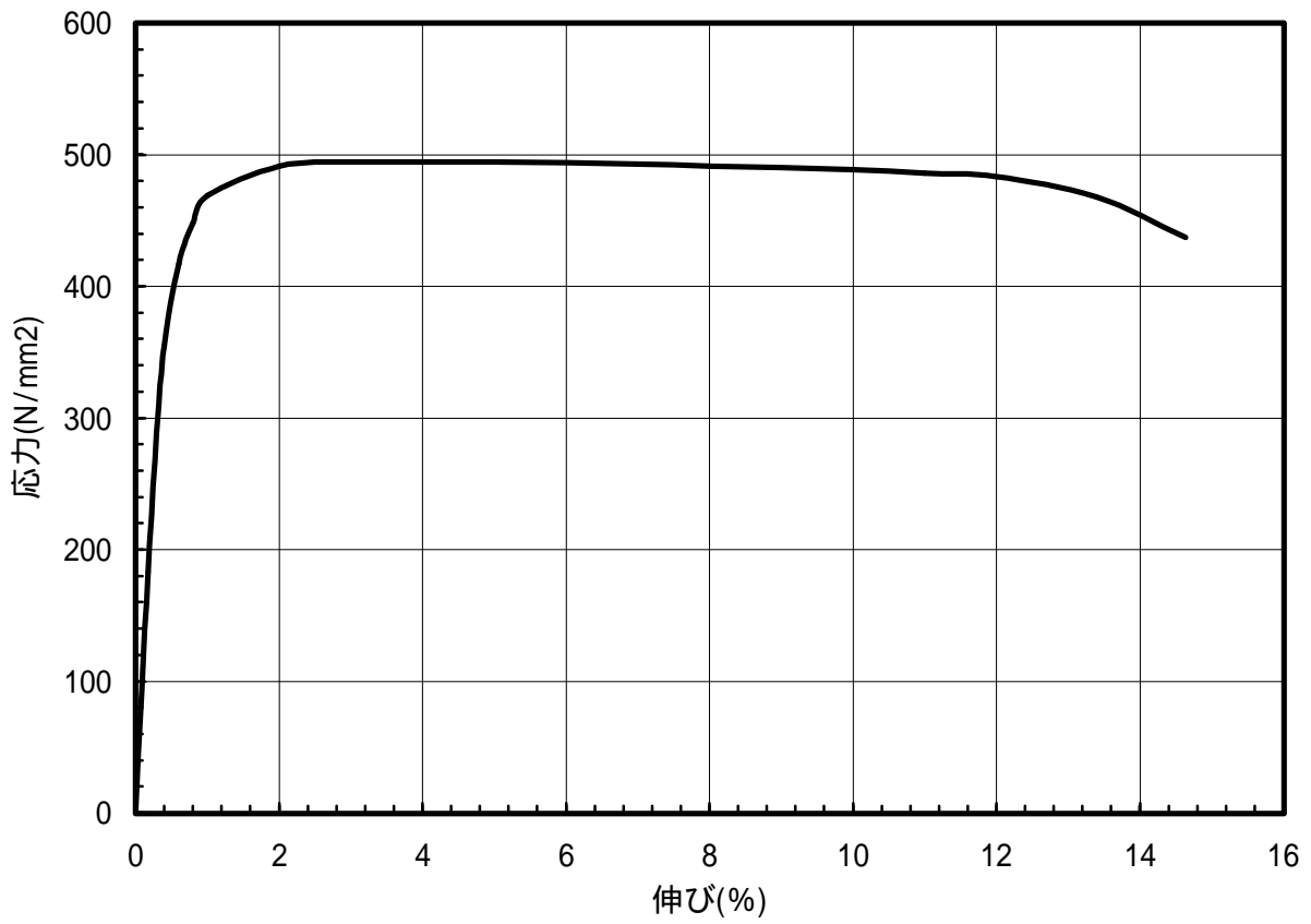
図 140 C2600-H材のS-S曲線(45 °)
