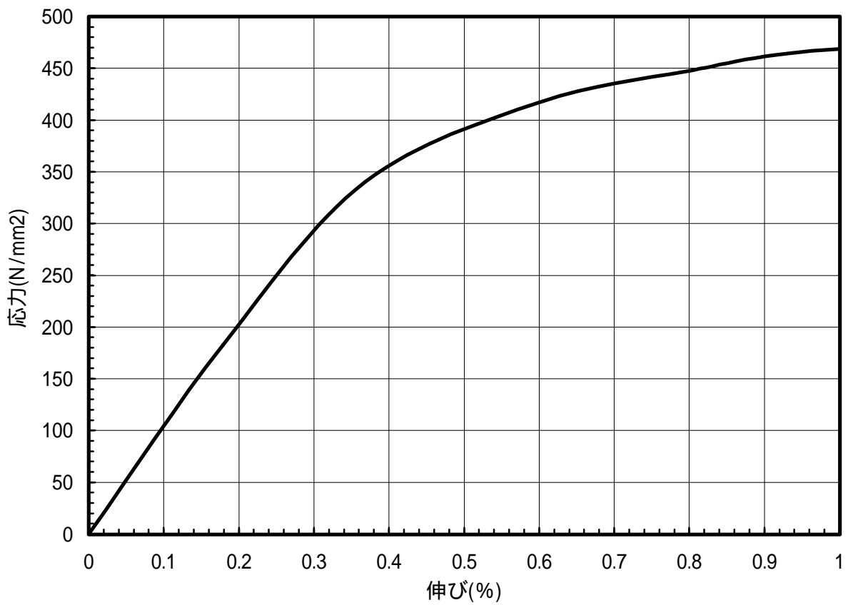
図 1.41 C2600-H材のS-S曲線(45 °)
