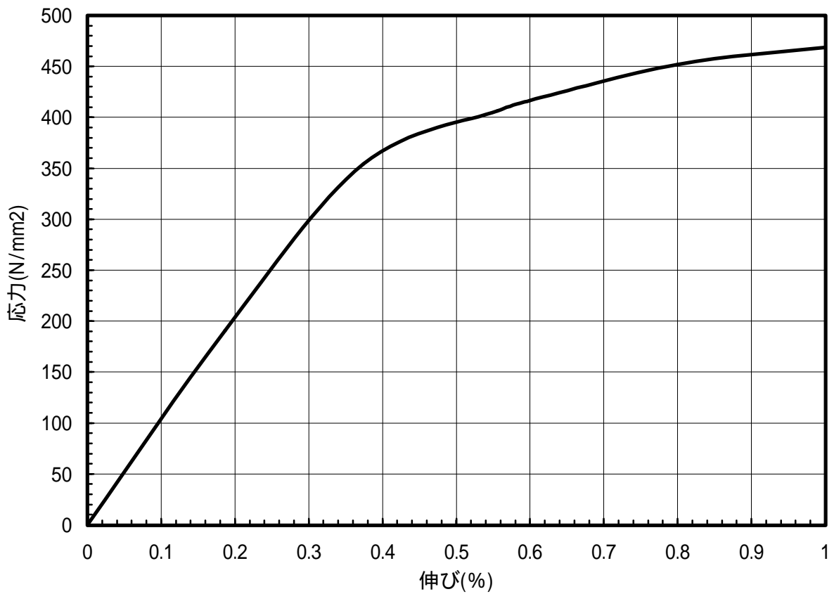
図 1.43 C2600-H材のS-S曲線(T.D.)
