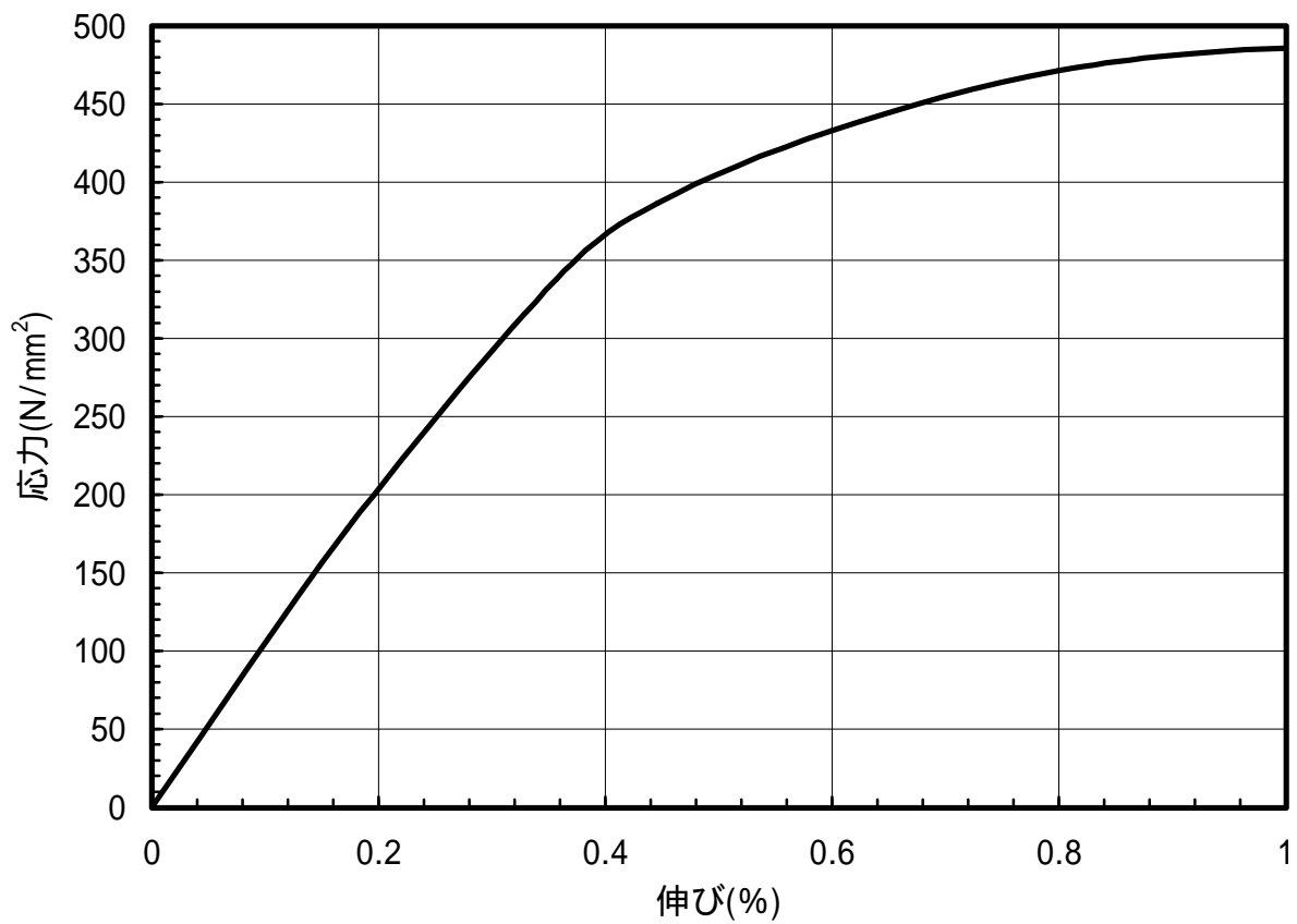
図 1.39 C2600-H材のS-S曲線(L.D.)
