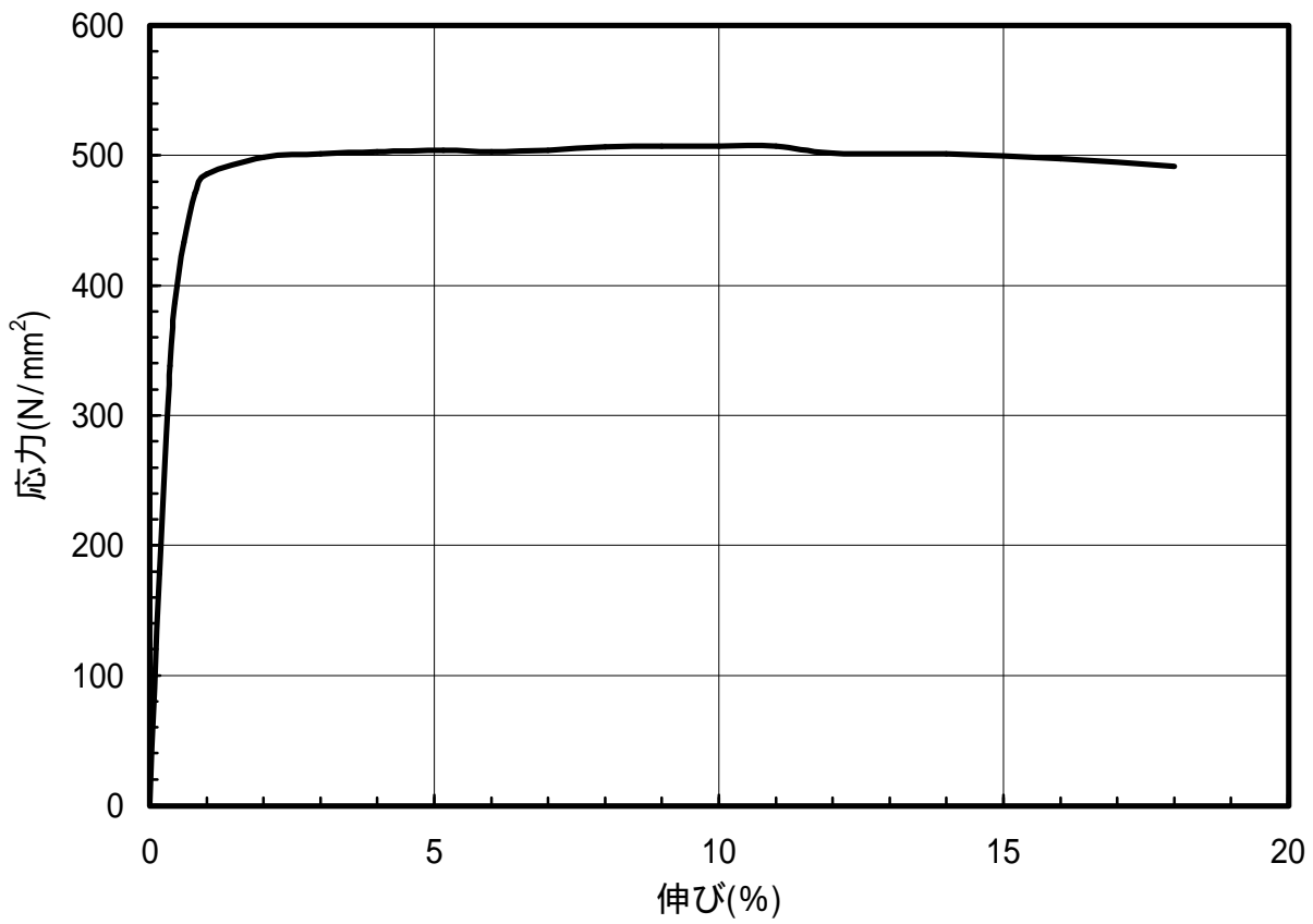
図 1.38 C2600-H材のS-S曲線(L.D.)
