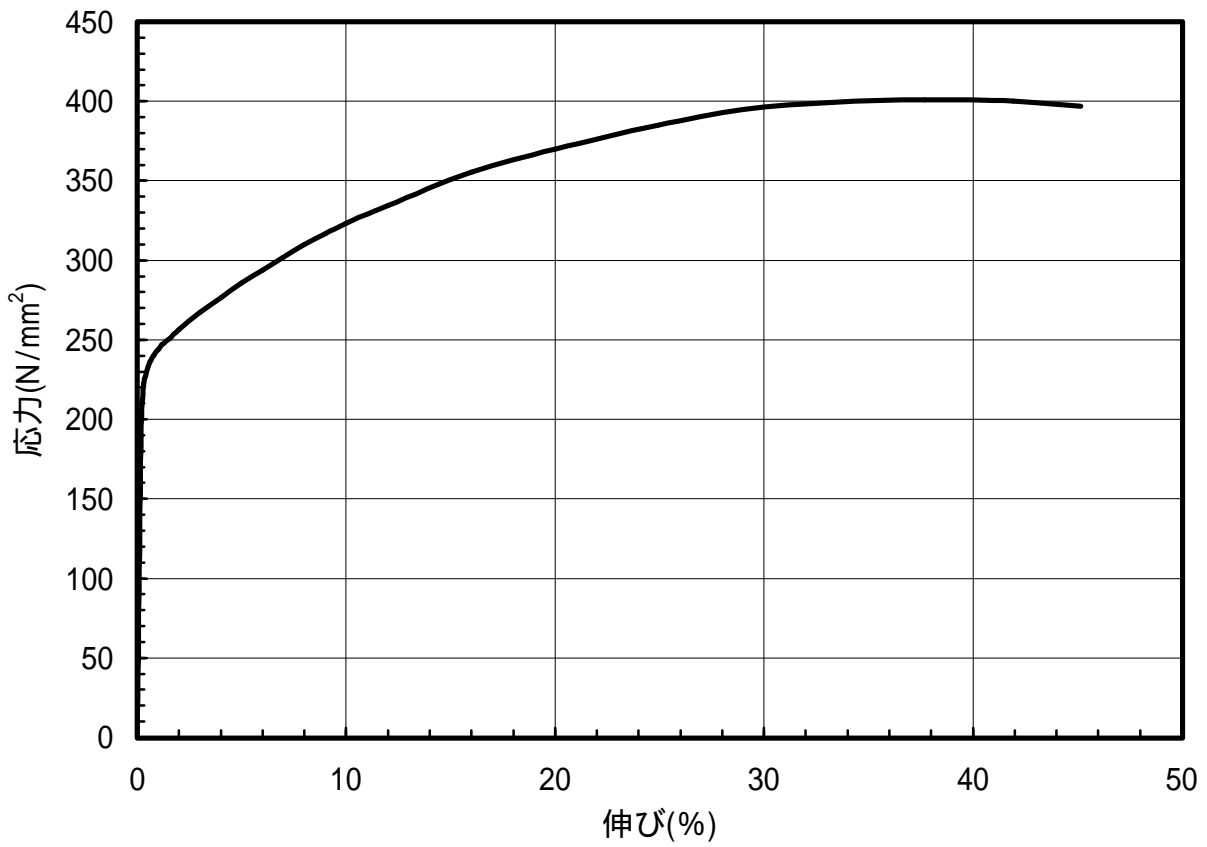
図 1.32 C2600-1/2H材のS-S曲線(L.D.)
