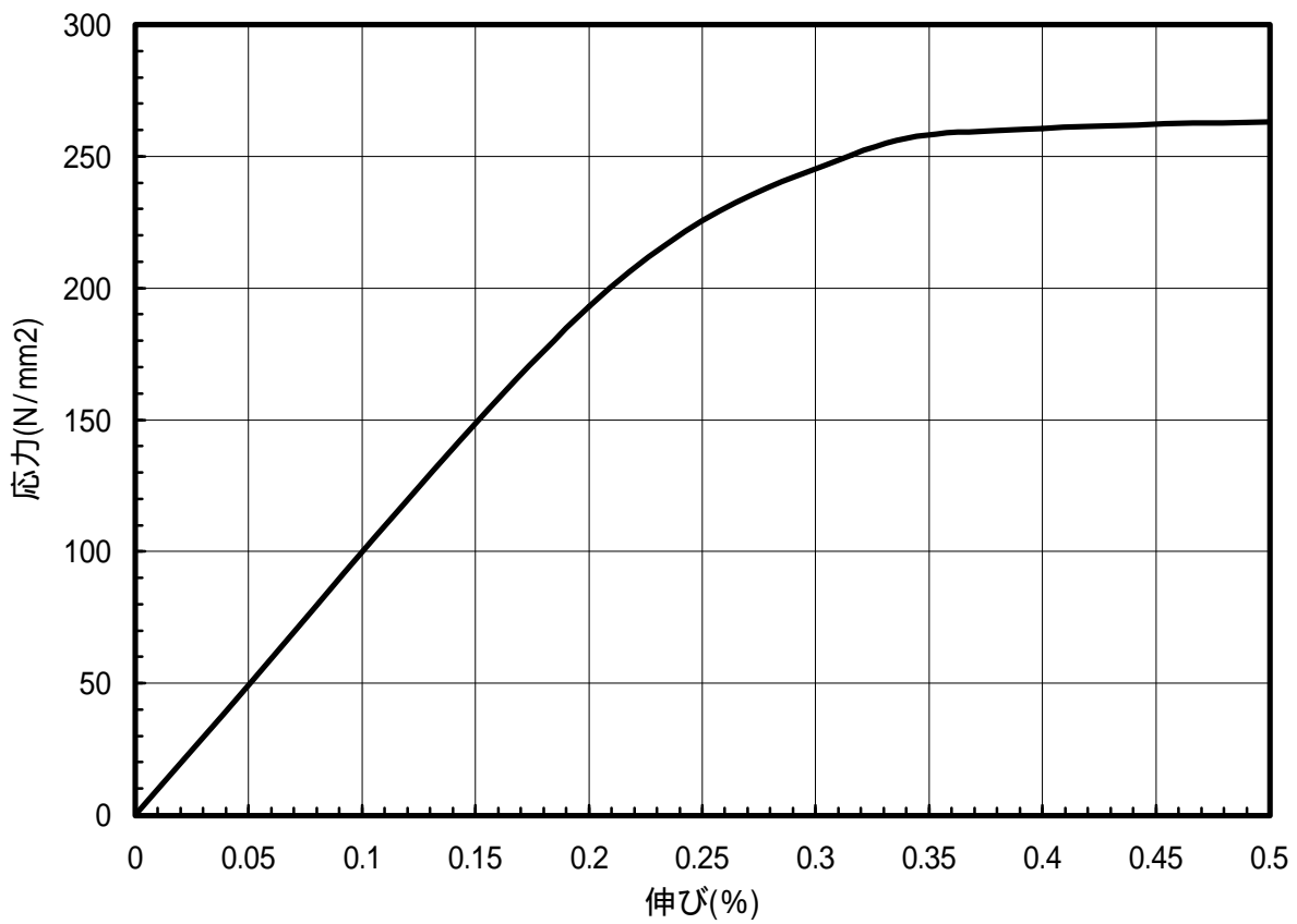
図 1.37 C2600-1/2H材のS-S曲線(T.D.)
