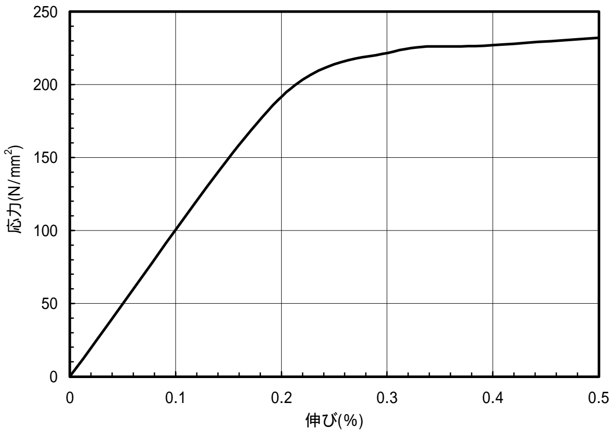
図 1.33 C2600-1/2H材のS-S曲線(L.D.)
