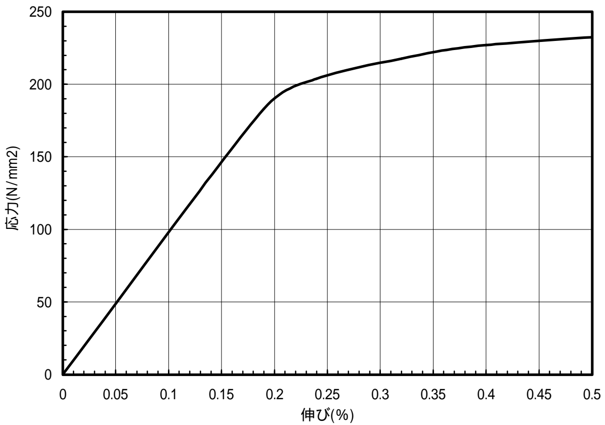
図 1.35 C2600-1/2H材のS-S曲線(45°)
