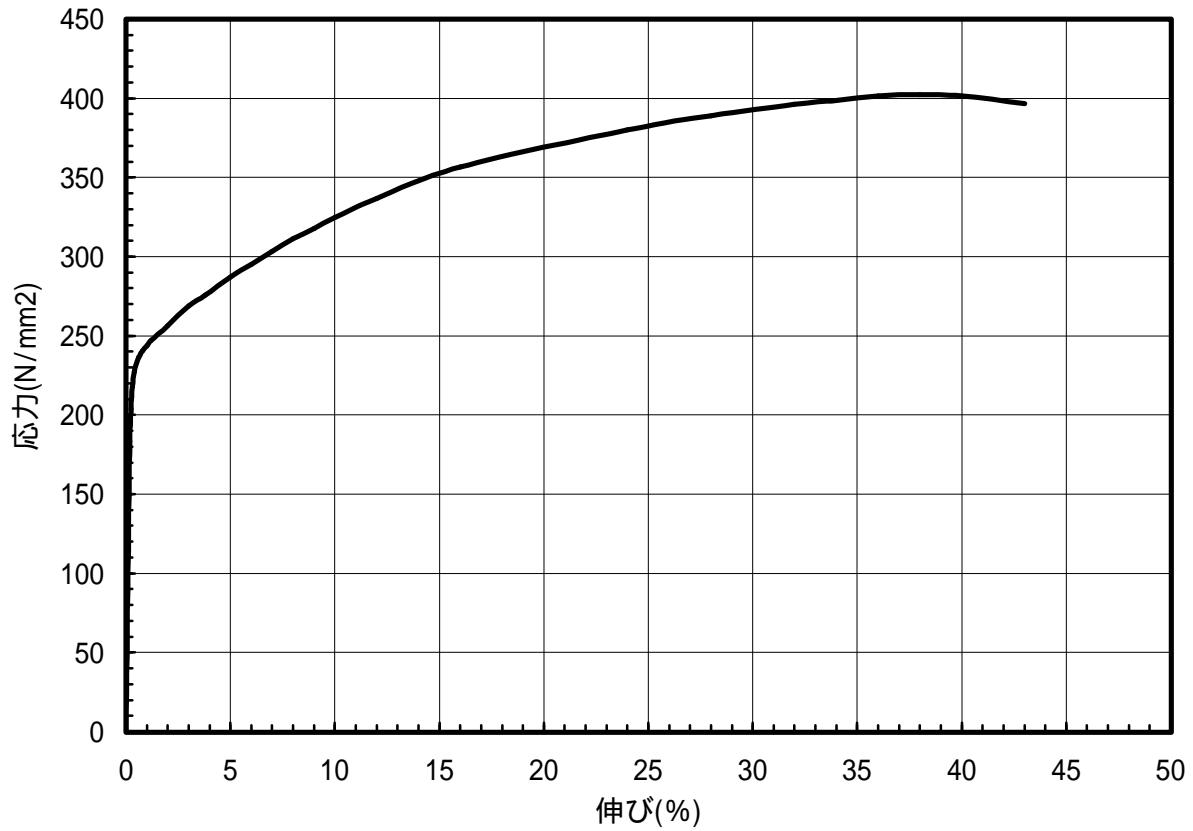
図 1.34 C2600-1/2H材のS-S曲線(45°)
