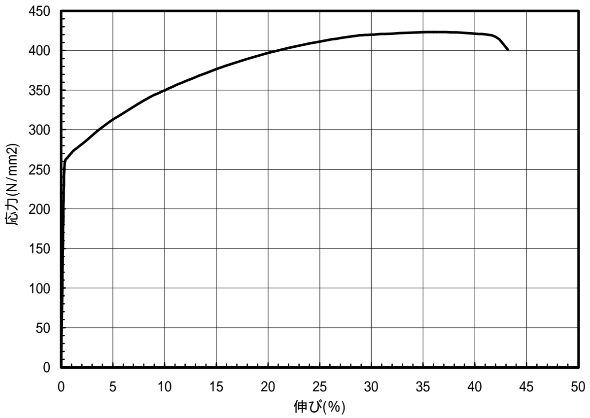
図 1.36 C2600-1/2H材のS-S曲線(T.D.)
