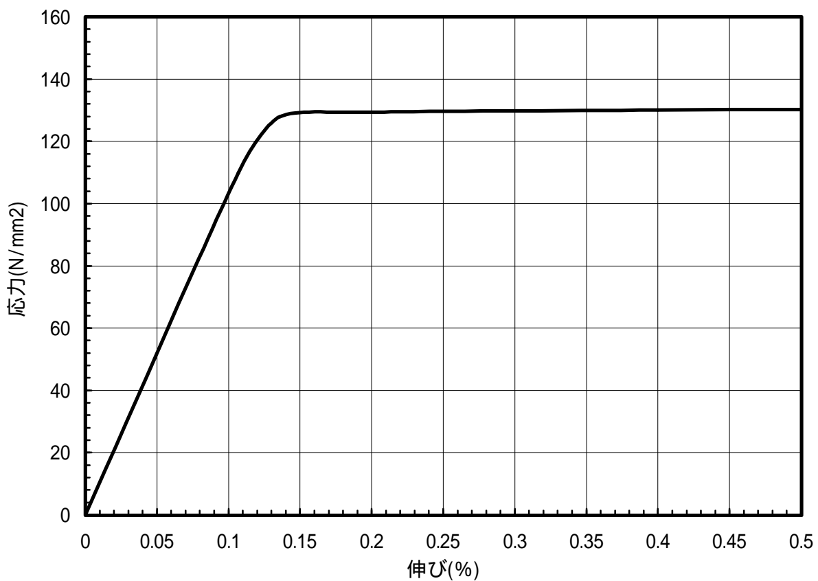
図 1.29 C2600-O材のS-S曲線(45°)
