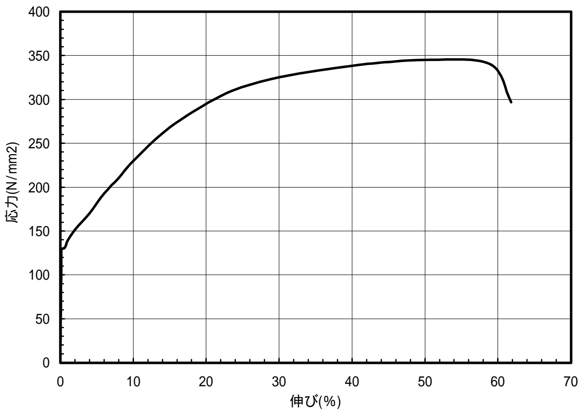
図 1.28 C2600-O材のS-S曲線(45°)
