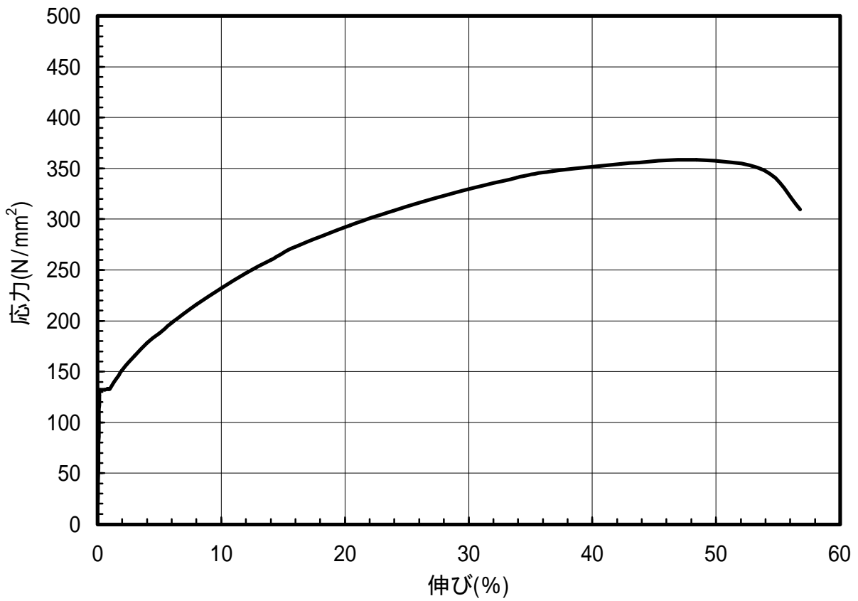
図 1.26 C2600-O材のS-S曲線(L.D.)
