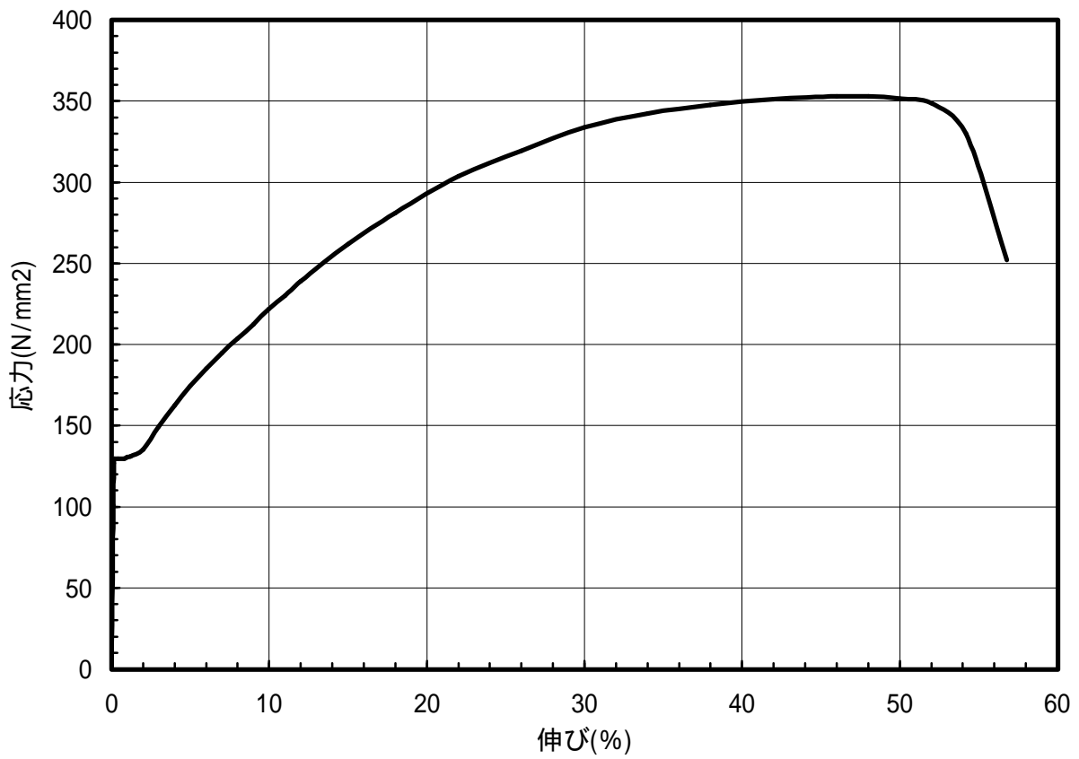
図 1.30 C2600-O材のS-S曲線(T.D.)
