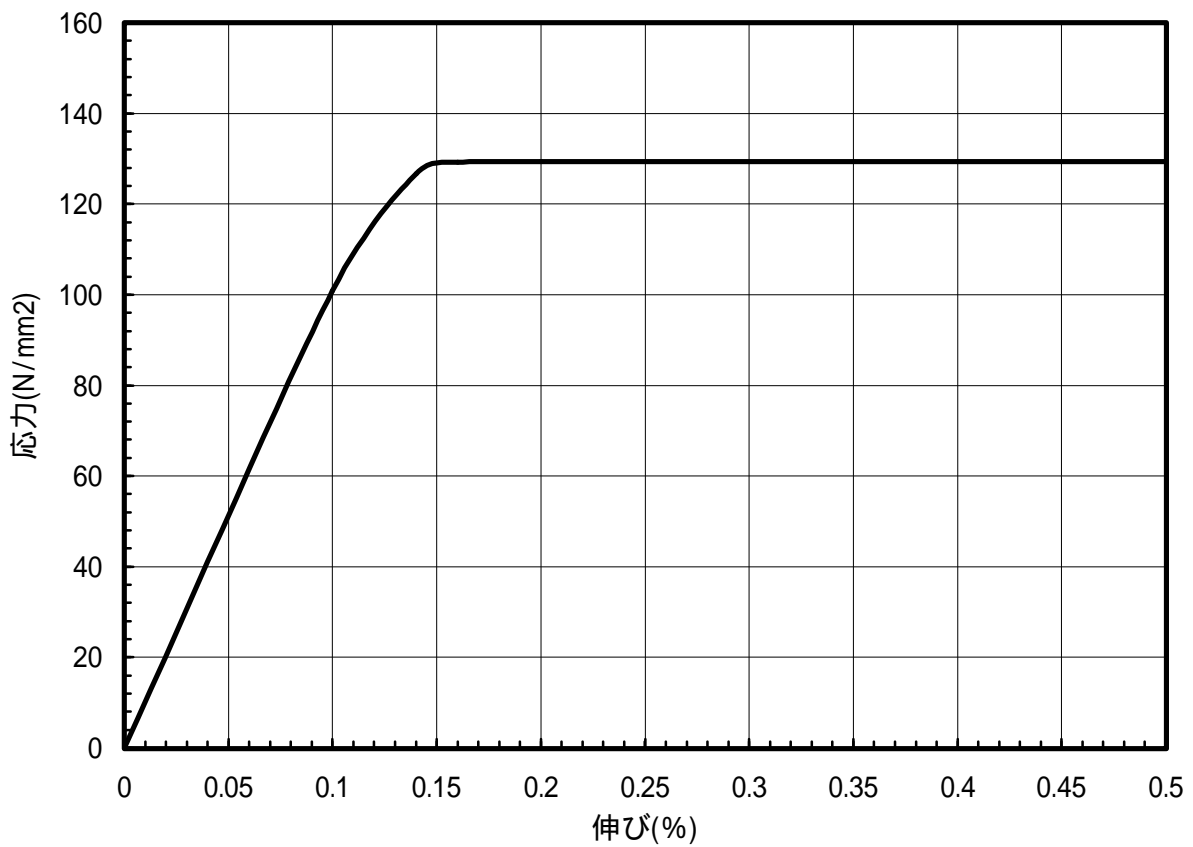
図 1.31 C2600-O材のS-S曲線(T.D.)
