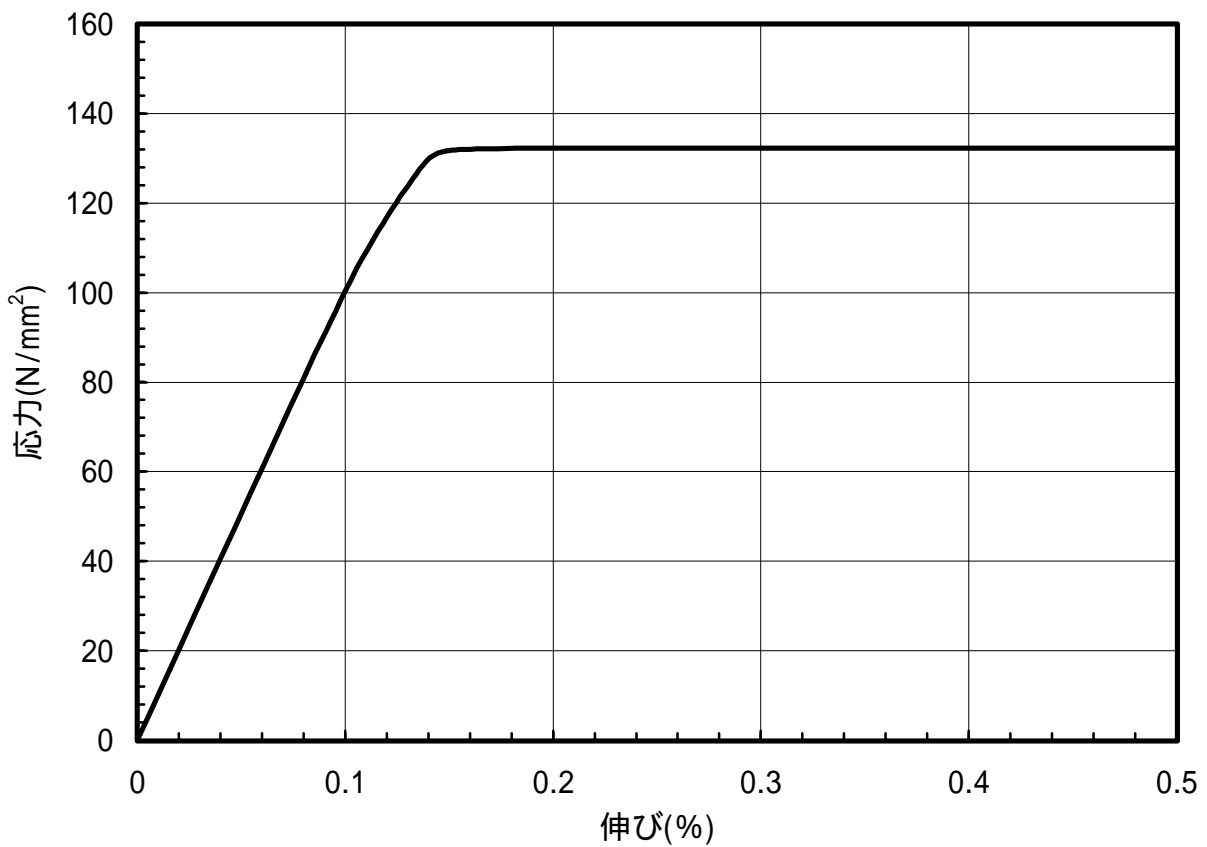
図 1.27 C2600-O材のS-S曲線(L.D.)
