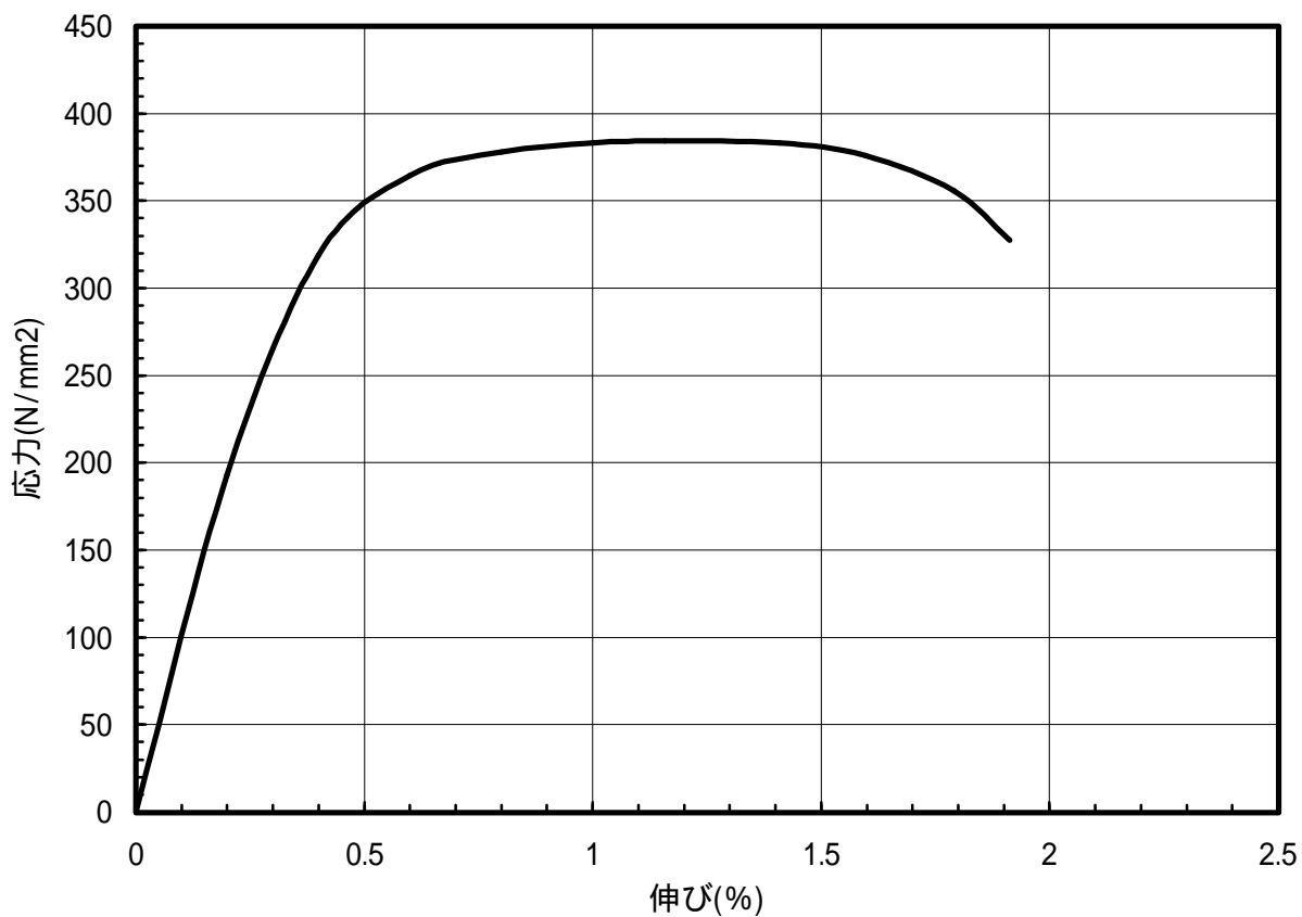
図 1.22 C1020-EH材のS-S曲線(45 °)
