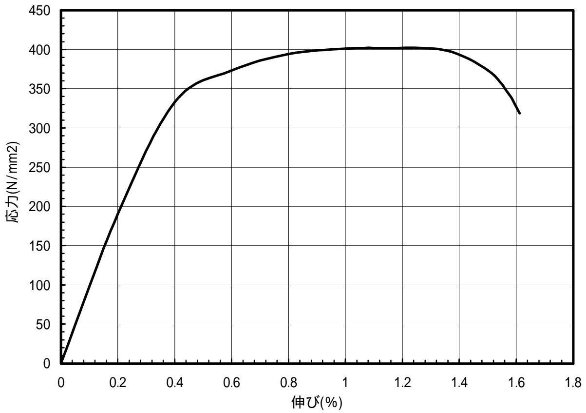
図 1.24 C1020-EH材のS-S曲線(T.D.)
