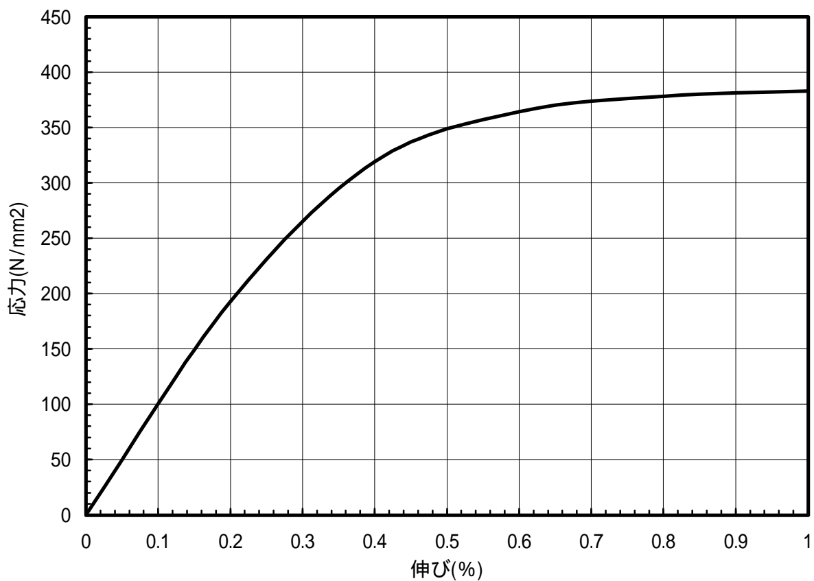
図 1.23 C1020-EH材のS-S曲線(45 °)
