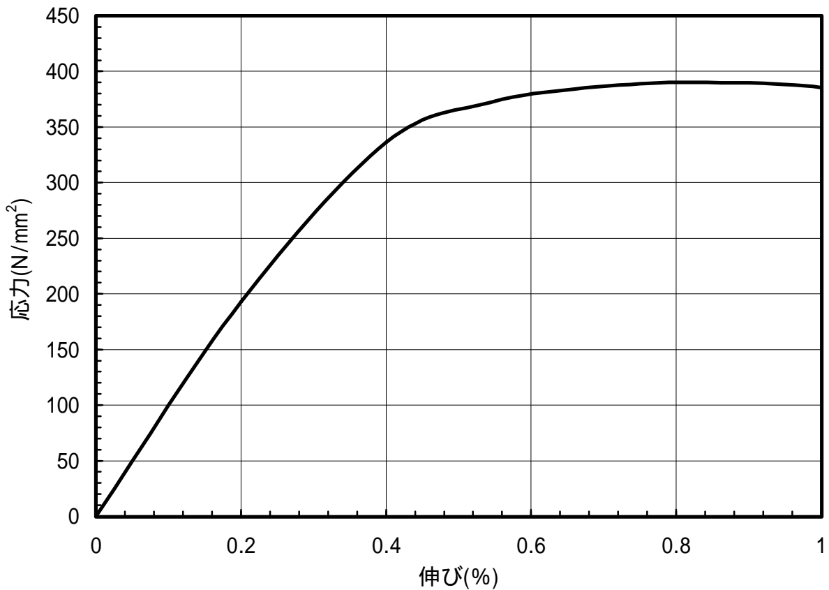
図 1.21 C1020-EH材のS-S曲線(L.D.)
