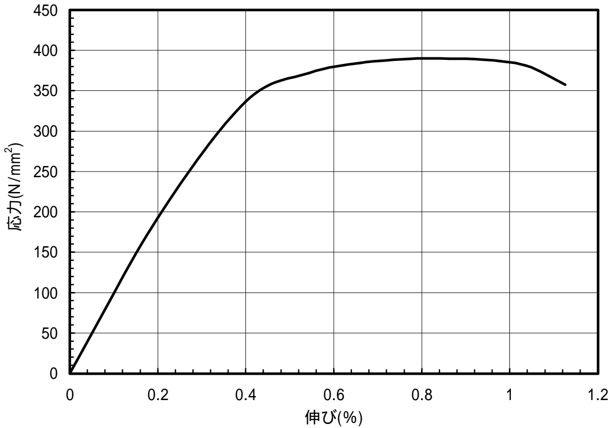
図 1.20 C1020-EH材のS-S曲線(L.D.)
