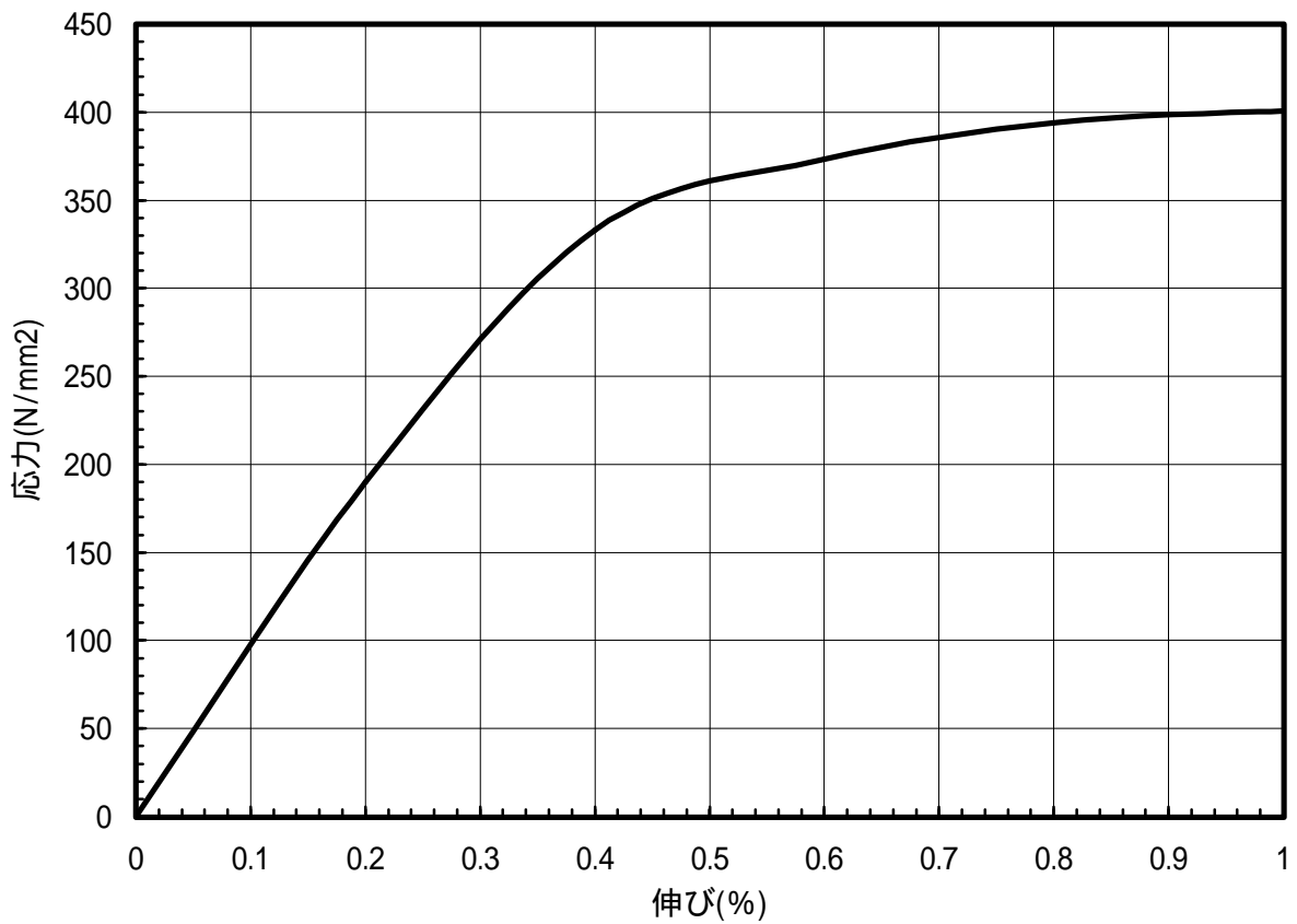
図 1.25 C1020-EH材のS-S曲線(T.D.)
