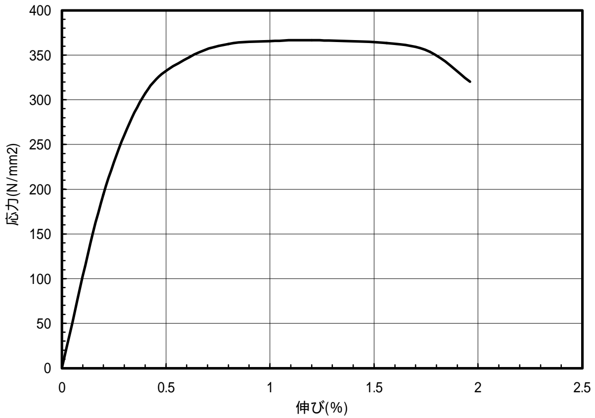
図 1.18 C1020-H材のS-S曲線(T.D.)
