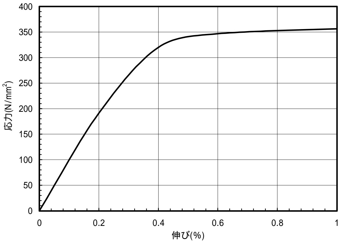
図 1.15 C1020-H材のS-S曲線(L.D.)
