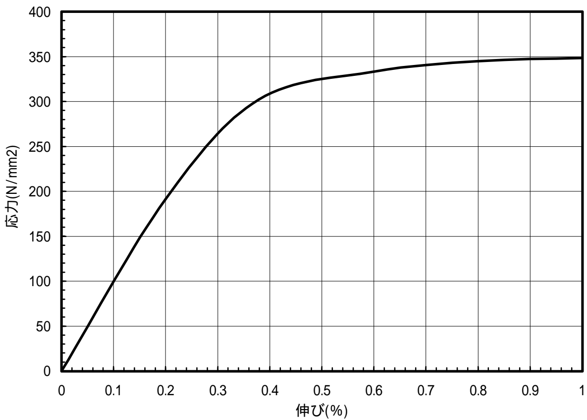
図 1.17 C1020-H材のS-S曲線(45 °)
