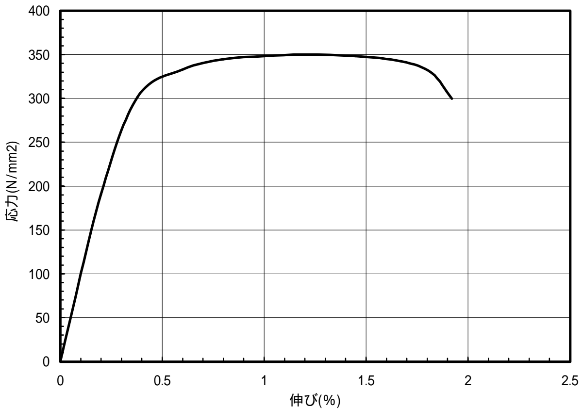
図 1.16 C1020-H材のS-S曲線(45 °)
