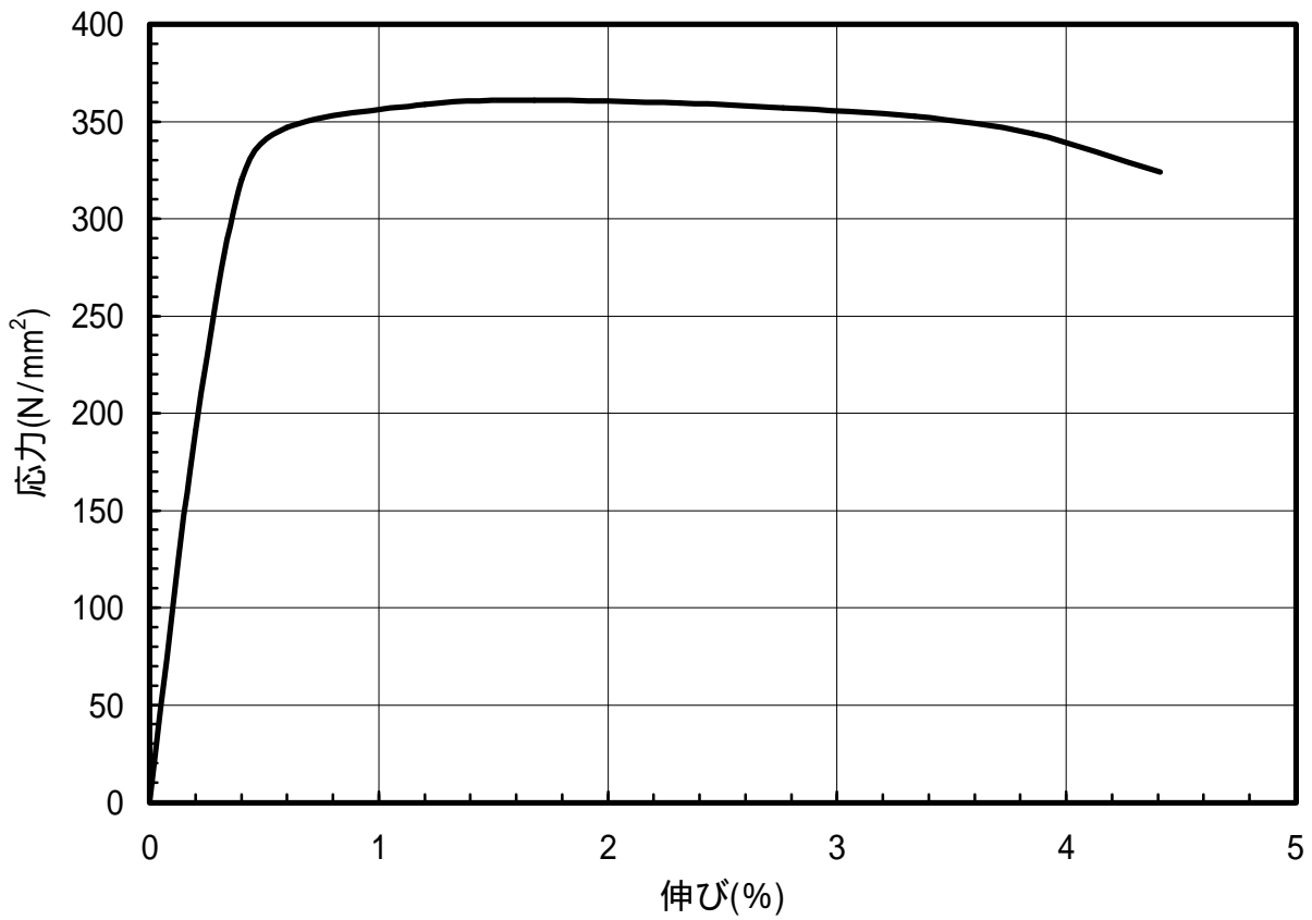
図 1.14 C1020-H材のS-S曲線(L.D.)
