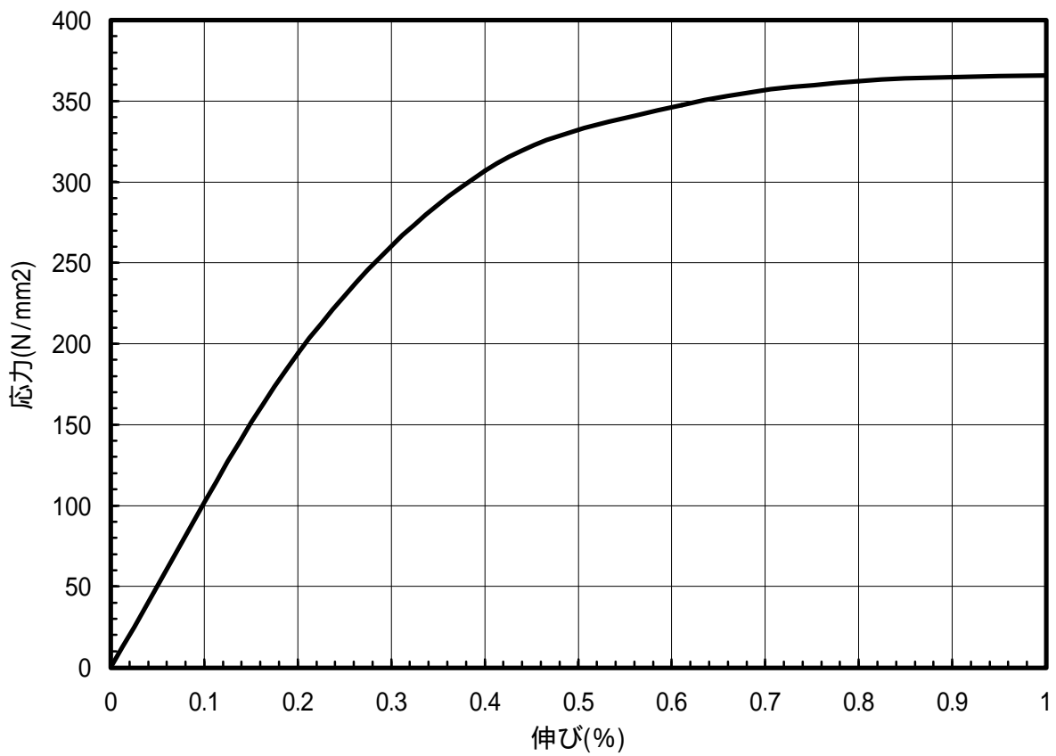
図 1.19 C1020-H材のS-S曲線(T.D.)
