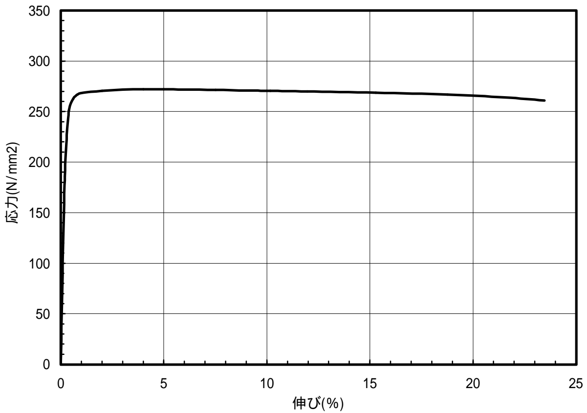
図 1.10 C1020-1/2H材のS-S曲線(45 °)
