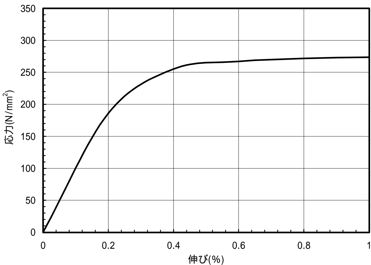
図 1.9 C1020-1/2H材のS-S曲線(L.D.)
