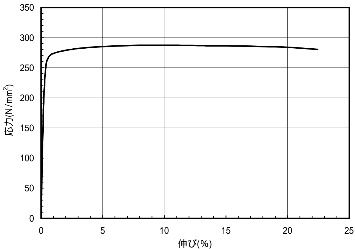
図 1.8 C1020-1/2H材のS-S曲線(L.D.)
