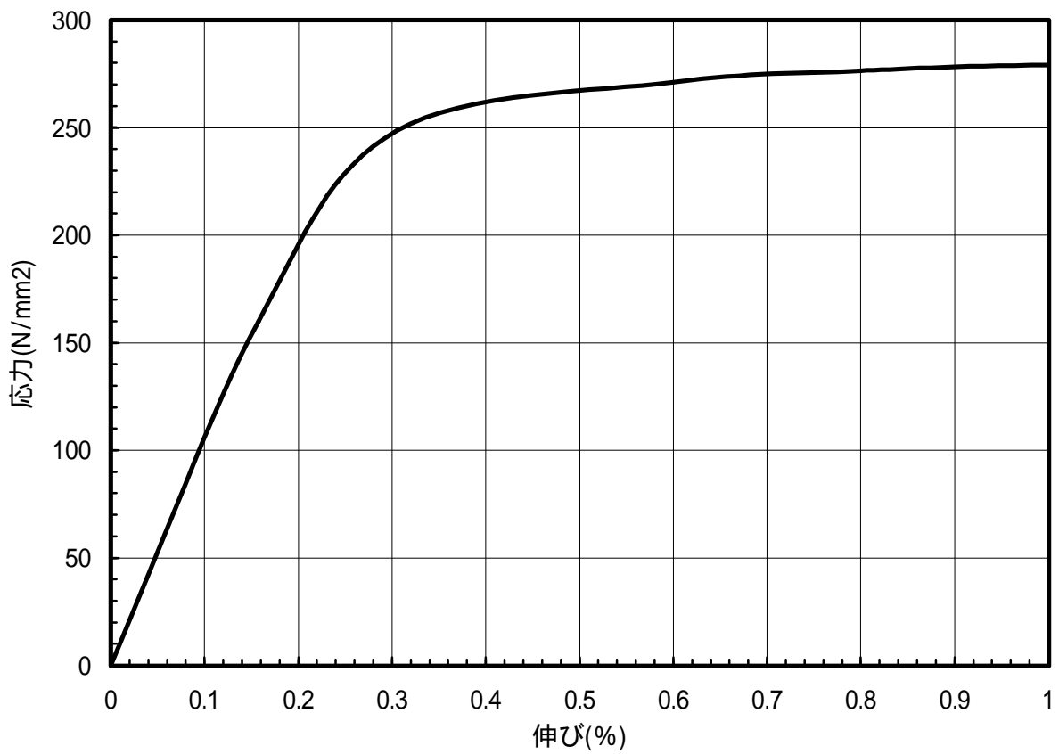
図 1.13 C1020-1/2H材のS-S曲線(T.D.)
