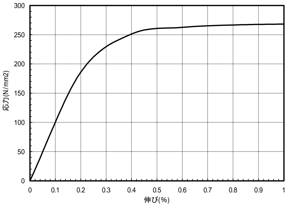
図 1.11 C1020-1/2H材のS-S曲線(45 °)
