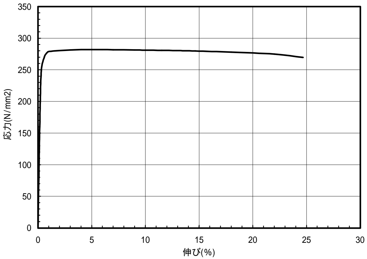
図 1.12 C1020-1/2H材のS-S曲線(T.D.)
