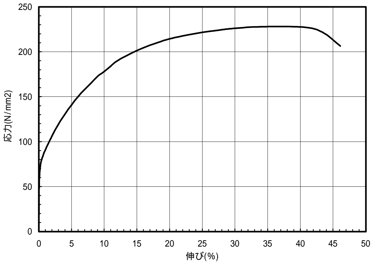
図 1.6 C1020-O材のS-S曲線(T.D.)
