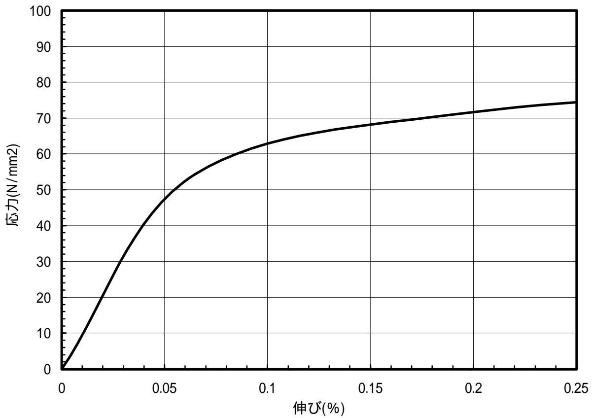
図 1.7 C1020-O材のS-S曲線(T.D.)
