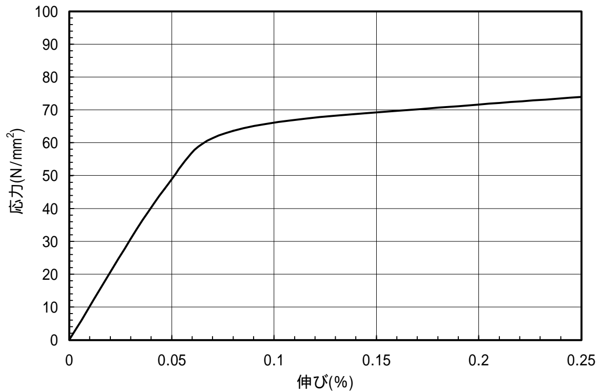
図 1.3 C1020-O材のS-S曲線(L.D.)
