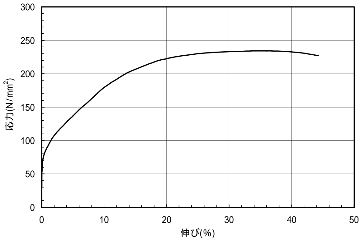
図 1.2 C1020-O材のS-S曲線(L.D.)
