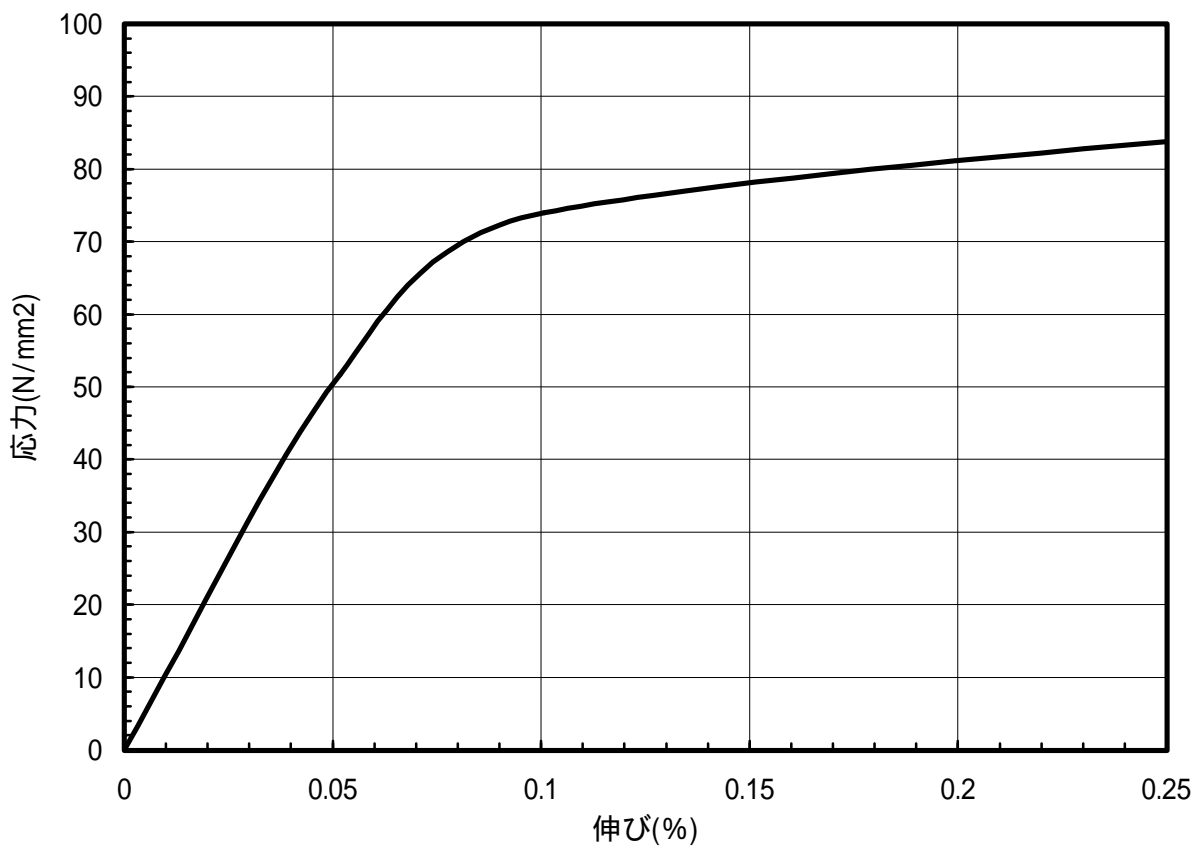
図 1.5 C1020-O材のS-S曲線(45°)
