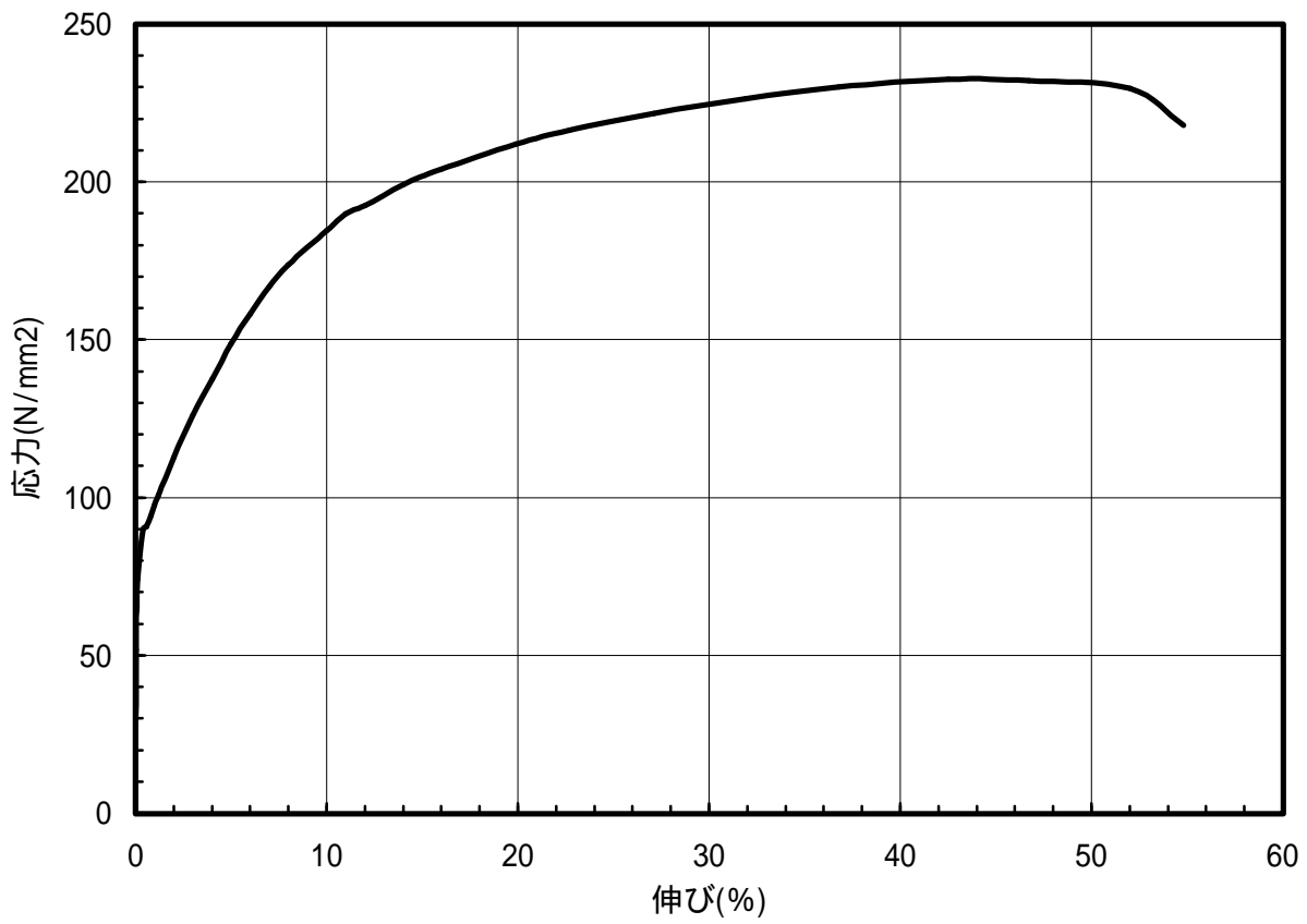
図 1.4 C1020-O材のS-S曲線(45°)
